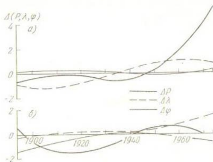
Рис. 19. Тренды третьего порядка отклонений параметров сезонных антициклонов от среднего многолетнего значения:
