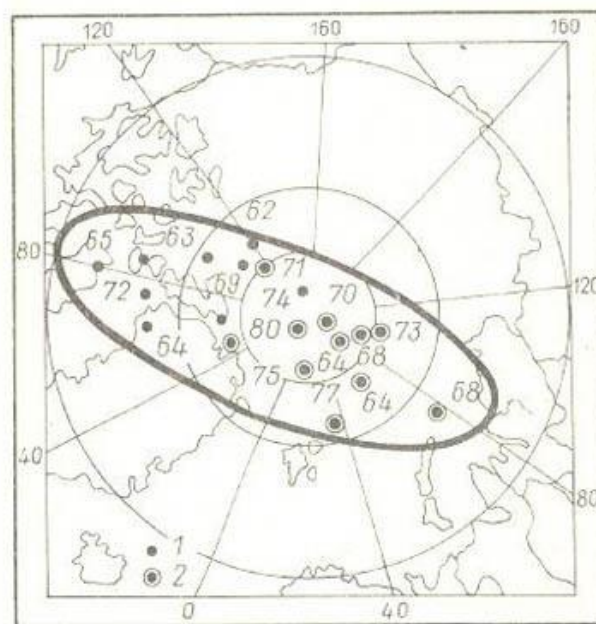
Рис. 16. Местоположение центра циркуляции на AT_{500} (среднее за май—август):
