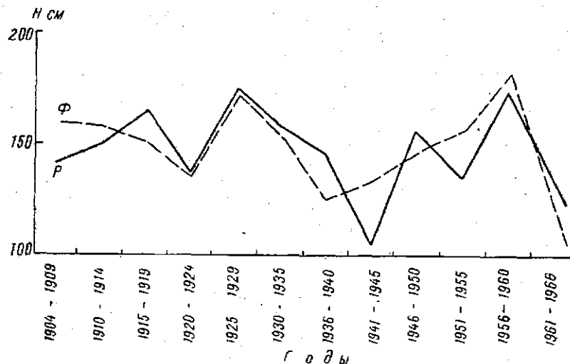
Рис. 2. Рассчитанные (P) и фактические (Ф) средние уровни Аральского моря по 5-6-летиям со сдвигом на один год
