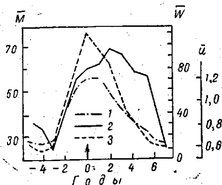
Рис. 1. Средние циклические кривые (за 1884—1966 гг.):
