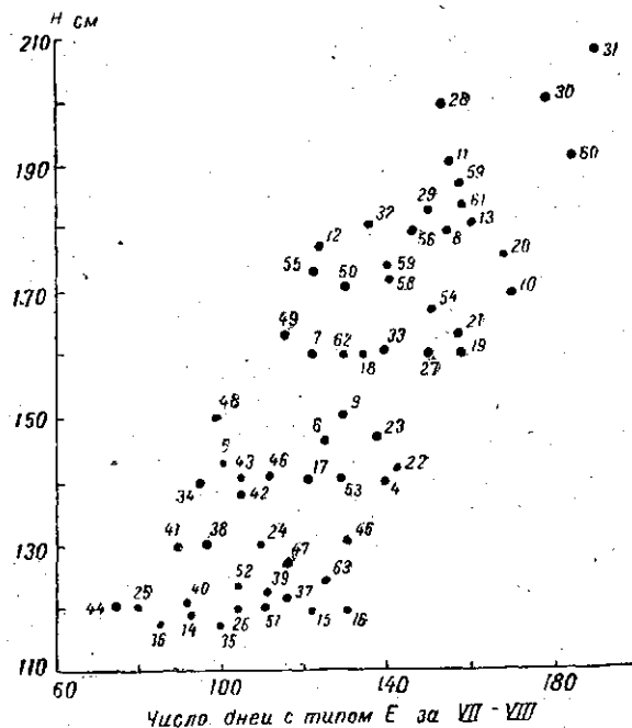
Рис. 1. Связь между уровнем Аральского моря и числом дней за июль—август с типом Е атмосферной циркуляции (1904—1963 гг.)
