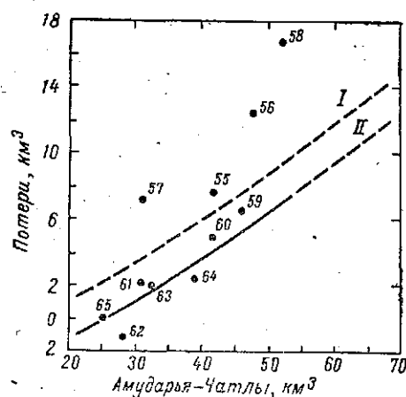
Рис. 2. Связь потерь стока в дельте Амударьи и ее стока у кишла. Чатлы за период 1955—65 гг.:
