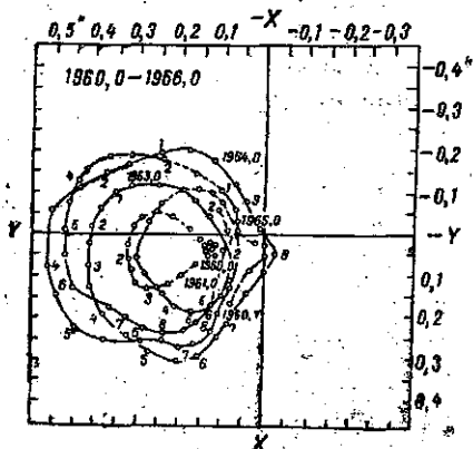
Рис. 1в. Траектория мгновенного полюса вращения Земли
