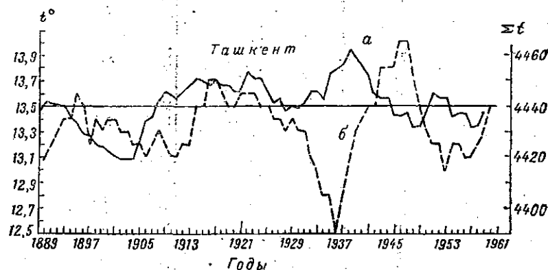
Рис. 4. Сопоставление средних годовых скользящих по 10-летиям температур воздуха и сумм температур \geq 10^\circ : а — средние годовые, б — сумма \geq 10^\circ
