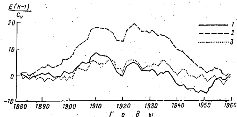
Рис. 1. Интегральные кривые \frac{\sum (K-1)}{C_v} годового стока:
