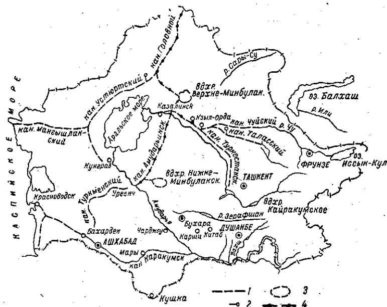
Рис. 1. Схематическая карта бассейна Аральского моря. Предварительная основа водохозяйственных мероприятий: 1 — водопроводящие тракты, 2 — насосные станции, 3 — водохранилища, 4 — первая очередь работ по переробу стока сибирских рек, 5 — граница бассейна
