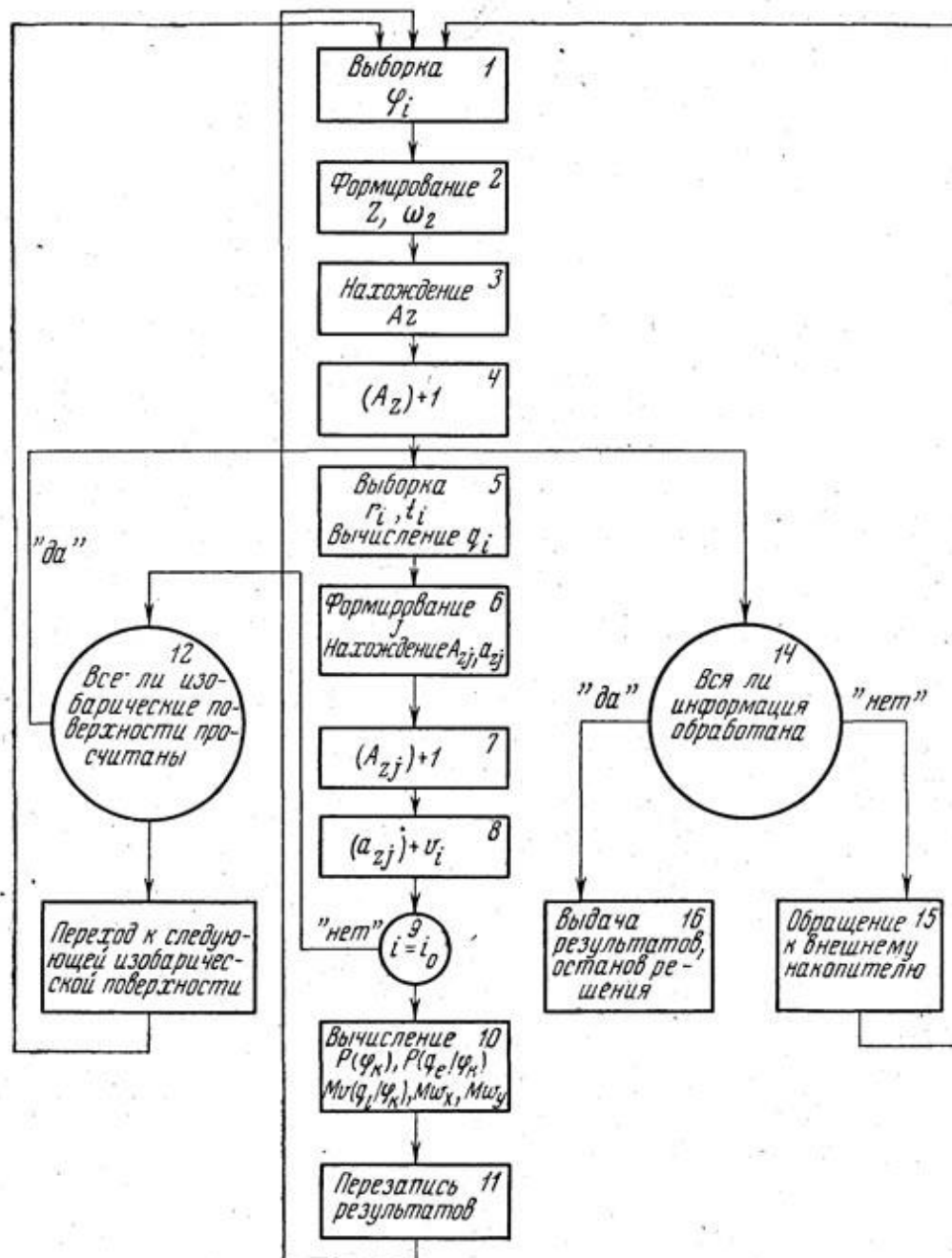
Рис. Блок-схема программы
