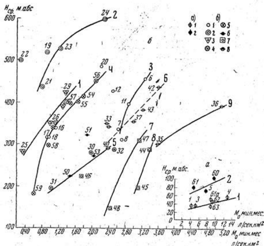
Рис. 2. Кривые зависимости минимального месячного зимнего стока от средней высоты водосбора: а — реки Северо-Сахалинской низменности; б — реки Центрального и Южного Сахалина. Прямыми цифрами (5) показаны кривые зависимостей, соответствующие номерам районов; наклонными (15) — номера гидрологических створов. Условные обозначения (1—9) см. в тексте статьи
