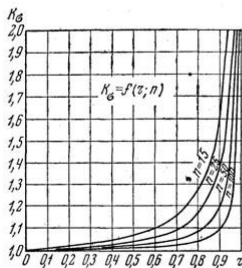
Рис. 4. График зависимости теоретической поправки на связность ряда для стандартной ошибки K_{\sigma} = f(r, n)
