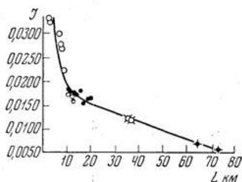
Рис. 1. Связь уклонов рек с их длиной
