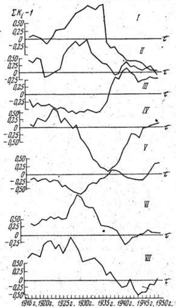
Рис. 2. Интегральные кривые суммарного стока по гидрологическим районам. Римскими цифрами показаны гидрологические районы
