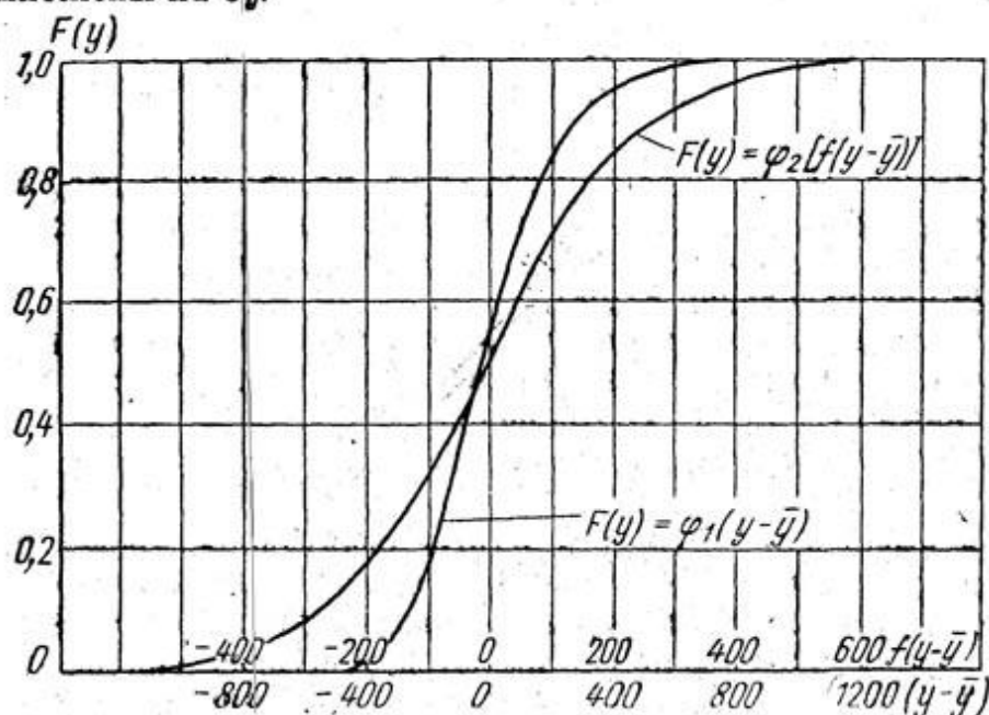
Рис. 1. График зависимости F(y) = \Phi_1(y - \bar{y}) и F(y) = \Phi_2[f(y - \bar{y})]
