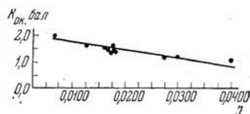
Рис. 2. Связь уклонов рек с окатанностью галечников
