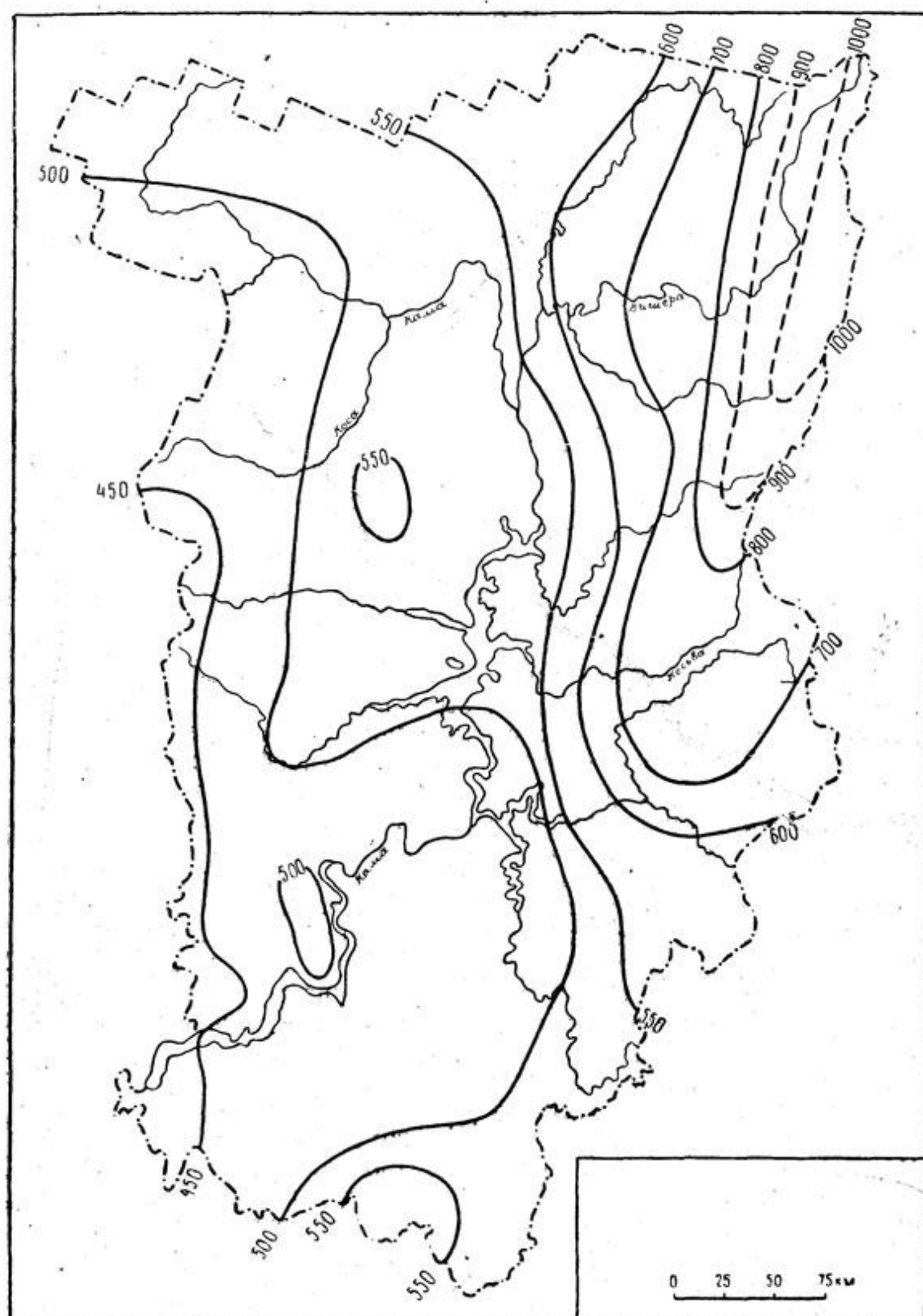
Рис. 1. Средние годовые суммы атмосферных осадков
