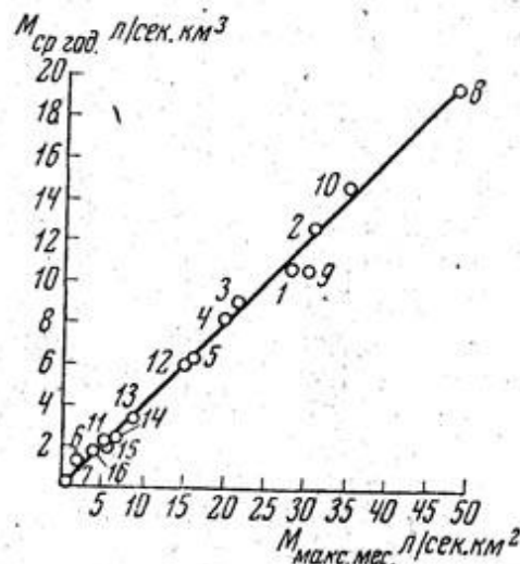
Рис. 3. Связь максимального месячного стока рек Ирака со средним годовым стоком. Цифры у точек — см. табл. 1, 2
