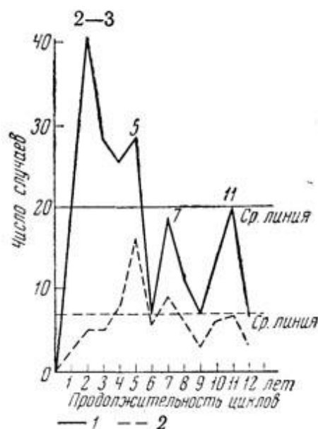
Рис. 3. Повторяемость циклов различной продолжительности: 1 — характерные значения (из 205 случаев); 2 — максимальные значения (из 72 случаев)
