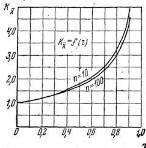
Рис. 2. Зависимость поправки на связность к стандартной ошибке среднего ( \bar{x} ) от коэффициента корреляции
