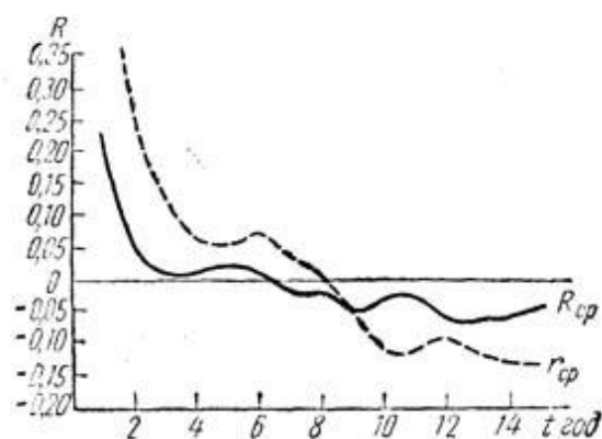
Рис. 1. Суммарные автокорреляционные функции. Кривые колебаний средних коэффициентов: R_{cp} — по 72 бассейнам, r_{cp} — только по зарегулированным бассейнам
