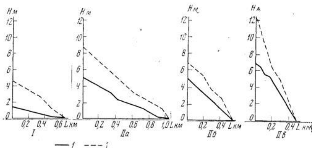
Рис. Типовые продольные профили русел рек Абхазии: I — полугорные русла; II — горные, с развитыми русловыми формами; IIб — горные, с неразвитыми русловыми формами; IIв — порожиисто-водопадные русла. 1 — русла рек с площадью бассейна более 100 км², 2 — русла рек с площадью бассейна более 10—100 км²
