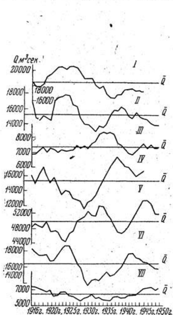
Рис. 1. Колебания суммарных средних годовых расходов воды по гидрологическим районам. Римскими цифрами показаны гидрологические районы
