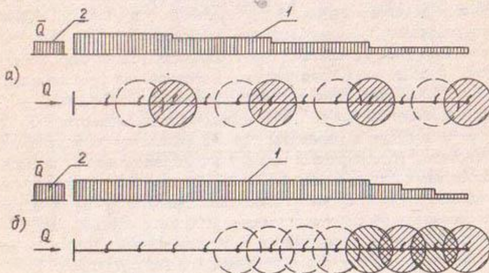
Рис. I. Варианты водооборотов на единичном водоводе: а) – равномерная и б) – сосредоточенная по длине водовода работа поливных устройств; 1 – эпюра линейного расхода водовода; 2 – средневзвешенная пропускная способность водовода
