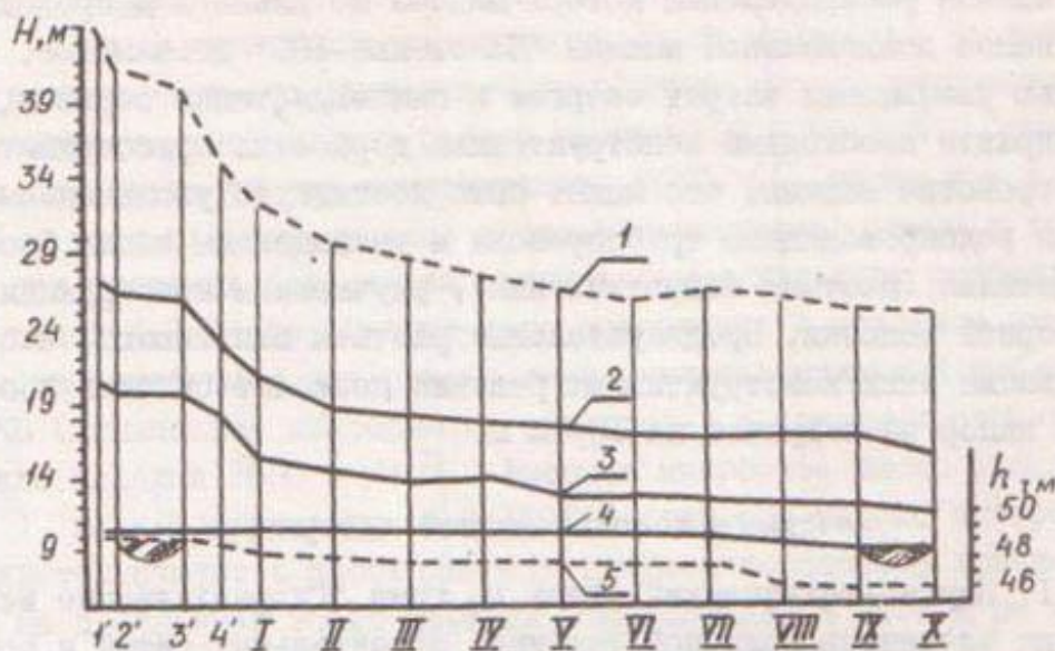
Рис.5. Распределение напора H (1, 2, 3) и отметок поверхности земли h_2 (4, 5) по длине водопроводящего пояса ДМ "Коломенка-100"
