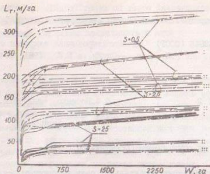
Рис.7. Удельный расход управляющей трубки для многоканальной схемы дистанционного управления группой запорных органов с гидроприводом: — при соотношении сторон 1:1; — при соотношении сторон 1:2; —v— при соотношении сторон 1:5; —. —. — при соотношении сторон 1:10
