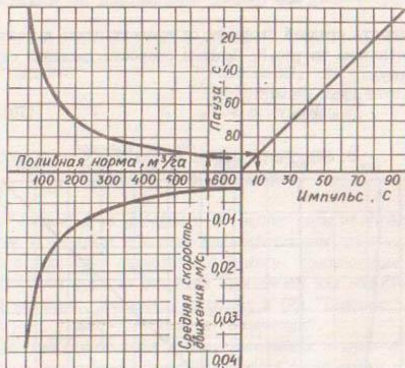
Рис. I. Номограмма для определения параметров движения ЭДМФ "Кубань"
