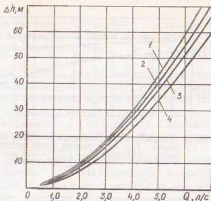
Рис.3. Зависимость потерь напора (на 100 м) от расхода для полиэтиленового шланга d_{\text{ш}} = 39,2 мм с разными диаметрами навивки: 1 - d_n = 1 м; 2 - d_n = 1,5 м; 3 - d_n = 2 м; 4 - гладкий участок
