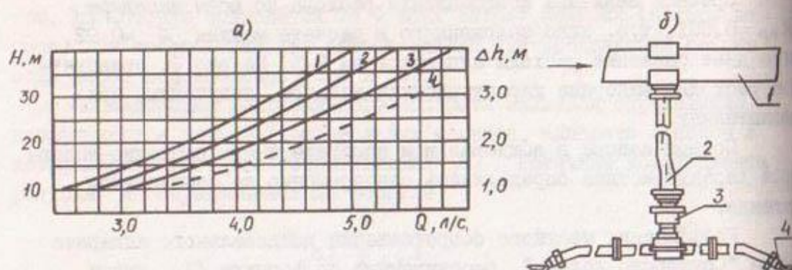
Рис. 4. Дождевальный аппарат типа "Сегнерово колесо" ДМ "Коломенка-100": а) зависимость Q = f(H) : 1 - d = 11,5 \text{ мм} , 2 - d = 12,0 \text{ мм} , 3 - d = 12,5 \text{ мм} ; 4 - зависимость \Delta h = f(Q) ; б) - основные узлы: 1 - трубопровод; 2 - резиновотканевый рукав; 3 - поворотный механизм; 4 - насадка
