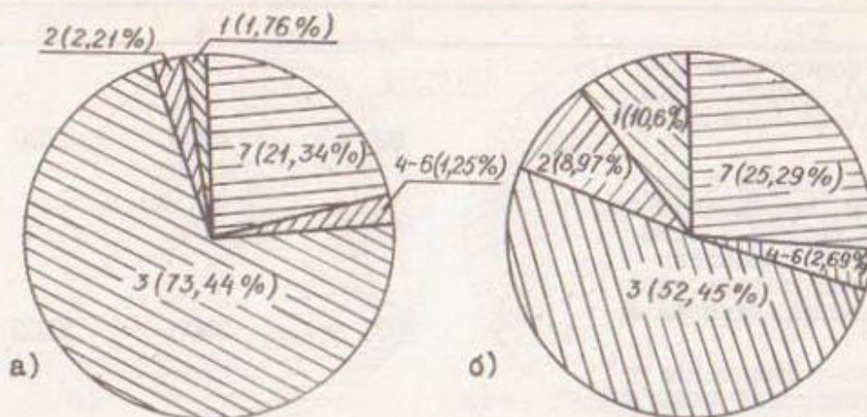
Рис.2. Распределение узлов и деталей ДМ "Фрегат" в зависимости от их ресурса: а) и б) – соответственно по массе и стоимости; 1...7 – обозначения соответствующих групп таблицы 2
