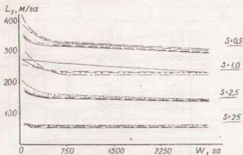
Рис.5. Удельный расход управляющей трубки при комбинированной (многоканальная и матричная) схеме дистанционного управления запорными органами с гидроприводом: — при соотношении сторон 1:1; --- при соотношении сторон 1:2; -·-·- при соотношении сторон 1:5; - - - - при соотношении сторон 1:10
