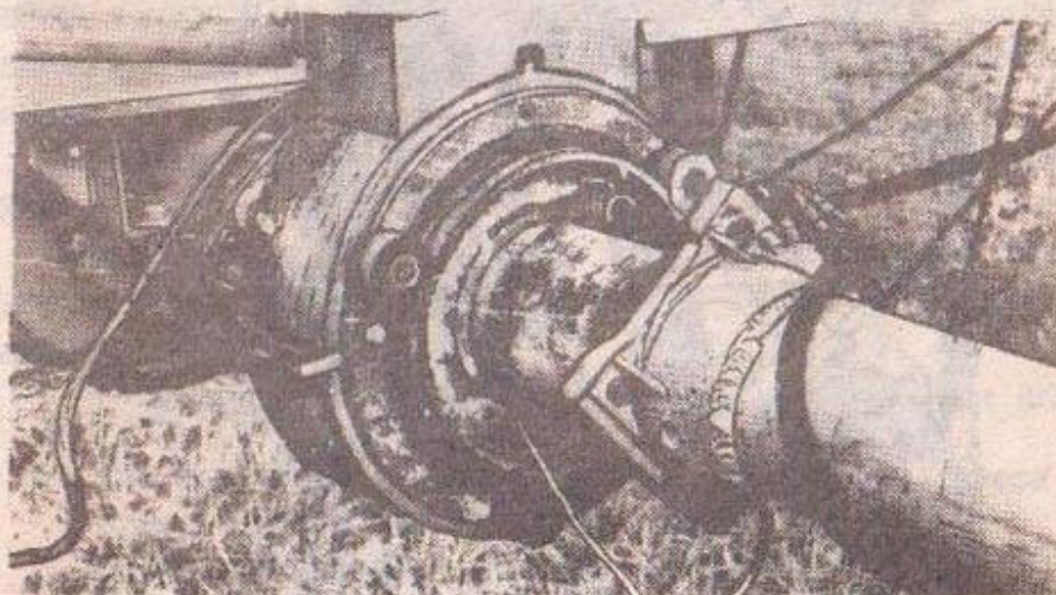
Рис. I. Токосъемник у приводной тележки
