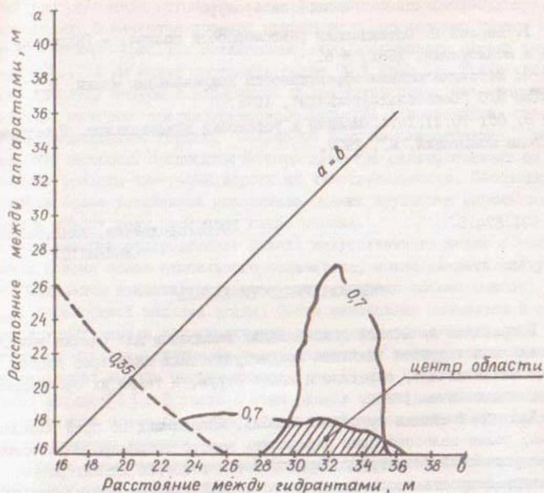
Рис.3. Область оптимальных расстановок дождевальных аппаратов на КДТ
