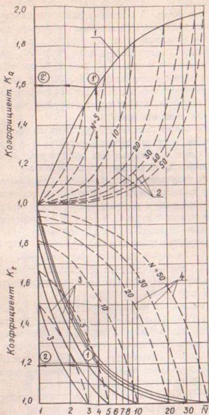
Рис.2. Номограмма для определения коэффициентов K_q и K_t единичного водовода: 1, 3 – соответственно значения K_q и K_t по уравнениям (14); 2, 4 – соответственно значения K_q и K_t по уравнениям (15)
