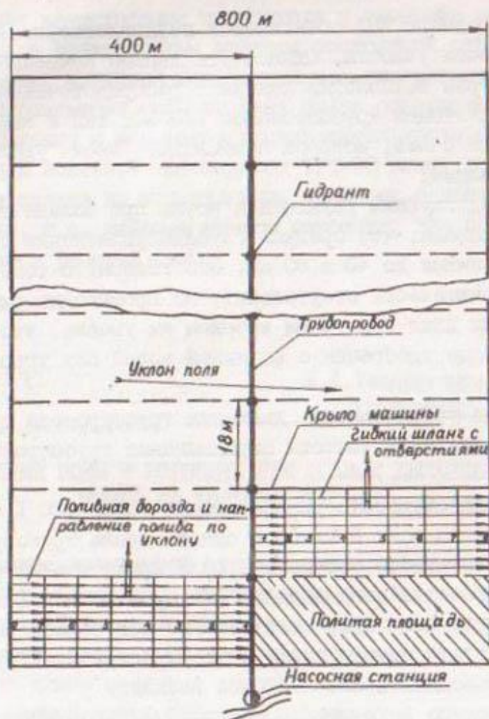
Рис.3. Схема полива
