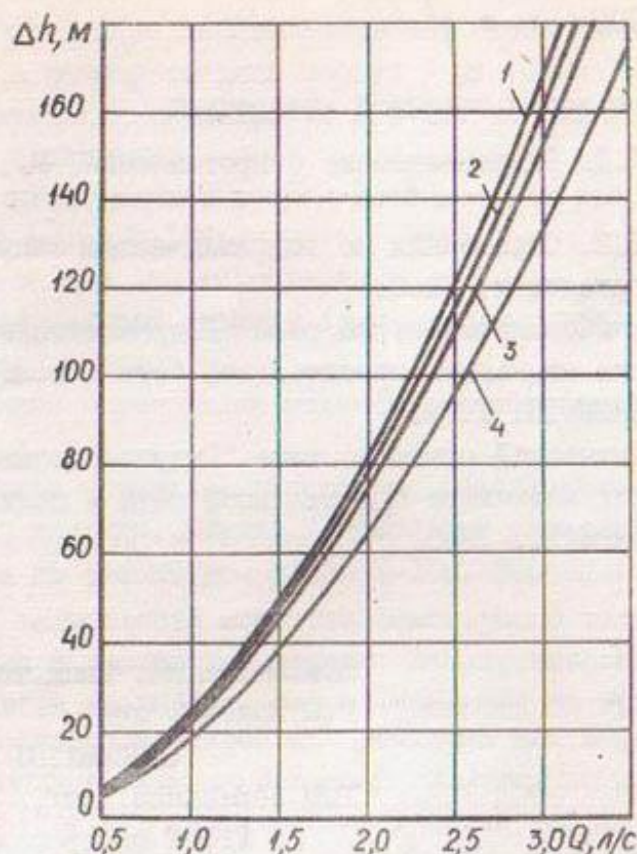
Рис. 4. Зависимость потерь напора (на 100 м) от расхода для полиэтиленового шланга d_{\text{ш}} = 24,5 мм с разными диаметрами навивки: 1 - d_n = 1 м; 2 - d_n = 1,5 м; 3 - d_n = 2 м; 4 - гладкий участок
