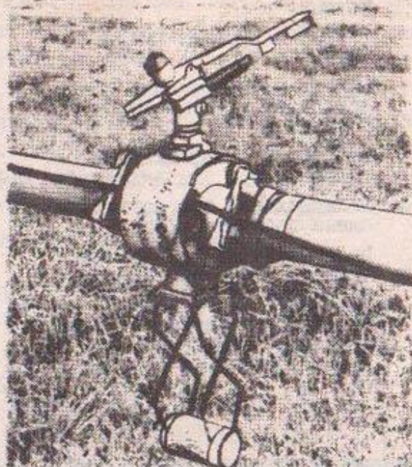
Рис.3. Механизм самоустановки дождевального аппарата
