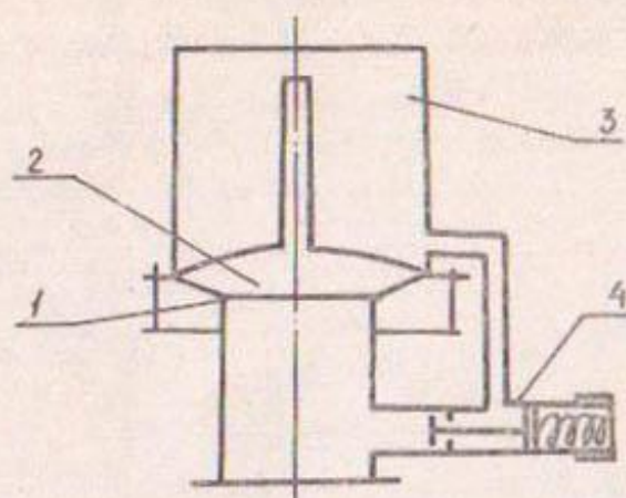
Рис. I. Схема противоударного устройства: I - диафрагма; 2 - водовоздушный бак; 3 - корпус; 4 - отсечный клапан
