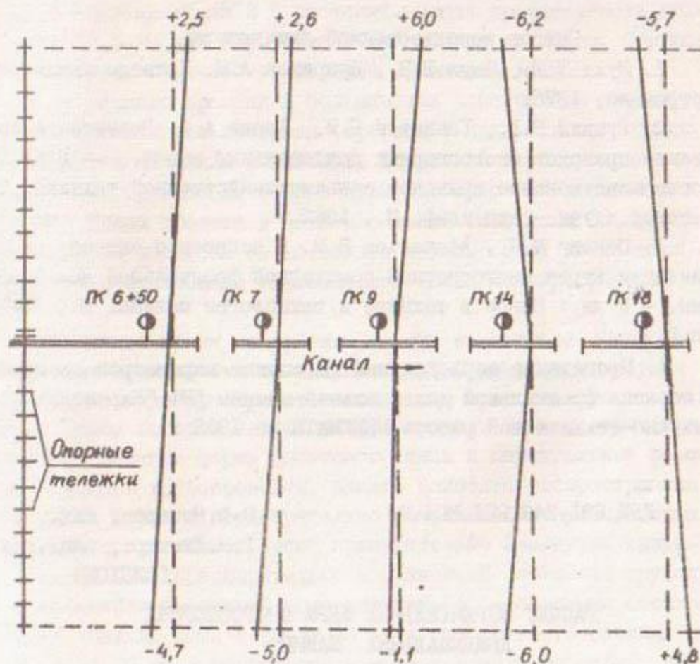
Рис.3. характер перемещения ДМФ "Каравелла"
