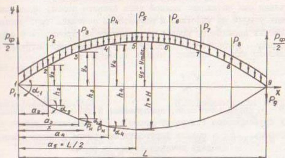
Рис.2. Расчетная схема фермы
