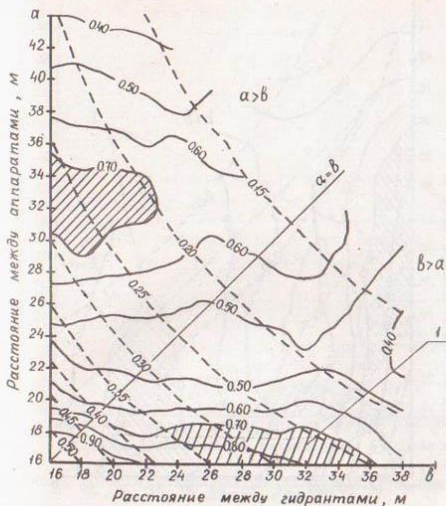
Рис. I. Зависимость средней интенсивности и коэффициента эффективного полива от расстояний между аппаратами и гидрантами: I - область оптимальной расстановки аппаратов; аппарат "Роса-3", H = 35 м; Q = 45 л/с; направление ветра перпендикулярно к оси трубопровода V_{ср} = 2,4 м/с; — — — — — K_{эп} ; - - - - - \rho_{ср}
