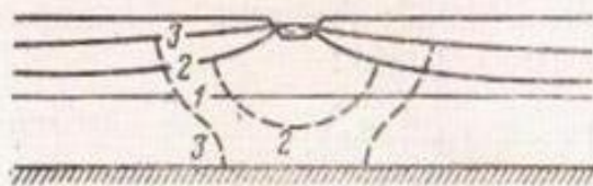
Рис. 56. Схема к расчету перемещения зоны опреснения вблизи канала в условиях не установившегося движения;
