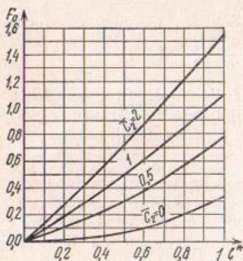
Рис. 36. График для расчета интерференции скважины.
