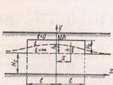
Рис. 17. Схема растекания бугра грунтовых вод.
