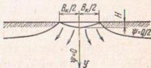
Рис. 48. Схема к расчету фильтрации из одиночного канала.
