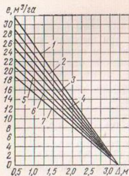
Рис. 19. Расход грунтовых вод на испарение и транспирацию хлопчатника:
