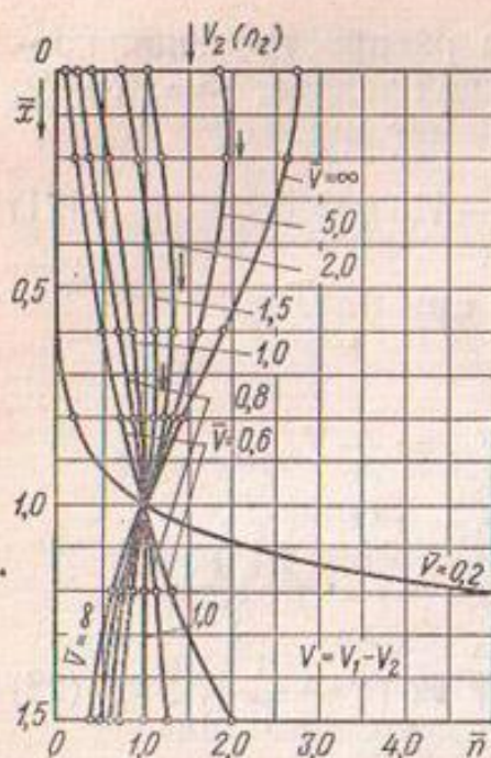
Рис. 7. Зависимость распределения солей в почве от соотношения скоростей вертикального водообмена \bar{V} с учетом расходования воды корнями растений при V = V_1 \bar{x} - V_2 , Re=1 , n_2=0 , \bar{V} = V_1/V_2 , \bar{n} = n/n_1 .
