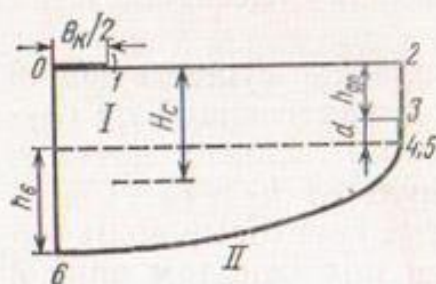
Рис. 55. Схема к расчету предельной глубины опреснения:
