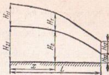
Рис. 46. Схема к расчету по формулам Н. К. Гириного.
