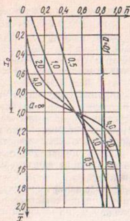
Рис. 10. Схема к расчету коэффициента конвективной диффузии.
