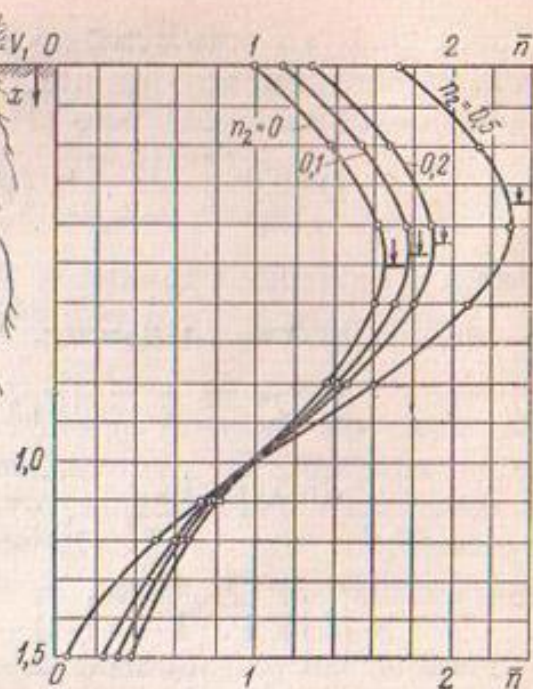
Рис. 8. Влияние минерализации поливных вод на засоление почв (для схемы рис. 7) при Re=2 , \bar{V}=2 .
