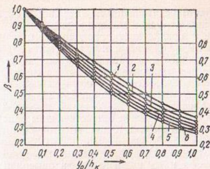
Рис. 39. График для определения расхода капиллярной зоны:
