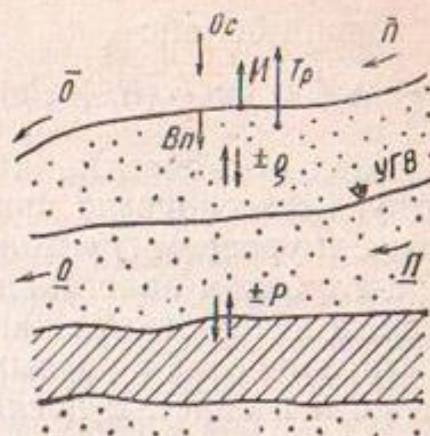
Рис. 1. Схема составляющих водного баланса:
