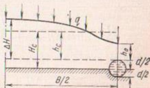
Рис. 24. Схема к расчету горизонтального дренажа при наличии инфильтрации (залегание дрен на водоупоре).
