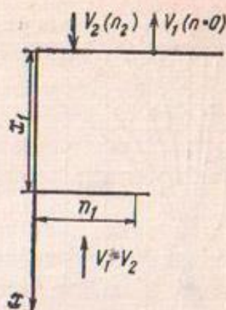
Рис. 2. Схема к расчету передвижения солей в почвенном слое.
