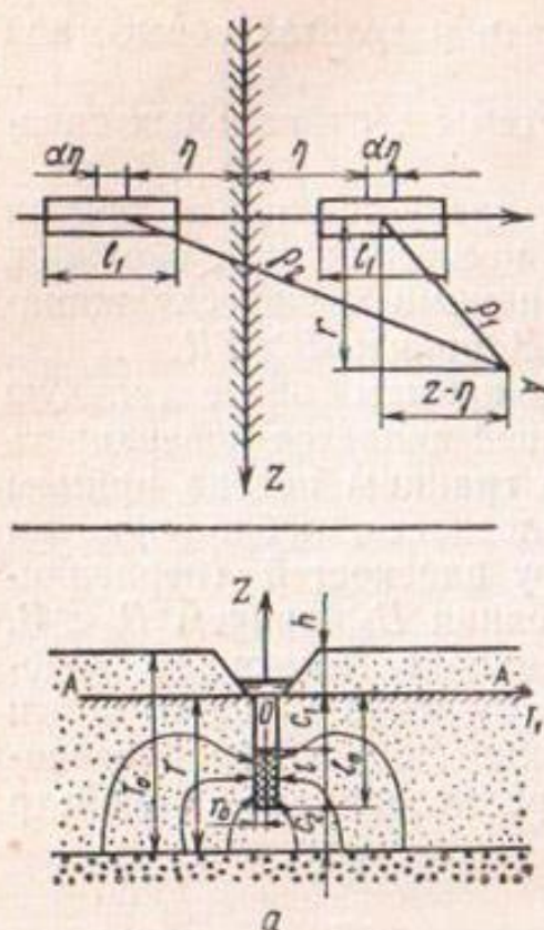
Рис. 33. Схема к расчету притока к одиночной скважине: 1 — сток; 2 — источник.
