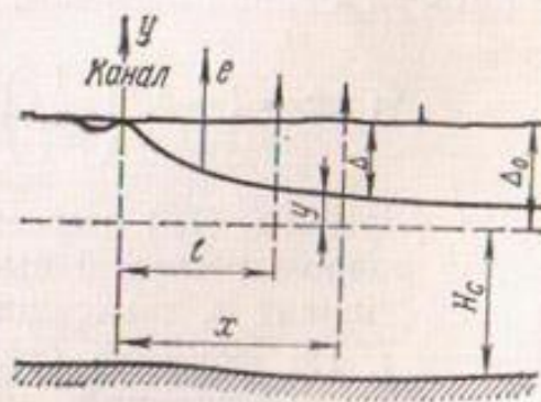
Рис. 18. Схема к расчету подпорной фильтрации из канала.
