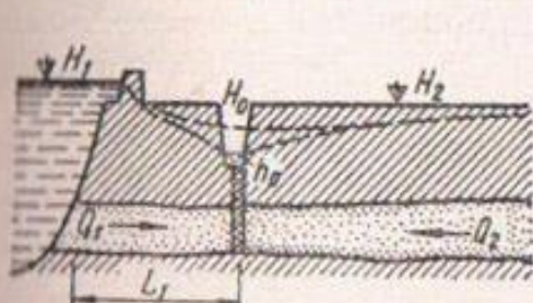
Рис. 43. Схема к расчету берегового дренажа.
