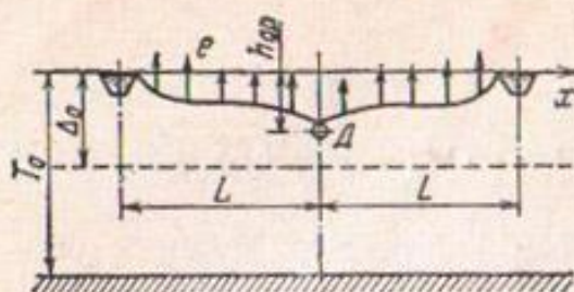
Рис. 51. Схема к расчету фильтрации из системы каналов при наличии дренажа и испарения с поверхности грунтовых вод.
