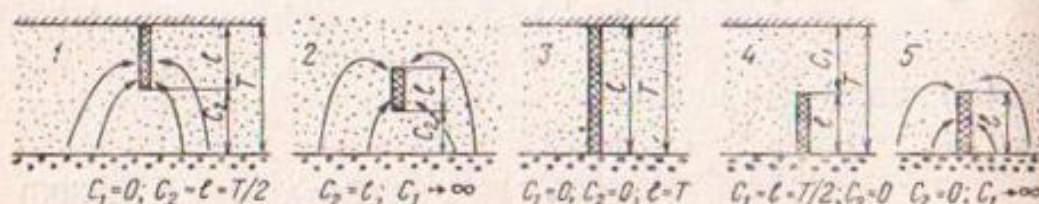
Рис. 35. Схемы расположения фильтра скважин в водоносном пласте.
