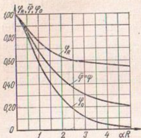
Рис. 29. Значения коэффициентов снижения напора в центре дренируемого массива \psi_0 , на его периферии \psi_R и среднее значение для всего массива \bar{\psi} в зависимости от параметра \alpha R .
