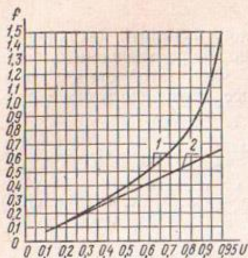
Рис. 34. Точные (1) и приближенные (2) значения сумм функции f .
