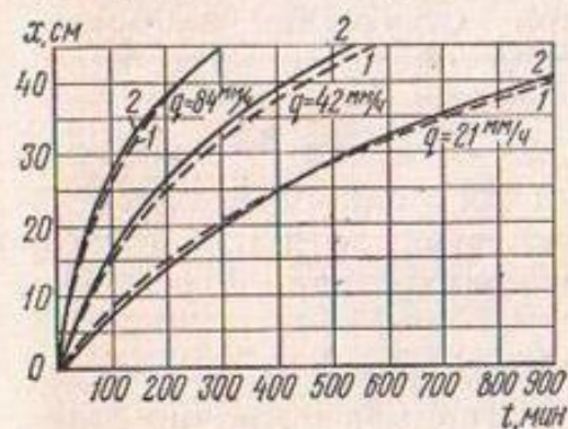
Рис. 13. Сравнение теоретических (кривая 1) и экспериментальных (кривая 2) данных по рассолению почвогрунтов при близком водоупоре.
