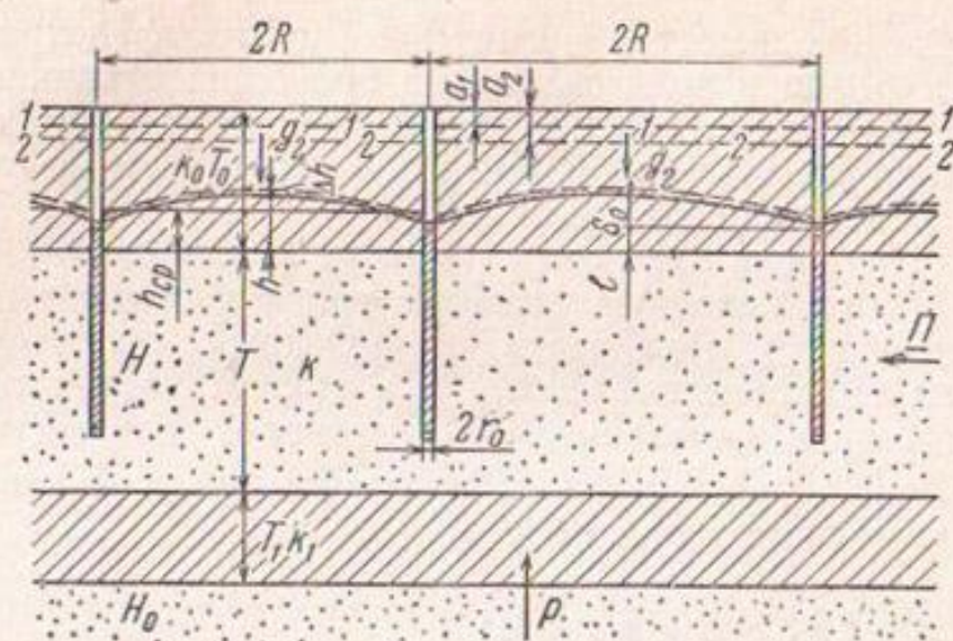
Рис. 40. Схема к расчету систематического вертикального дренажа.
