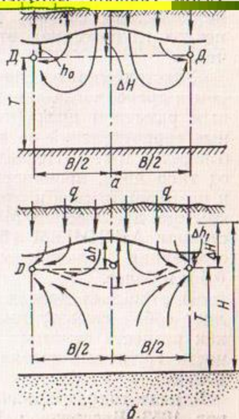
Рис. 21. Схемы работы горизонтального дренажа:
