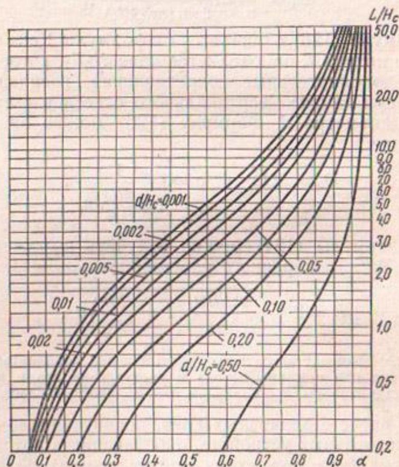
Рис. 23. График для определения коэффициента висячности дренажа \alpha :
