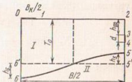
Рис. 54. Схема к расчету движения фильтрационного потока:
