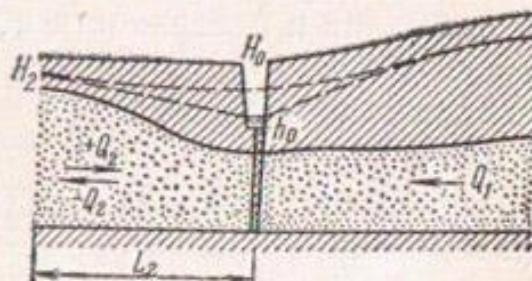
Рис. 44. Схема к расчету ловчего дренажа.
