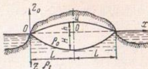
Рис. 45. Вытеснение засоленных грунтовых вод в условиях острова.
