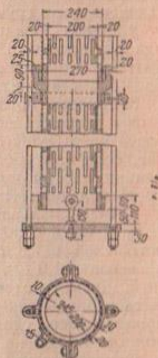
Фиг. 79г. Гончарный фильтр Принца
