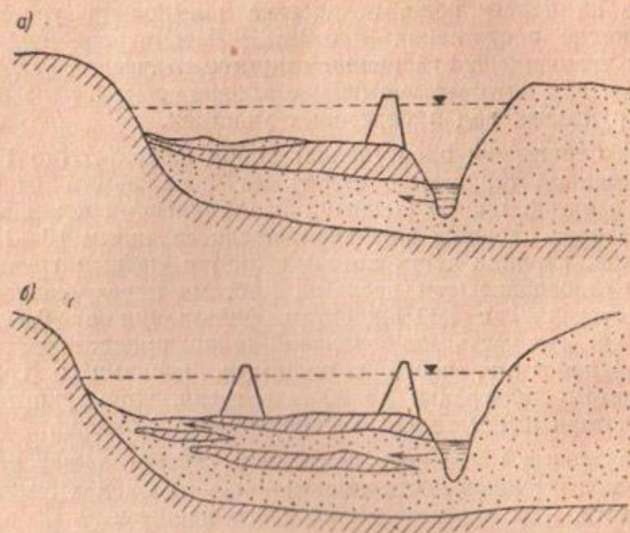
Фиг. 9. Схема расположения ограждающих дамб
