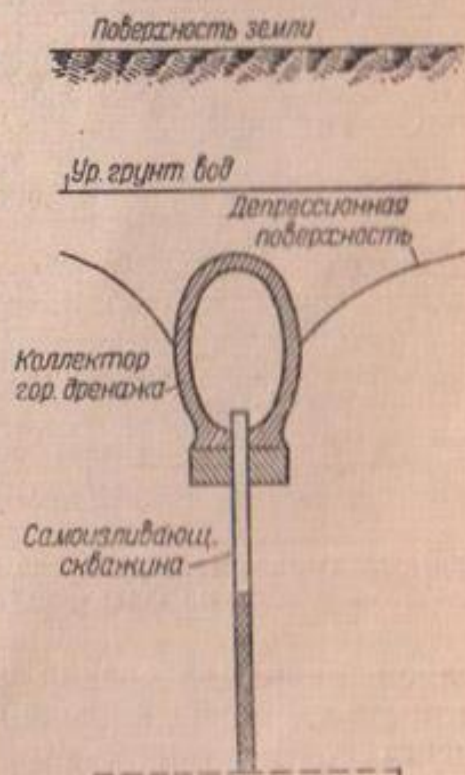
Фиг. 94. Общая схема комбинированного дренажа
