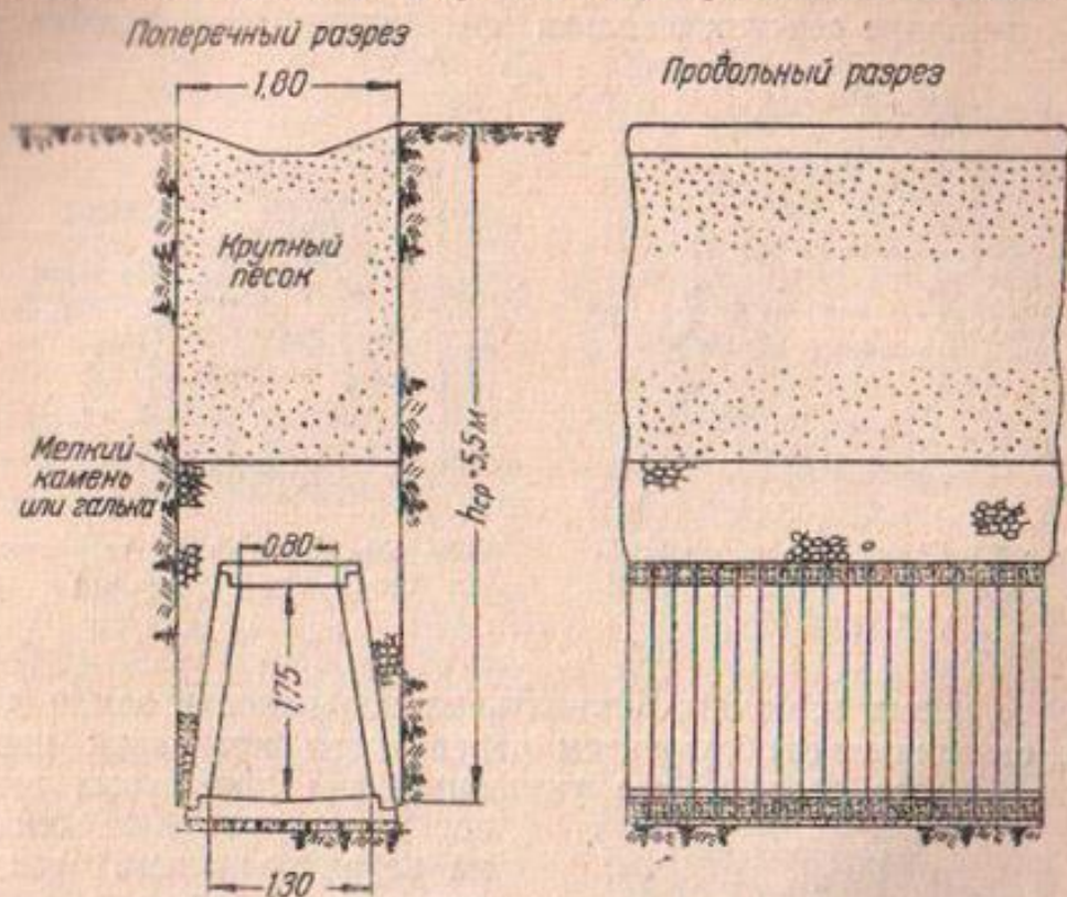
Фиг. 37. Деревянная дренажная галлерея
