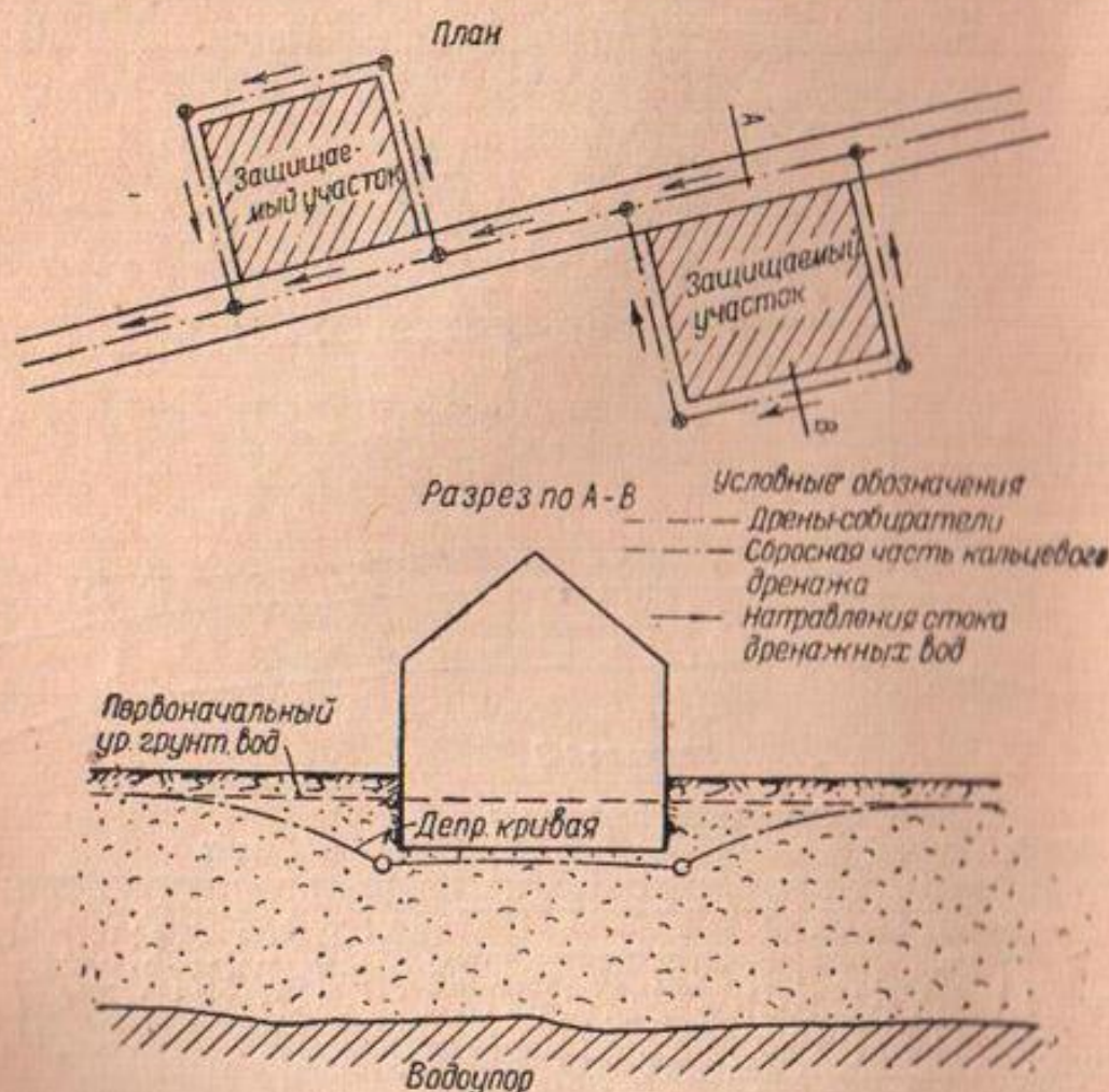
Фиг. 12. Схема кольцевого дренажа
