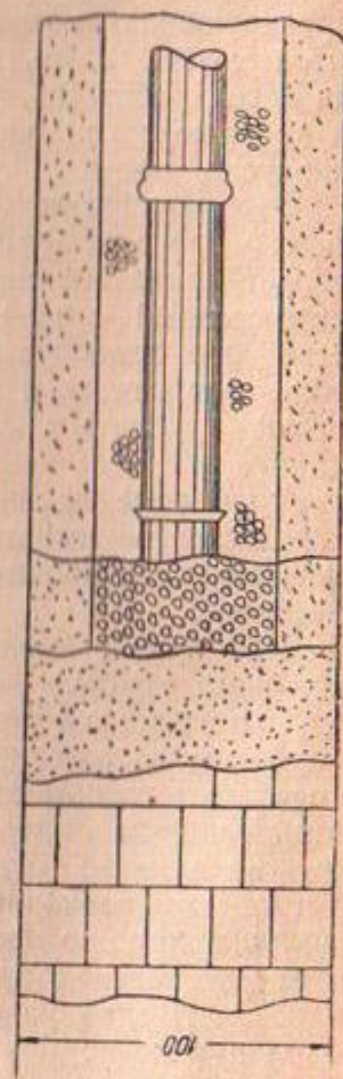
Фиг. 24. Трубчатый дренаж
