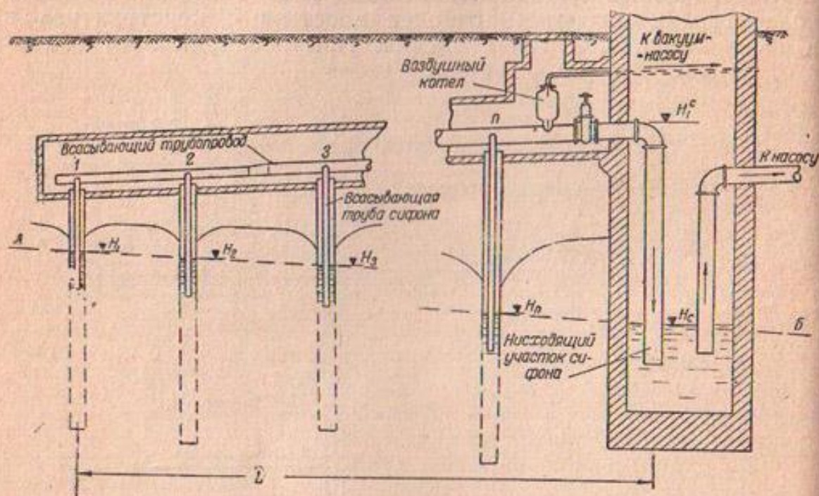
Фиг. 886. Схема дренажной завесы с сифонным устройством
