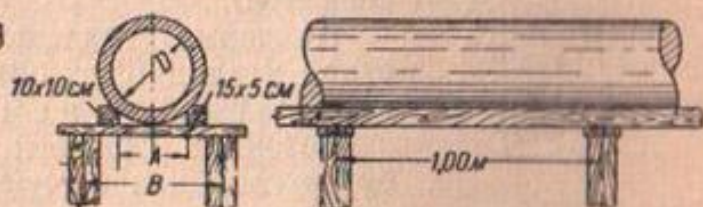
Фиг. 35. Брусчатые стеллажи на сваях
