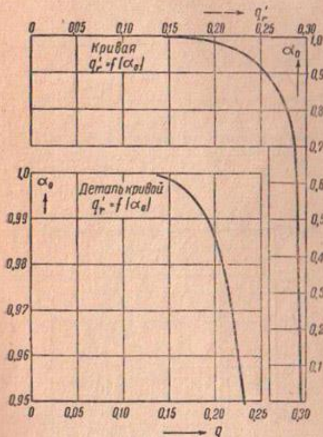
Фиг. 51. График для нахождения величины q_r'
