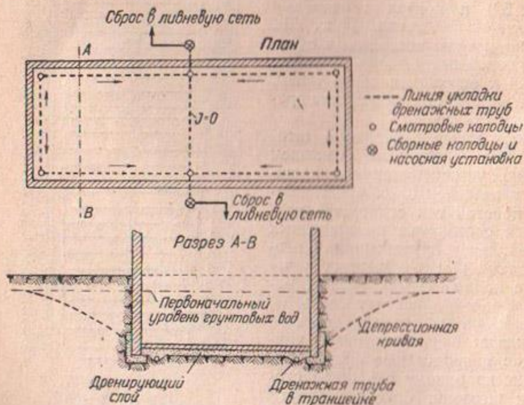
Фиг. 44. Схема внутреннего дренирования заглубленных сооружений
