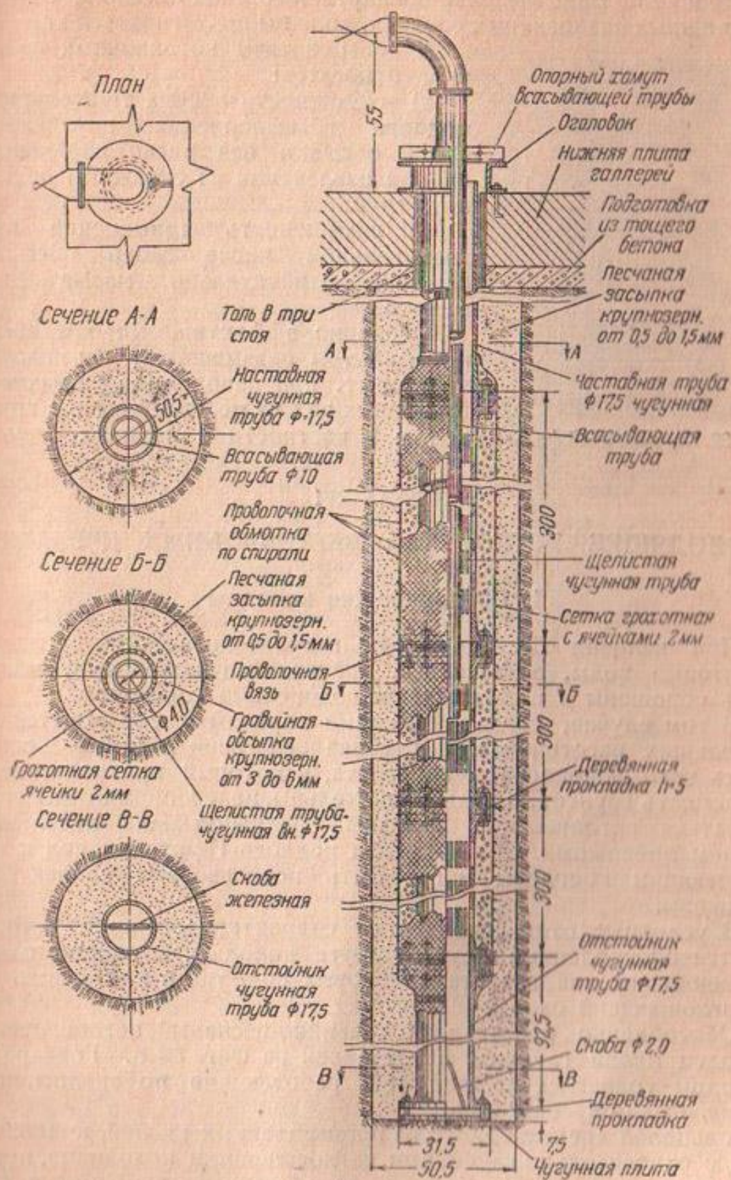
Фиг. 81. Чугунный фильтр с обсыпкой
