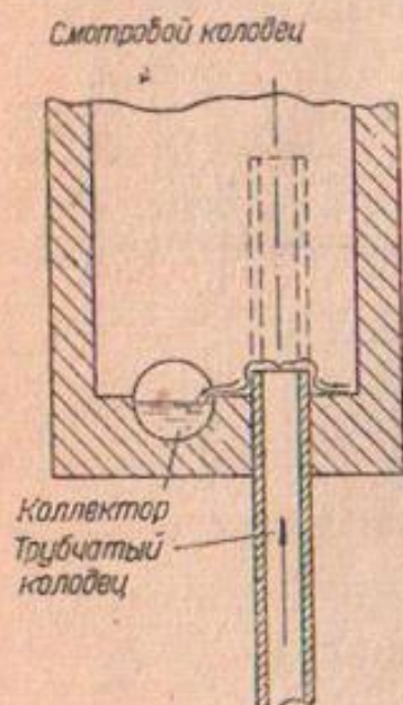
Фиг. 87. Схема присоединения трубчатого колодца к коллектору
