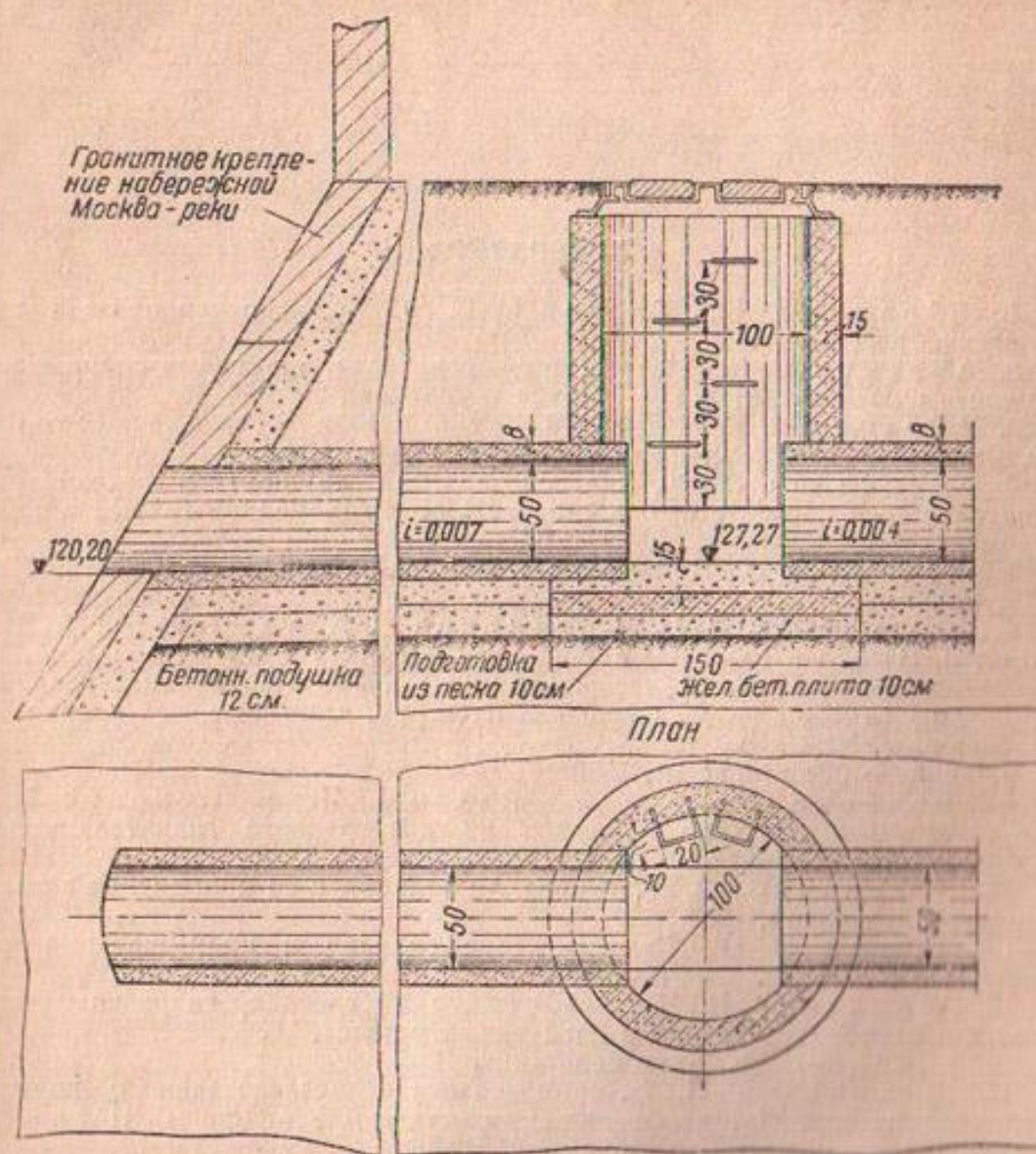
Фиг. 106. Выпуск дренажных вод через стенки набережной
