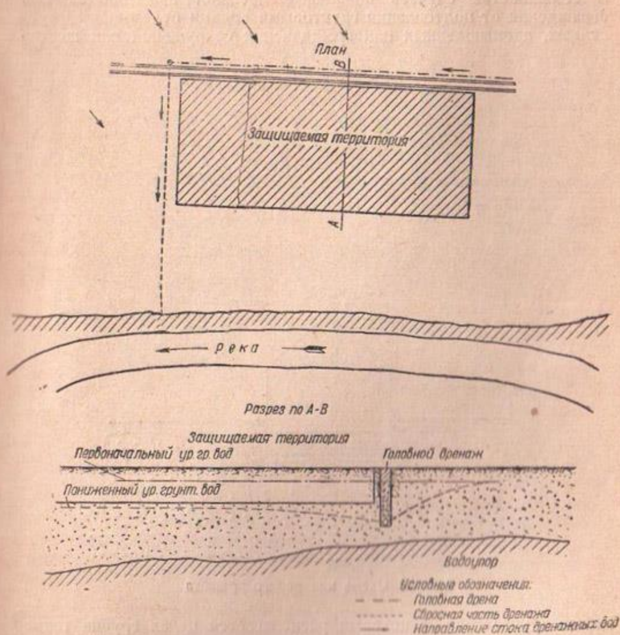
Фиг. 11. Схема головного дренажа
