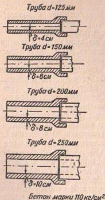
Фиг. 26. Бетонные дренажные трубы малых размеров
