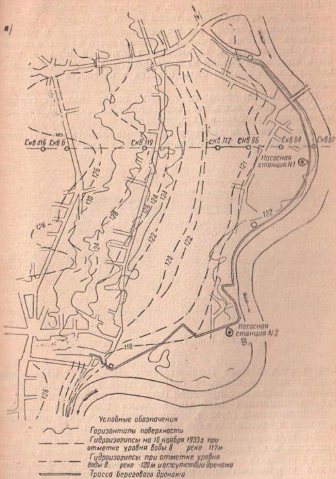
Фиг. 72а. План дренажа
