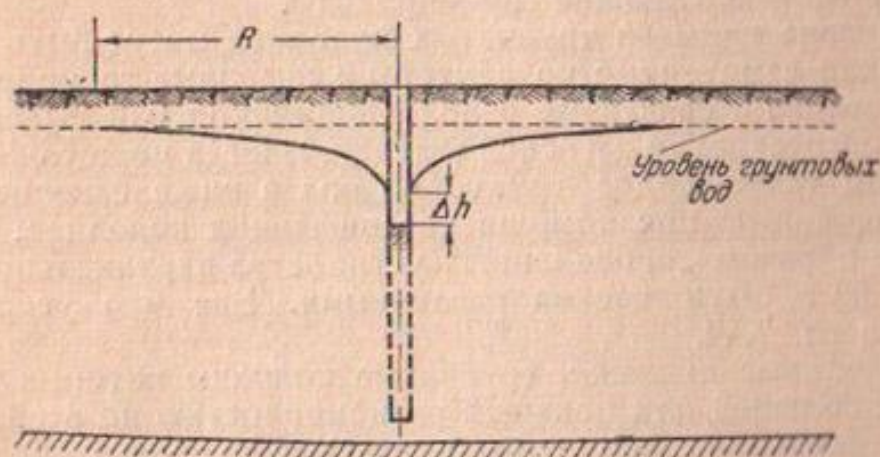
Фиг. 70б. Схема понижющего действия трубчатого колодца
