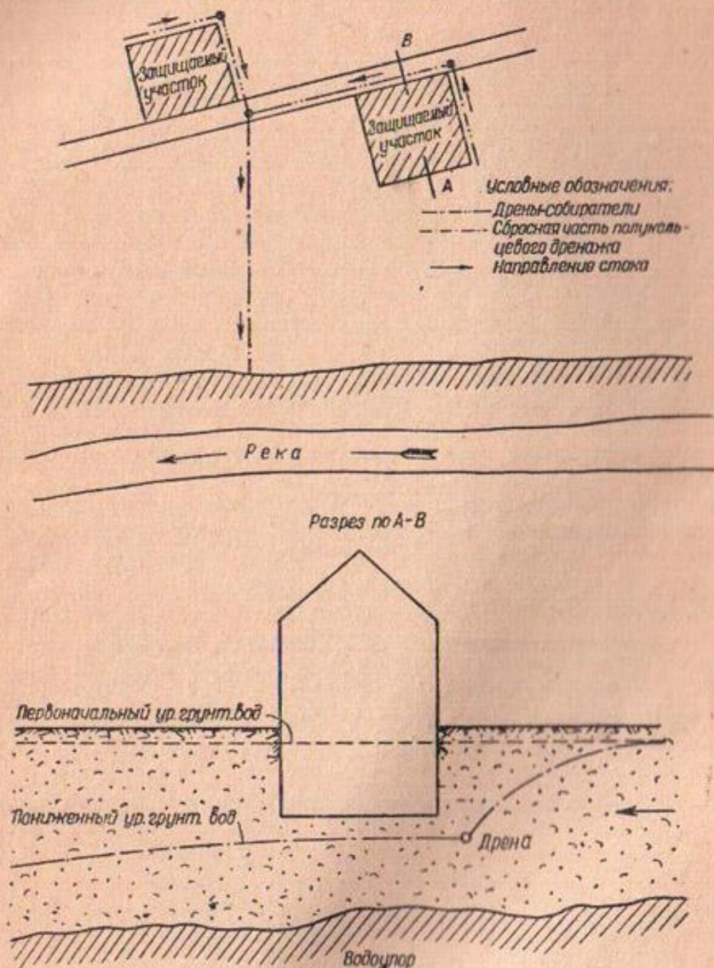
Фиг. 13. Схема полукольцевого дренажа
