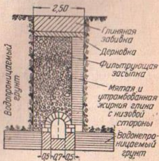
Фиг. 38. Дренажная галлерея с экраном
