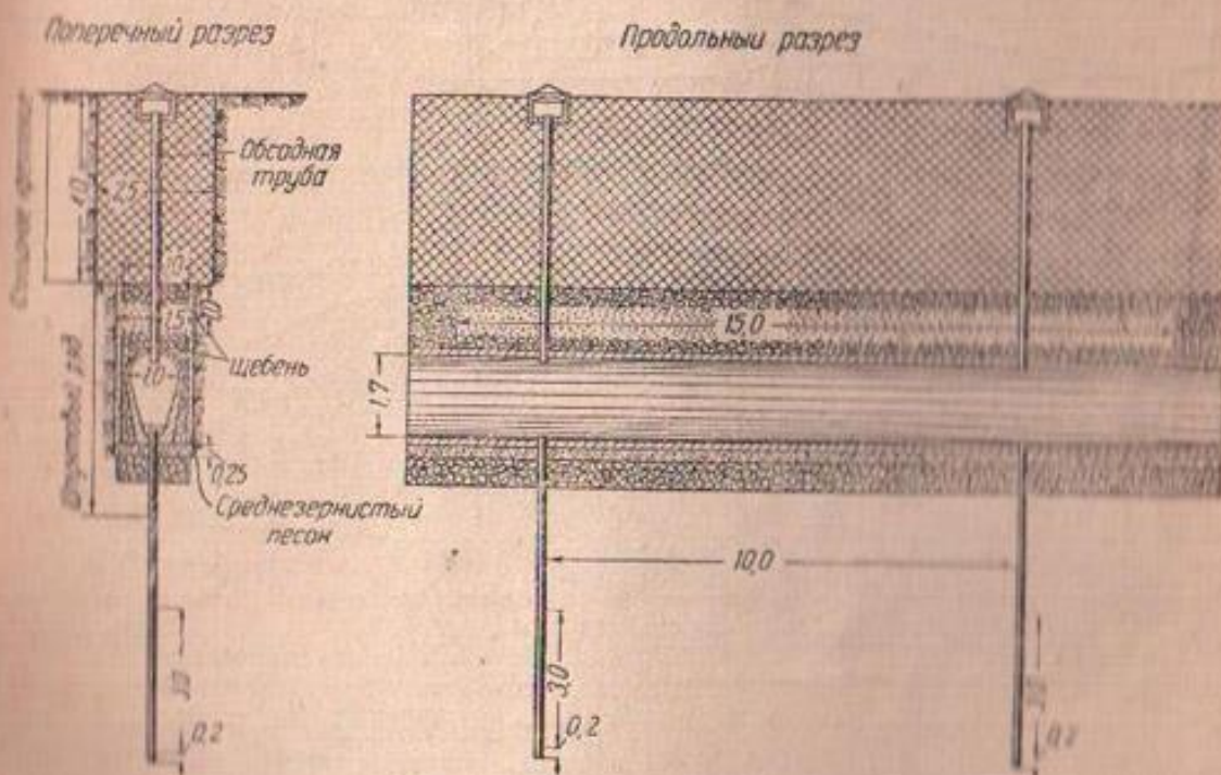
Фиг. 97. Конструкция комбинированного дренажа
