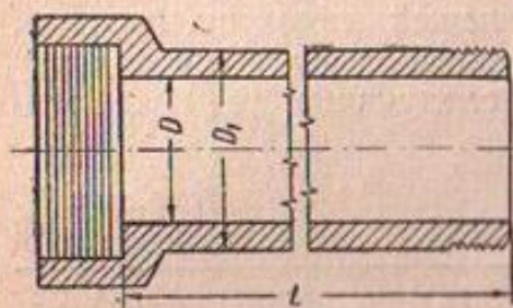
Фиг. 25. Керамиковые дренажные трубы
