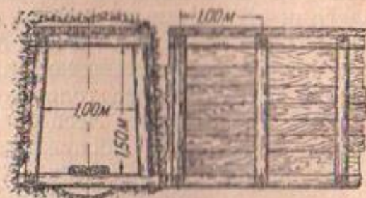
Фиг. 42. Временное крепление штольни облегченного типа
