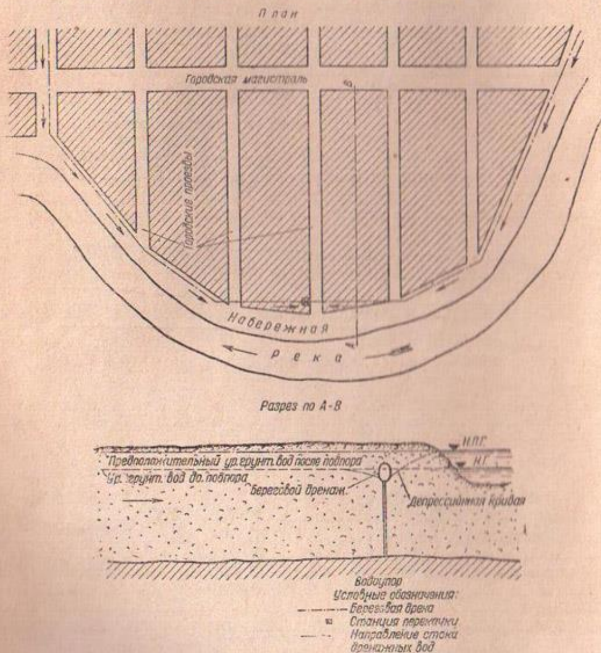
Фиг. 14. Схема берегового дренажа
