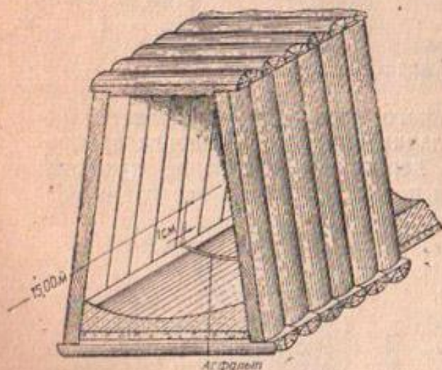
Фиг. 41. Сплошное крепление штольни вязаными рамами
