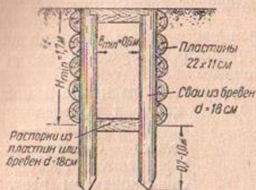
Фиг. 17. Дренажный лоток свайного типа
