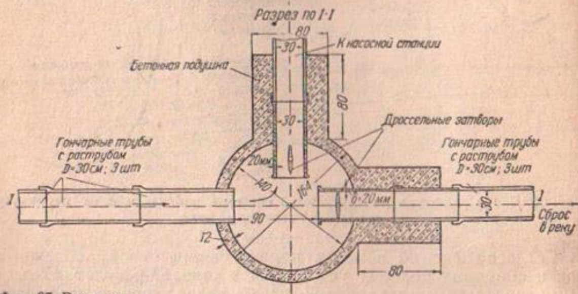
Фиг. 67. Распределительный колодец с дроссельным затвором
