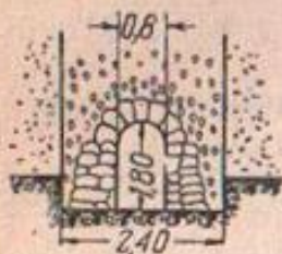
Фиг. 36. Дренажная галлерей из каменной кладки
