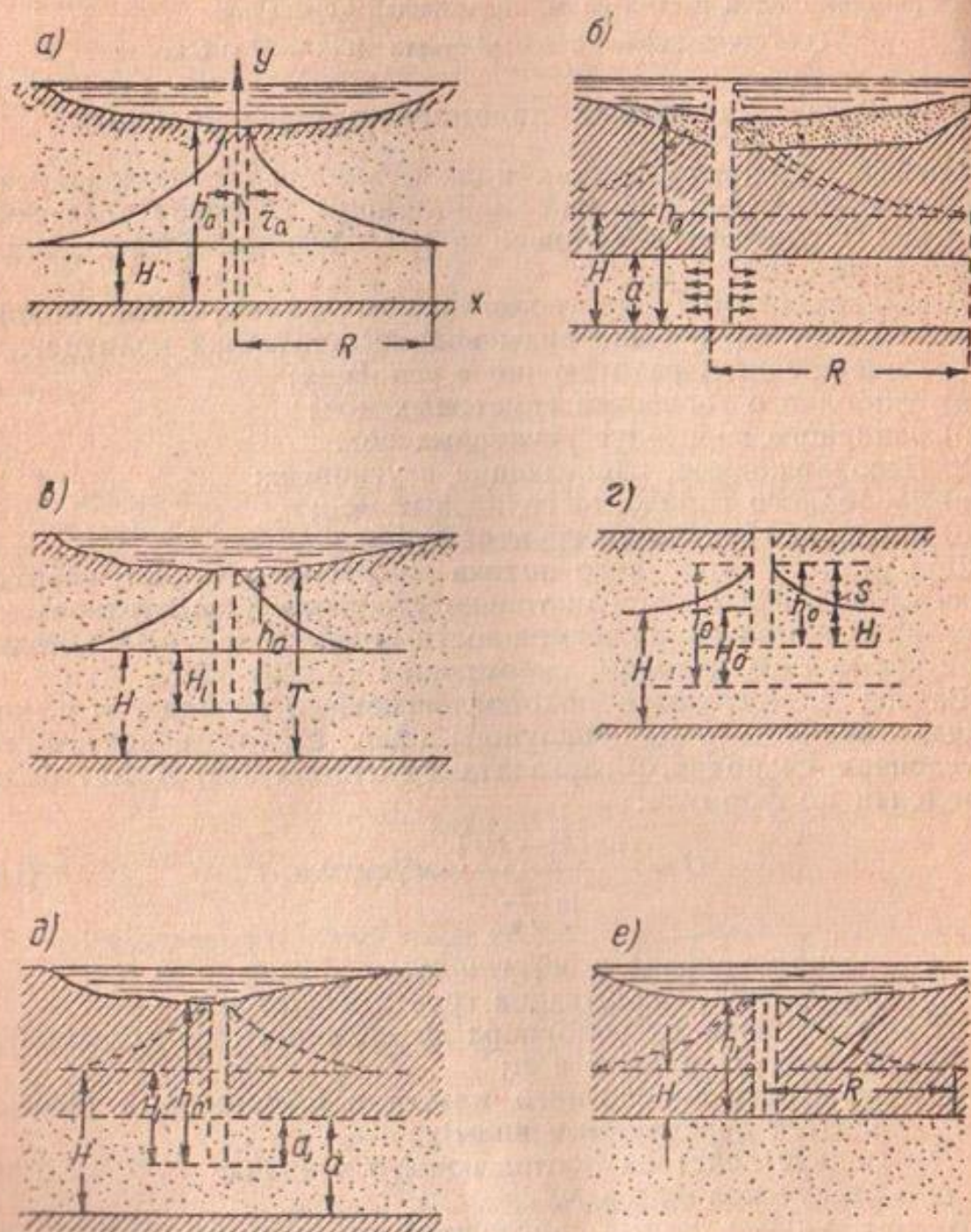
Фиг. 92. Схемы поглощающих колодцев
