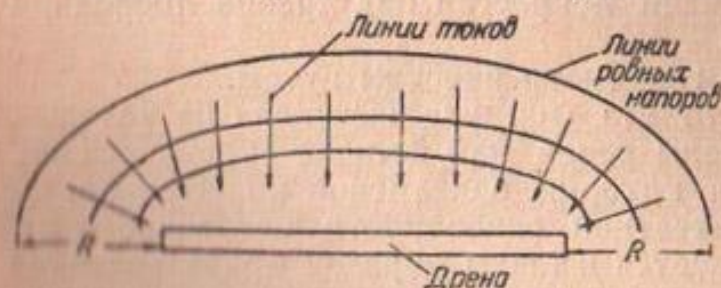
Фиг. 47. Схема притока воды к короткой дрены
