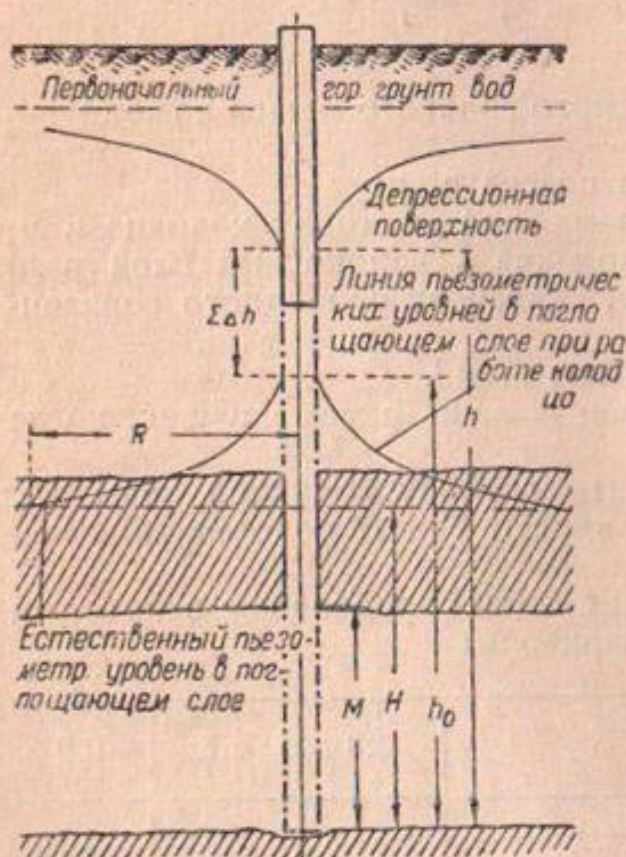
Фиг. 93. Схема к расчету поглощающих колодцев
