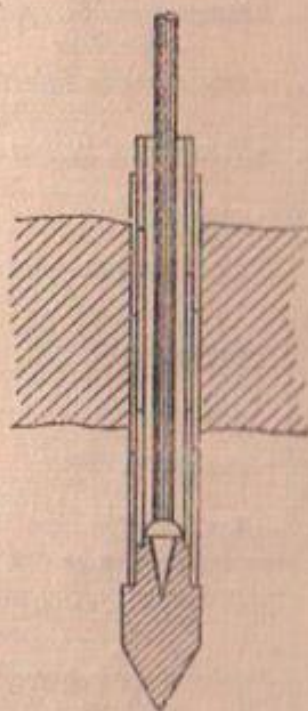
Фиг. 73. Вертикальная дрена голландского дренажа
