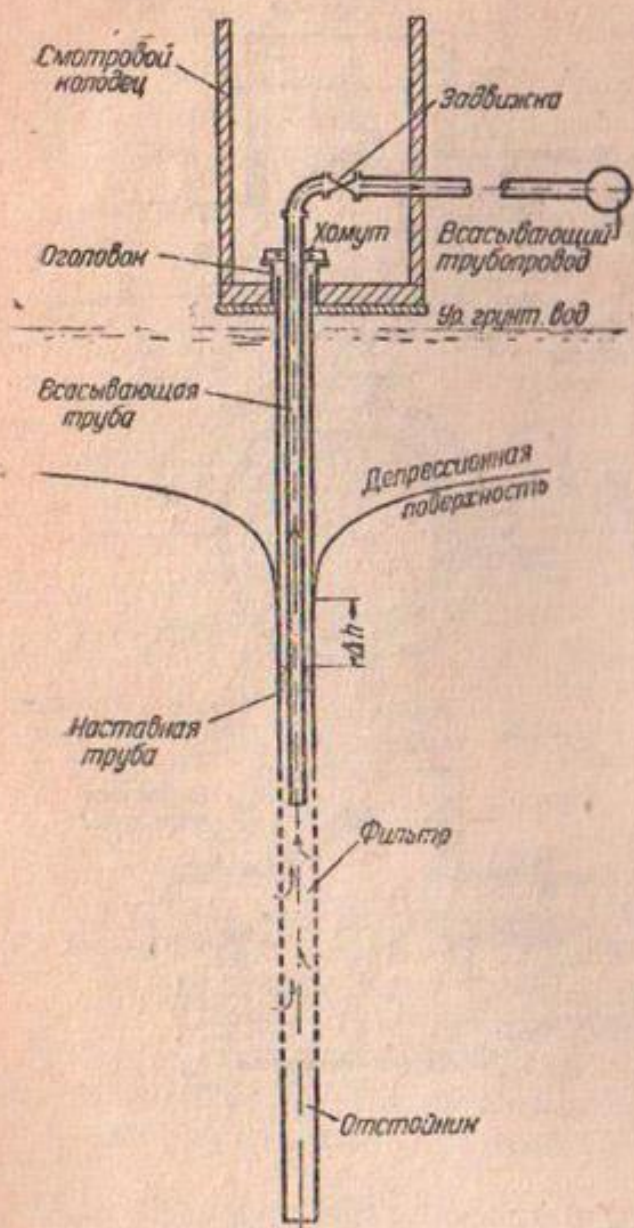
Фиг. 70а. Общая схема трубчатого колодца
