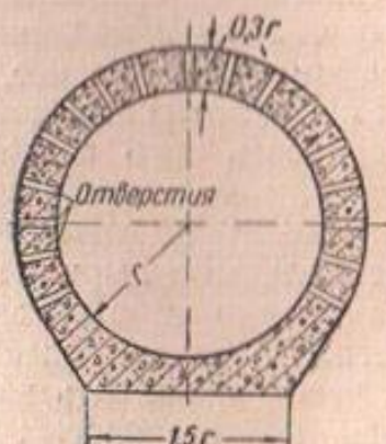
Фиг. 27. Бетонные дренажные трубы с плоским основанием
