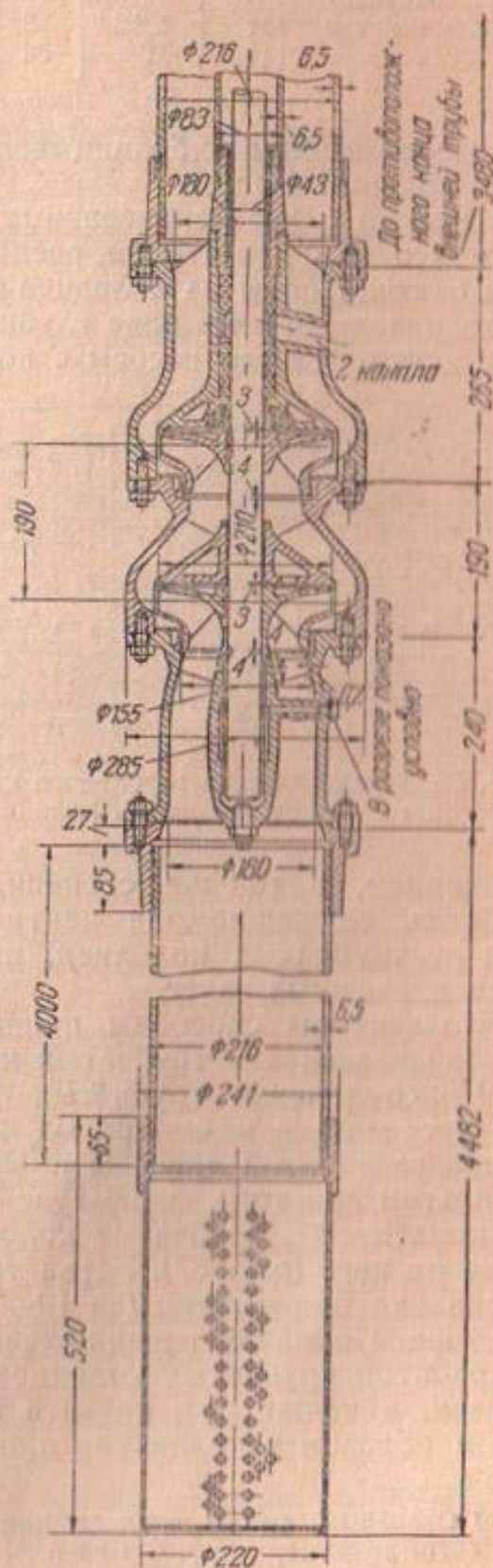
Фиг. 84. Разрез глубинного насоса
