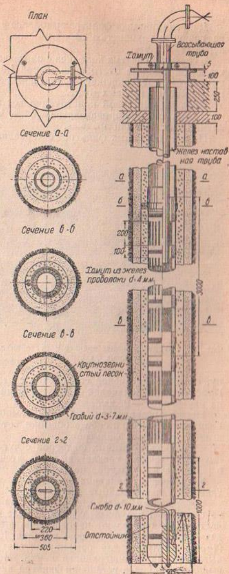
Фиг. 80а. Деревянный фильтр с обсыпкой
