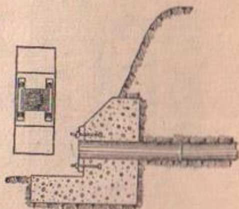
Фиг. 63. Устье дренажа американского типа
