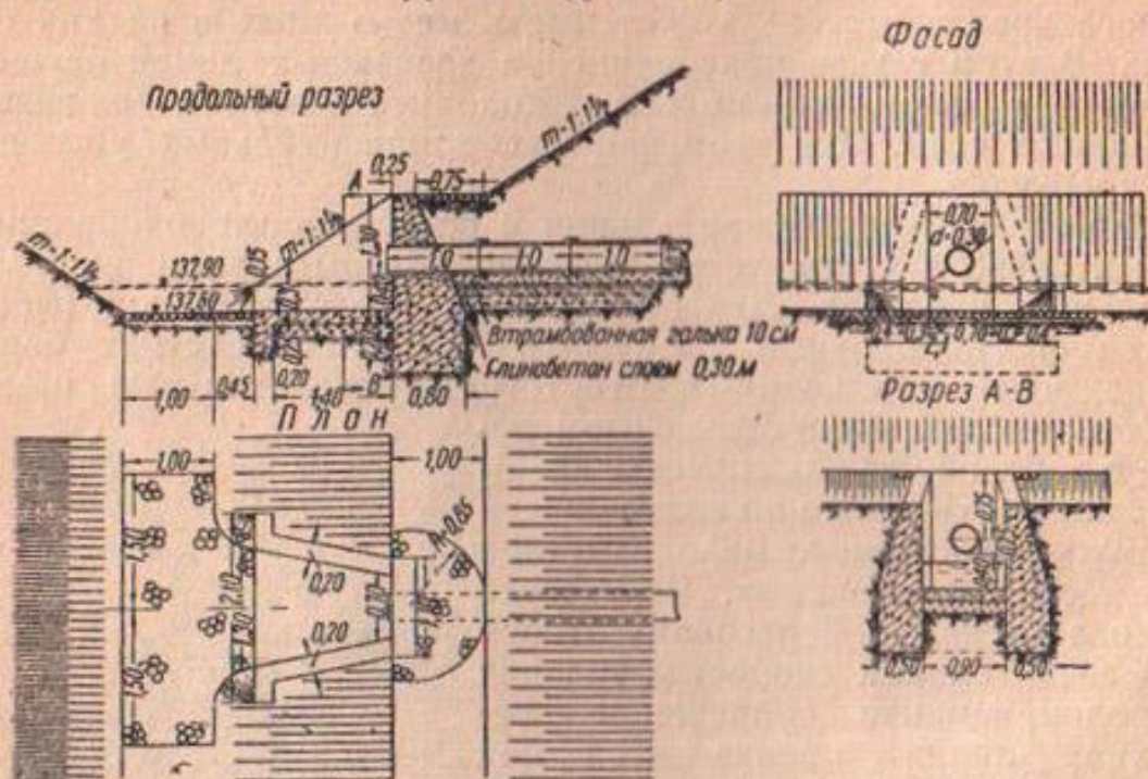
Фиг. 64. Устье дренажа в виде бетонного оголовка
