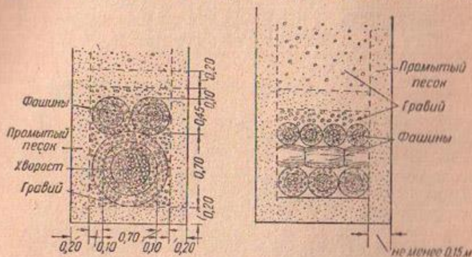
Фиг. 22. Фашинные дренажи
