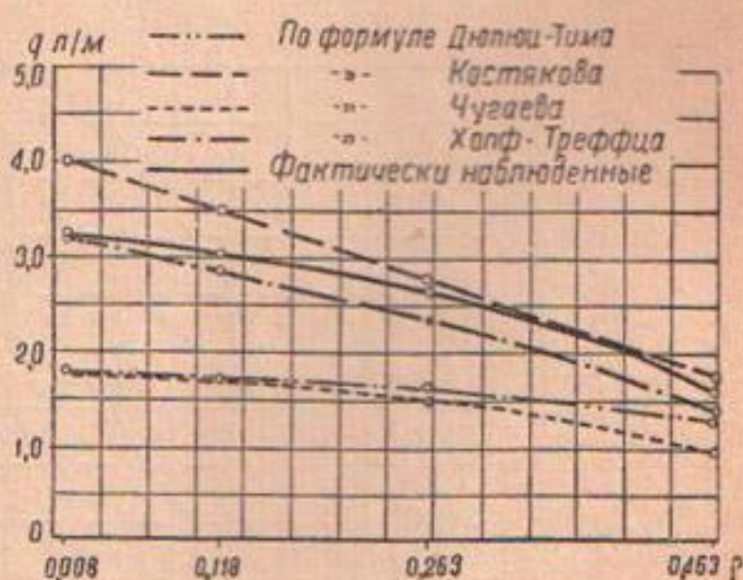
Фиг. 53. Кривые дебита незатопленных одиночных дрена в зависимости от их положения над водоупором для условий потока
