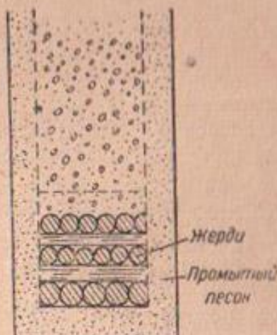
Фиг. 21. Жердевой дренаж
