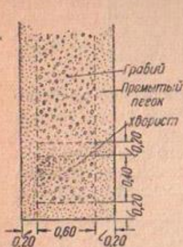
Фиг. 20. Хворостяной дренаж
