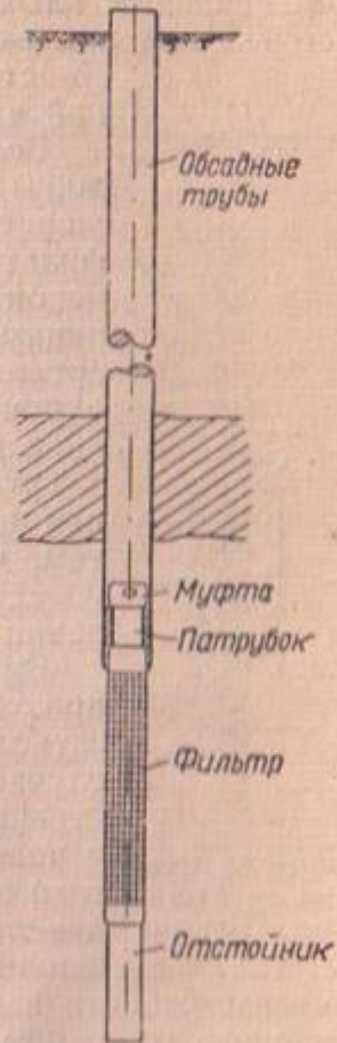
Фиг. 75. Схема трубчатого колодца
