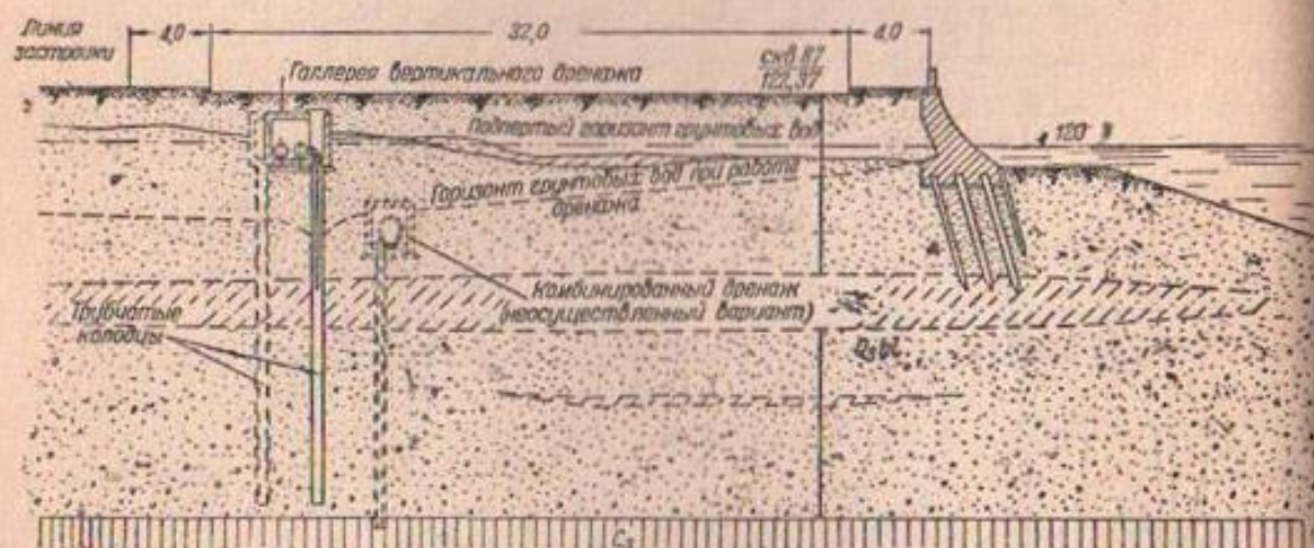
Фиг. 726. Поперечный разрез по дренажу
