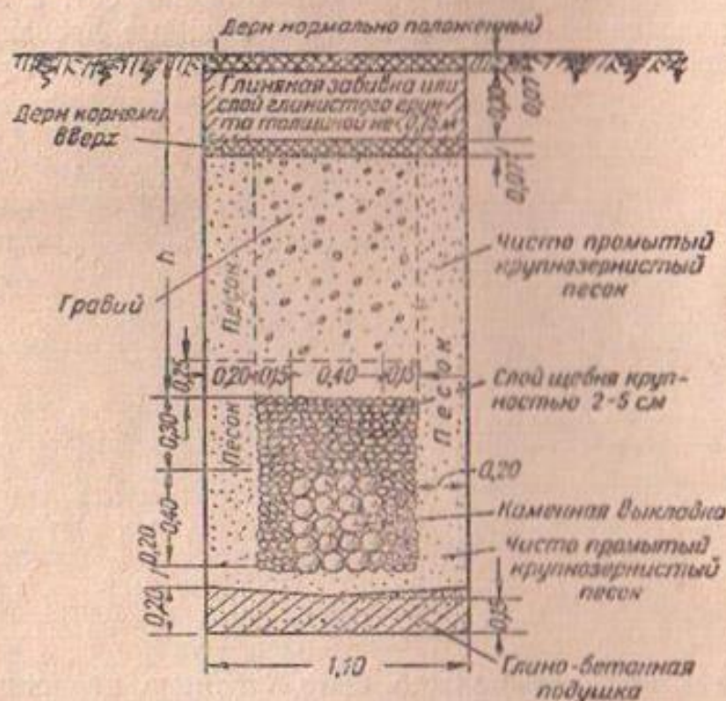
Фиг. 23. Каменно-щебенчатый дренаж
