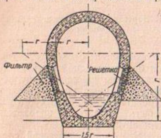
Фиг. 28. Бетонные дренажные трубы овоидальной формы
