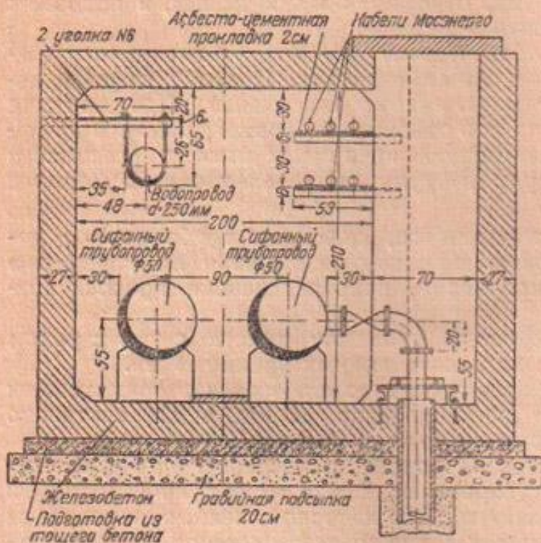
Фиг. 89а. Поперечный разрез по галлерее берегового дренажа
