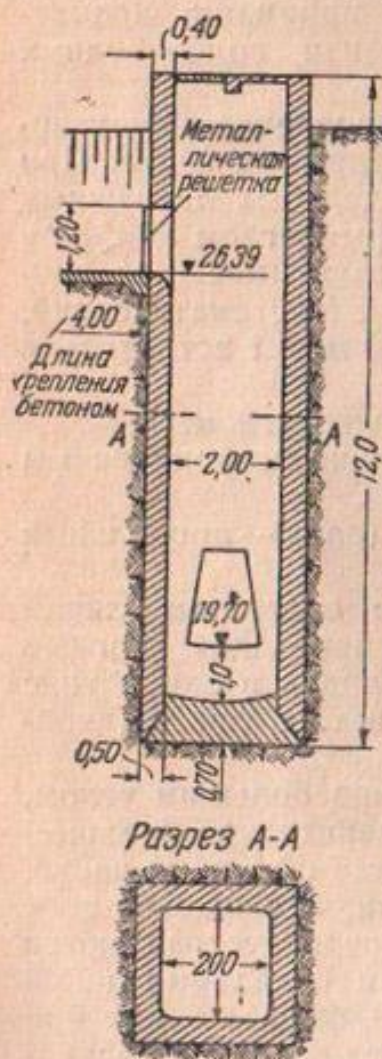
Фиг. 61. Шахтный бетонный колодец
