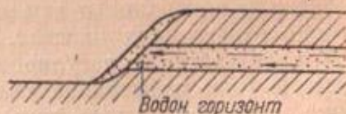
Фиг. 3. Выход грунтового потока в склоне
