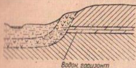
Фиг. 4. Выклинивание водоносного горизонта в аллювий
