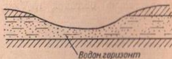
Фиг. 5. Заболачивание подземными водами
