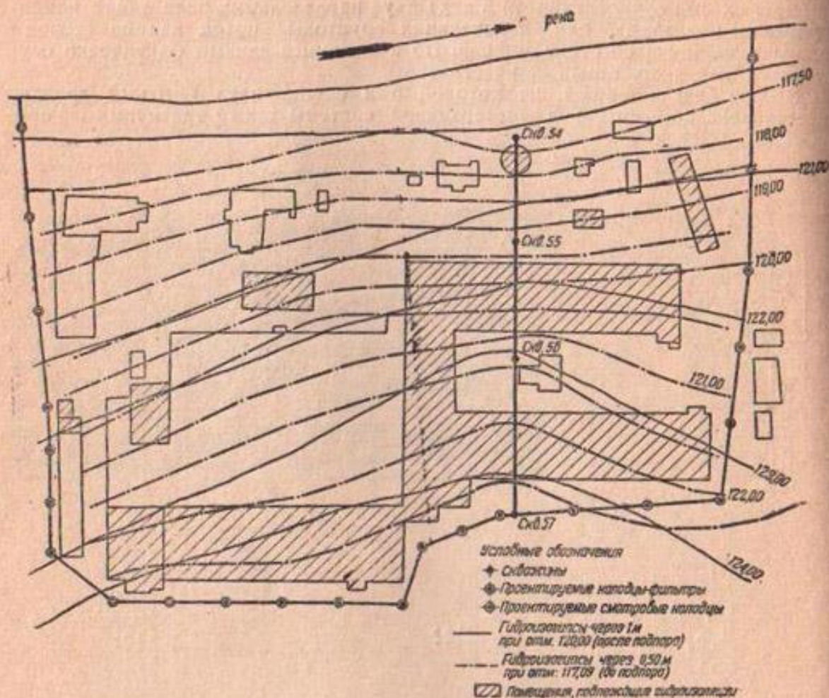
Фиг. 98. Схема расположения комбинированного дренажа.
