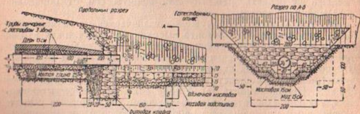
Фиг. 65. Выход дрены в открытый канал
