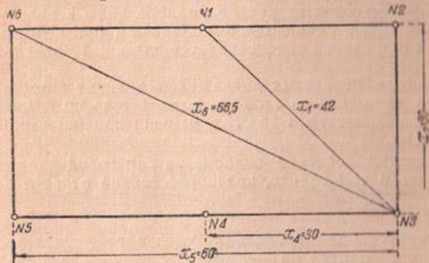
Фиг. 91. Схема к расчету кольцевого дренажа
