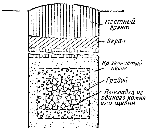
Рис. 69. Каменно-щебеночный водозабор
