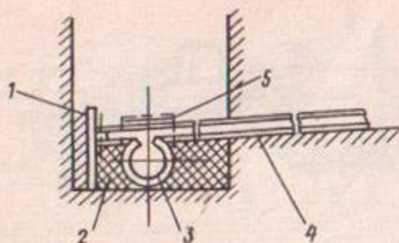
Рис. 48. Соединение дренажной линии с коллектором:
