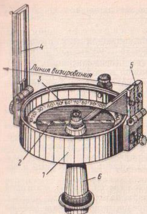
Рис. 5. Буссоль:
