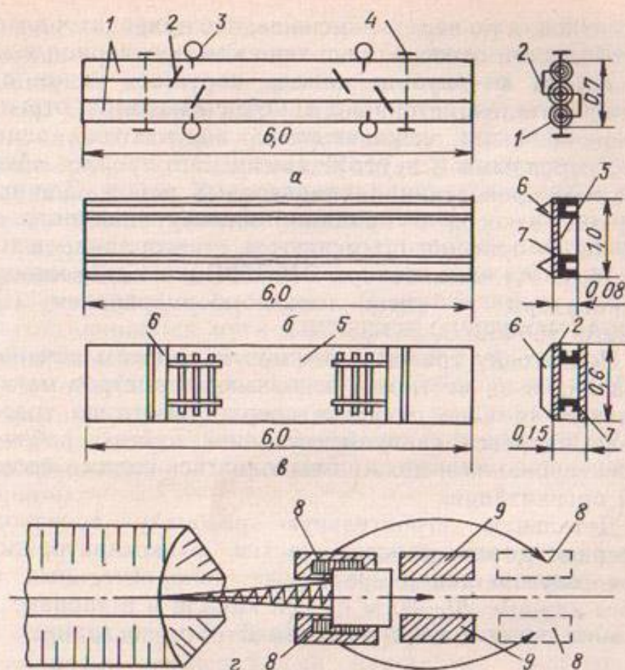
Рис. 30. Разработка грунта одноковшовыми экскаваторами со сланей:
