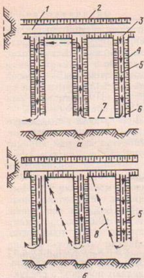
Рис. 37. Схема движения каналокопателя:
