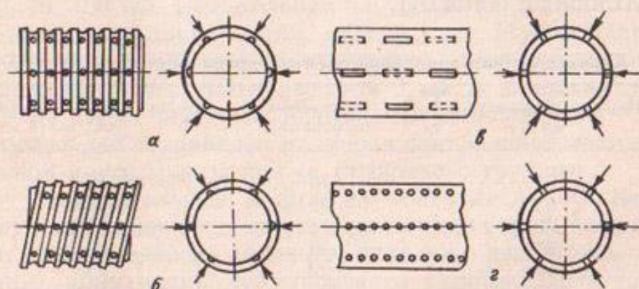
Рис. 24. Пластмассовые дренажные трубы:
