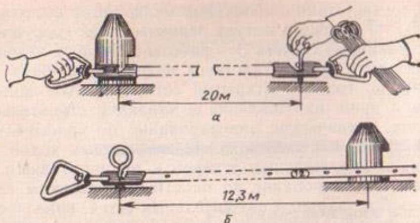
Рис. 1. Стальная мерная лента:
