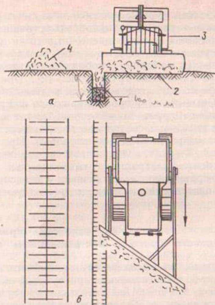
Рис. 49. Схема засыпки траншеи гумусированным (растительным) грунтом:
