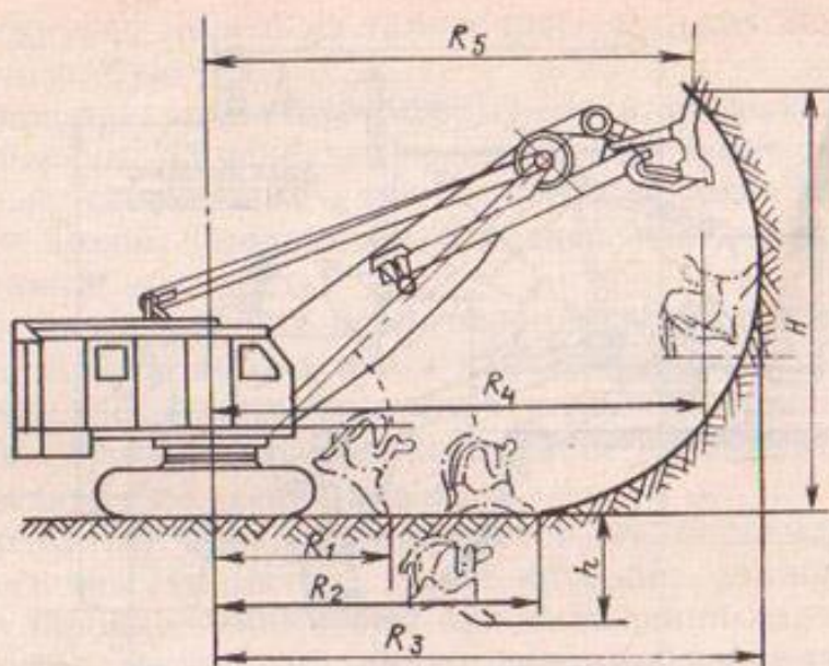
Рис. 42. Рабочие размеры экскаватора, оборудованного прямой лопатой:
