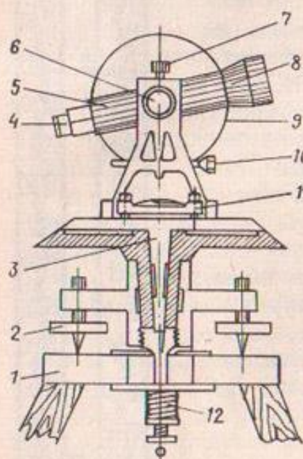
Рис. 4. Теодолит:
