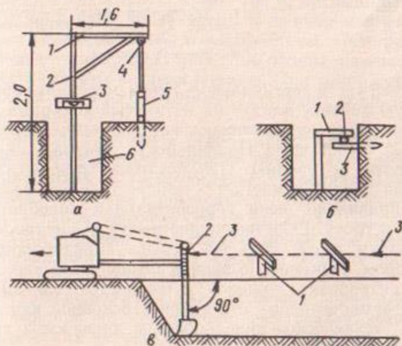
Рис. 60. Способы контроля глубины копания траншей:
