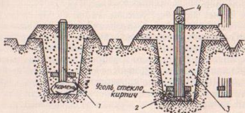
Рис. 13. Геодезические знаки (реперы):
