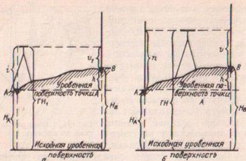
Рис. 12. Способы нивелирования: а — вперед; б — из середины
