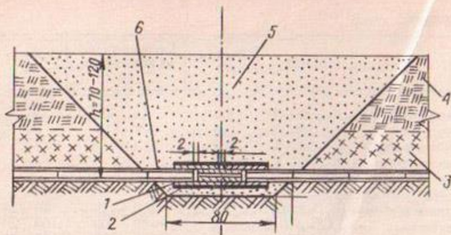
Рис. 22. Поглощительная колонка:
