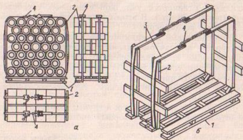
Рис. 26. Контейнеры для перевозки керамических труб:
