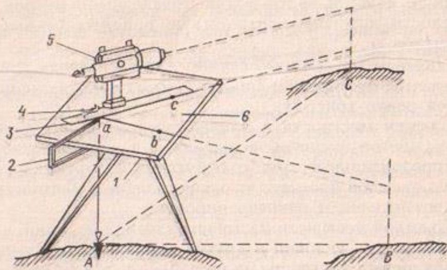
Рис. 7. Мензула:
