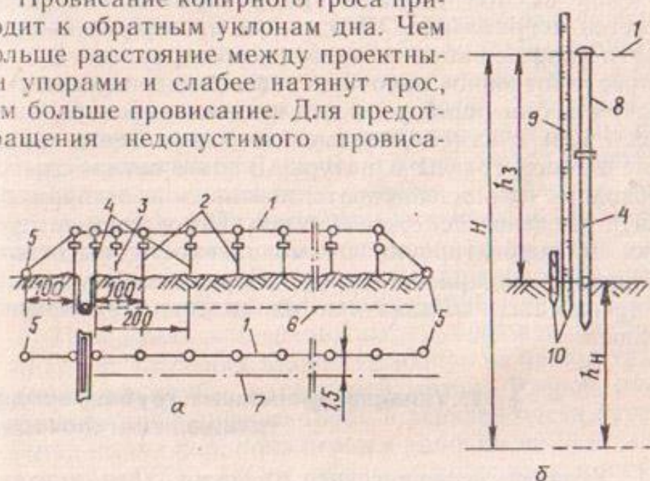
Рис. 45. Установка копирного троса на фиксирующие упоры:
