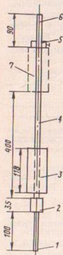
Рис. 57. Ударник ДорНИИ:
