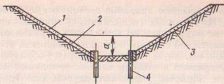
Рис. 44. Крепление откосов каналов:
