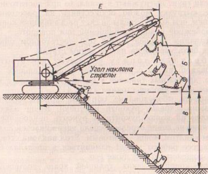
Рис. 40. Схема экскаватора Э-652Б с драглайном:
