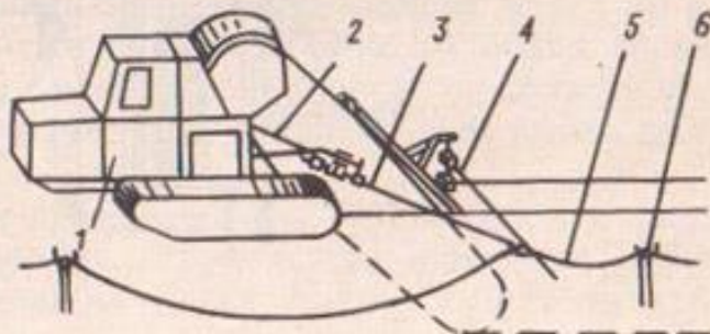
Рис. 54. Схема установки люнета на экскаваторе-дреноукладчике:
