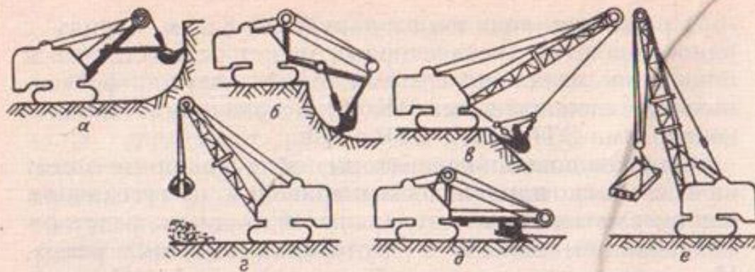
Рис. 39. Экскаватор со сменным оборудованием:
