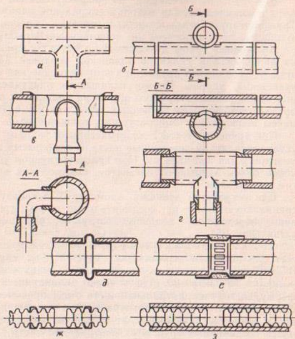
Рис. 25. Дренажная арматура:
