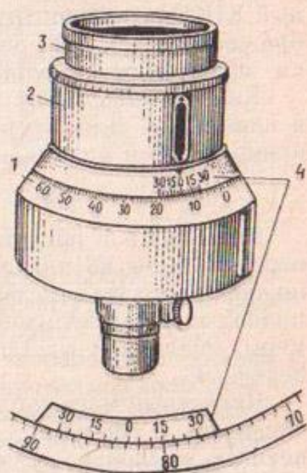
Рис. 6. Гониометр:
