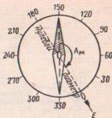
Рис. 11. Схема измерения угла по азимуту
