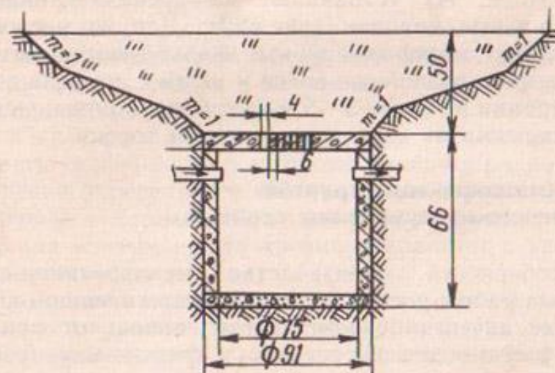
Рис. 21. Поглощающий колодец:
