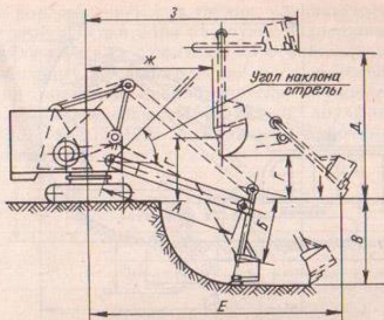
Рис. 41. Схема экскаватора Э-652Б с обратной лопатой:
