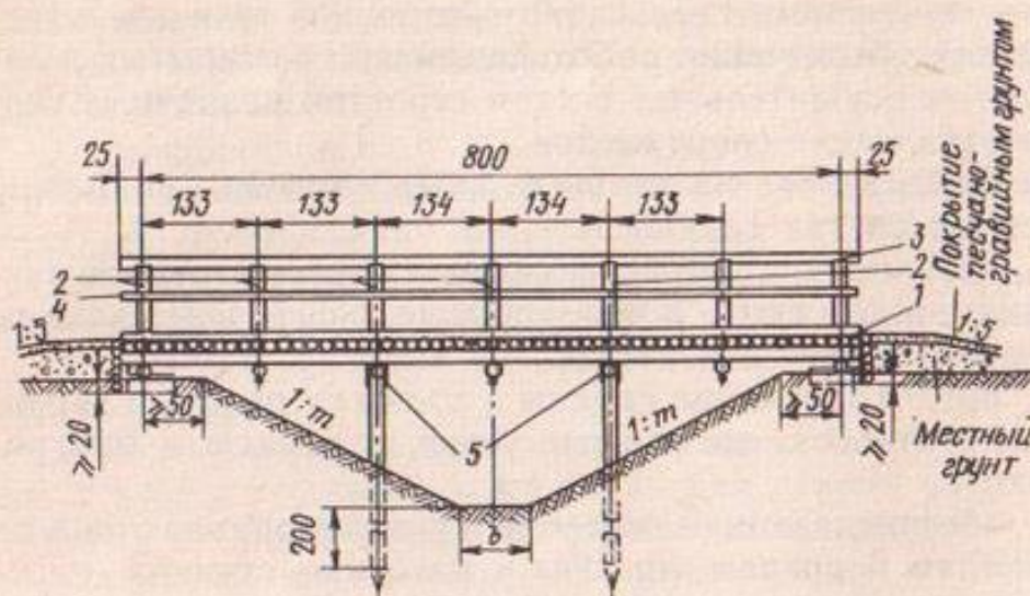
Рис. 17. Типовая конструкция деревянного пешеходного моста:
