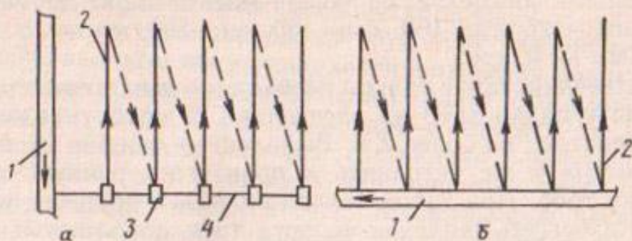
Рис. 50. Технологические схемы бестраншейной укладки дренажа: а — при впадении дрен в закрытый коллектор; б — при впадении дрен в открытый канал; 1 — открытый канал; 2 — дрена; 3 — приямок; 4 — закрытый коллектор
