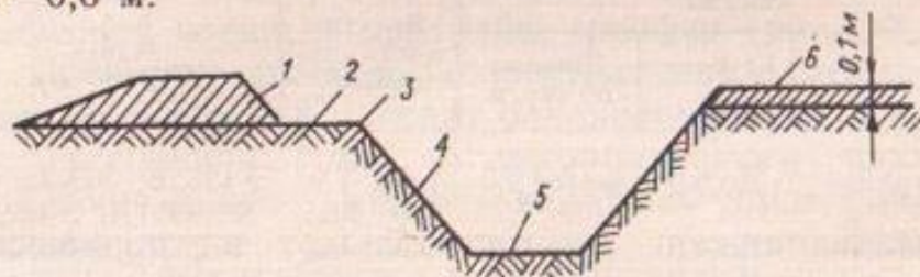
Рис. 38. Профиль осушительного канала:
