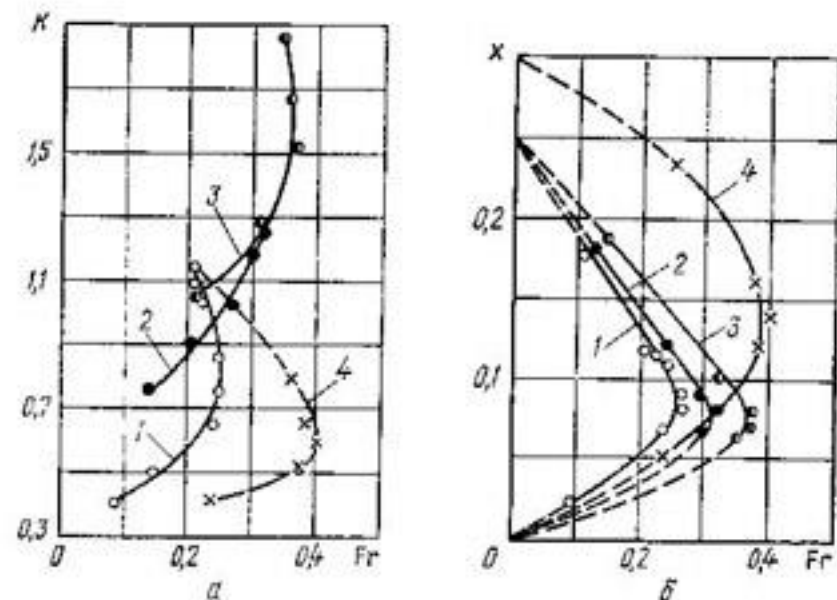
Рис. 47. График зависимости \kappa = \kappa(Fr) (а) и x = x(Fr) (б): 1, 2, 3 — песчаное дно ( d_{cp} = 0,21 мм) с уклонами соответственно I = 0,0012 , I = 0,0025 и I = 0,005 ; 4 — дно сложено из мелкой гальки ( d_{cp} = 5,2 мм), I = 0,0025 .
