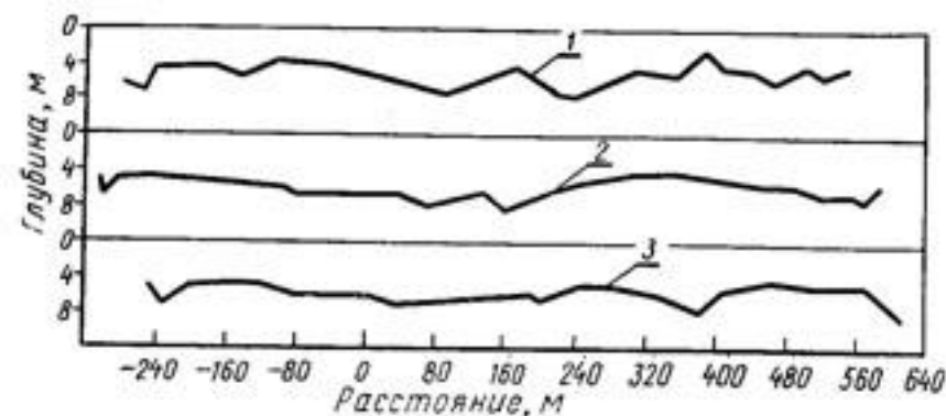
Рис. 32. Продольные профили канала в мелкопесчаных грунтах:
