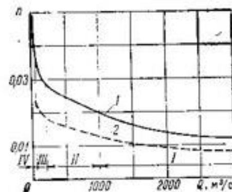
Рис. 52. Классификация земляных каналов по гидравлическим сопротивлениям, характеризующим коэффициентом шероховатости n и пропускной способностью Q :
