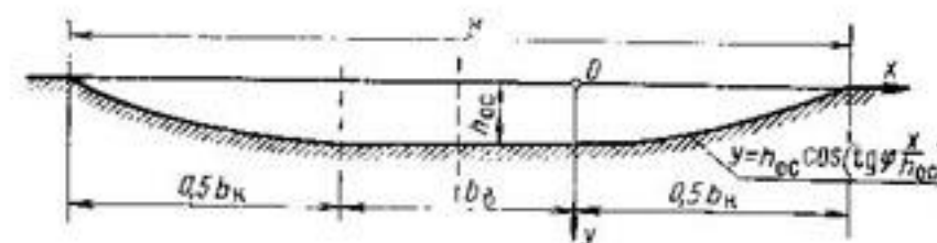
Рис. 54. Безмерный профиль живого сечения канала, рассчитанный по методу влекущей силы: b_0 — ширина вставки.
