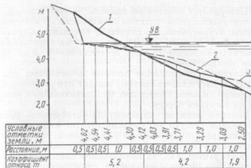
Рис. 8. Формирование левого берега Каракумского канала под воздействием волн: 1 — 1971 г.; 2 — 1973 г.; 3 — 1975 г.
