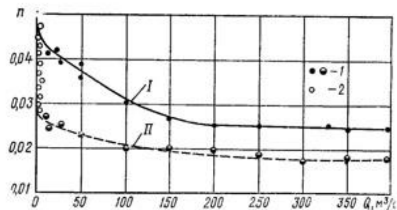
Рис. 36. График зависимости максимальных (I) и минимальных (II) коэффициентов шероховатости n при различных расходах воды Q : 1 — натура; 2 — модель.
