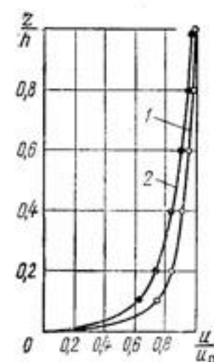
Рис. 45. Эпюры распределения продольных скоростей на вертикали: 1 — поток без взвешенных наносов ( x_c = 0,09 ); 2 — взвесенесущий поток ( S_d \approx 15 кг/м³) при x_n = 0,18 .
