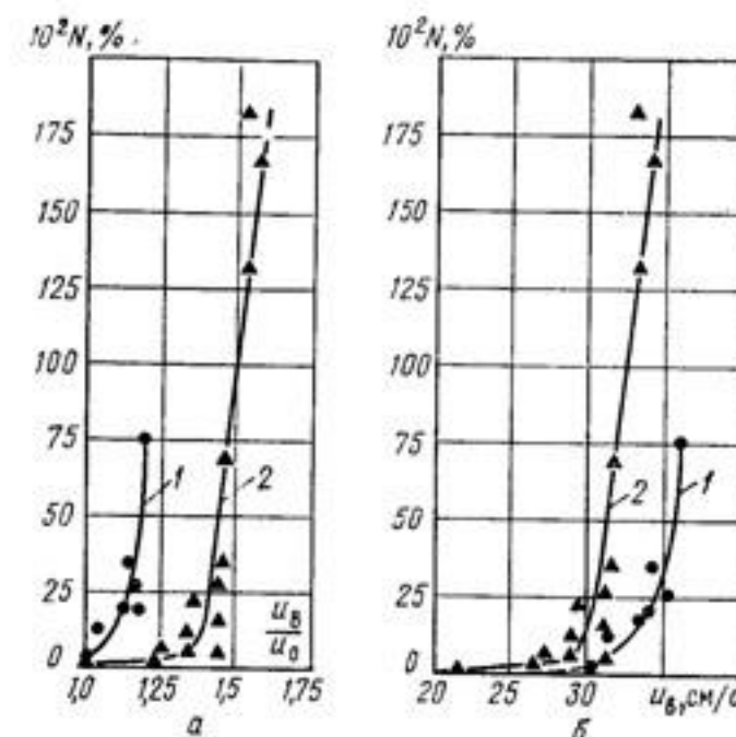
Рис. 43. Зависимости характеристики N от относительной скорости u/u_0 (а) и средней скорости на вертикали u_v (обозначения те же, что и на рис. 42).
