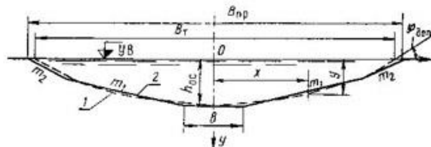
Рис. 55. Схема поперечного сечения канала, принятая В. П. Троицким при уточнении метода влекущей силы: 1 — теоретическое сечение; 2 — проектное, ( B_t , B_{пр} — ширина соответственно теоретического и проектного сечений канала).
