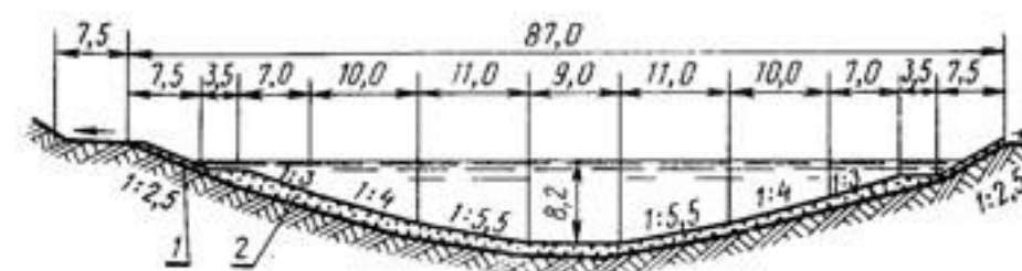
Рис. 19. Типовое поперечное сечение Каховского магистрального канала:
