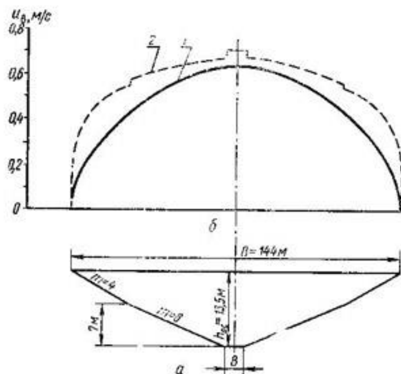
Рис. 56. Поперечный профиль канала (а) в мелкопесчаных грунтах, рассчитанный по методу эпюр скоростей (б) при расходе воды Q=600 \text{ м}^3/\text{с} : 1 — эпюра скоростей течения; 2 — эпюра допустимых скоростей.
