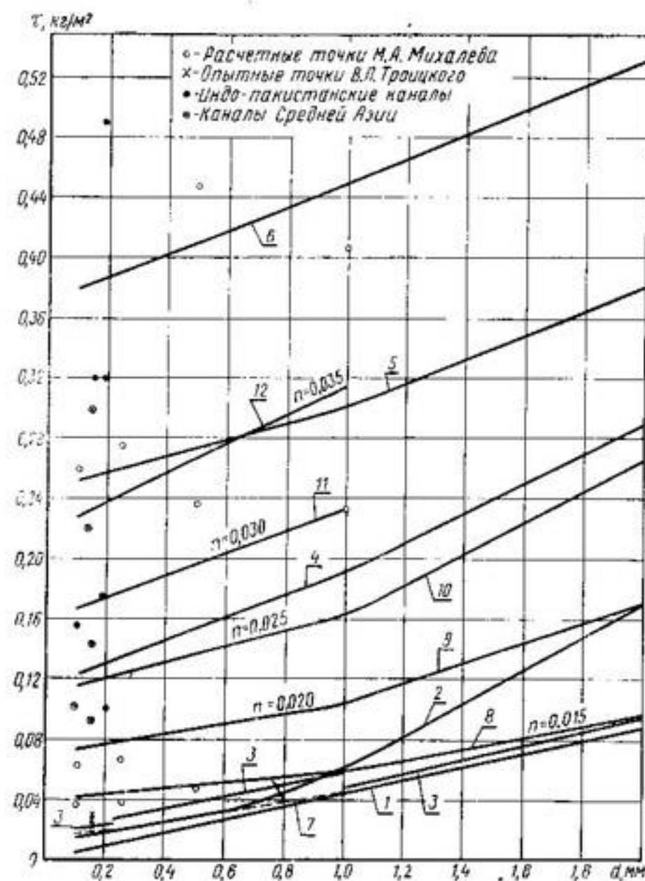
Рис. 53. График зависимости предельных значений касательных напряжений \tau от диаметра d по данным разных авторов: 1 — В. Н. Гончаров; 2 — А. Шильдс; 3 — В. С. Кнороз; 4 — Е. Лейн (чистая вода); 5 — Е. Лейн (небольшое количество коллоидных частиц); 6 — Е. Лейн (значительное количество коллоидных частиц); 7 — М. А. Михалев; 8—12 — В. С. Алтушкин.
