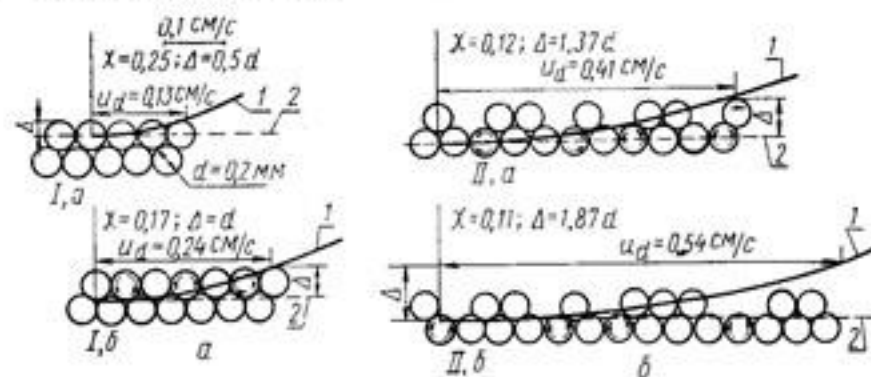
Рис. 44. Схема к определению теоретического дна для начального периода деформаций плоского песчаного дна: 1 — эпюра распределения продольной скорости; 2 — теоретическое дно.
