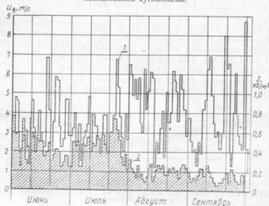
Рис. 7. Совмещение графика скорости ветра U_{\text{в}} (1) и средней мутности потока S (2) в Правоегорлыкском канале (по данным И. Н. Кириенко).
