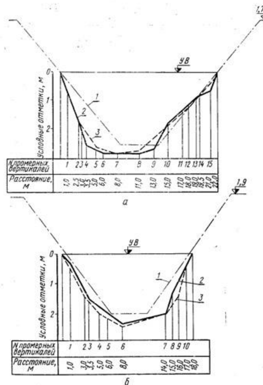
Рис. 22. Поперечные сечения Саратовского канала на 27 км (а) и 28 км (б):
