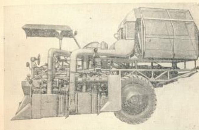
Рис. 21. Хлопкоуборочная машина ХВС-1,2 (общий вид).
