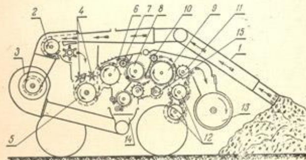
Рис. 32. Хлопководоочиститель УПХ-1,5А (схема работы):
