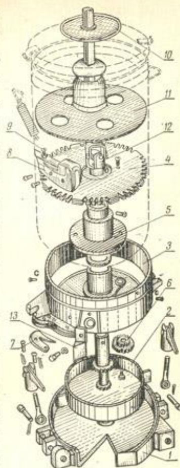
Рис. 10. Высевачный аппарат сеялки СТВХ-4:
