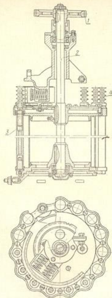
Рис. 22 Шпиндельный барабан хлопкоуборочной машины ХВС-1,2: 1 — приводная шестерня; 2 — вал барабана; 3 — шпиндель; 4 — приводные ролики шпинделя.
