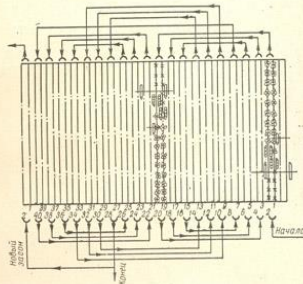
Рис. 28. Схема заездов в рядки машины ХВС-1,2.
