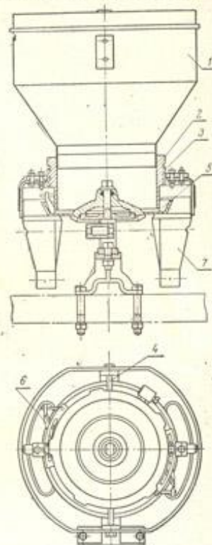
Рис. 16. Культиватор-удобритель НКУ-4-6А:
