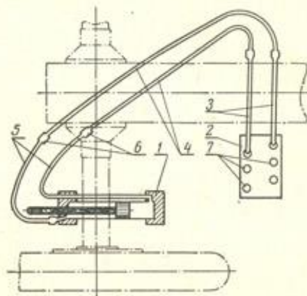
Рис. 19. Схема подключения внешнего гидроцилиндра:
