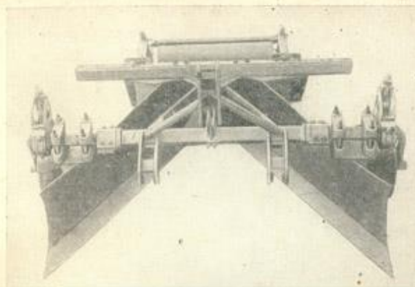
Рис. 33. Канавокопатель-выравниватель универсальный (КЗУ-0,3Б) в варианте валикоделателя, (вид спереди).
