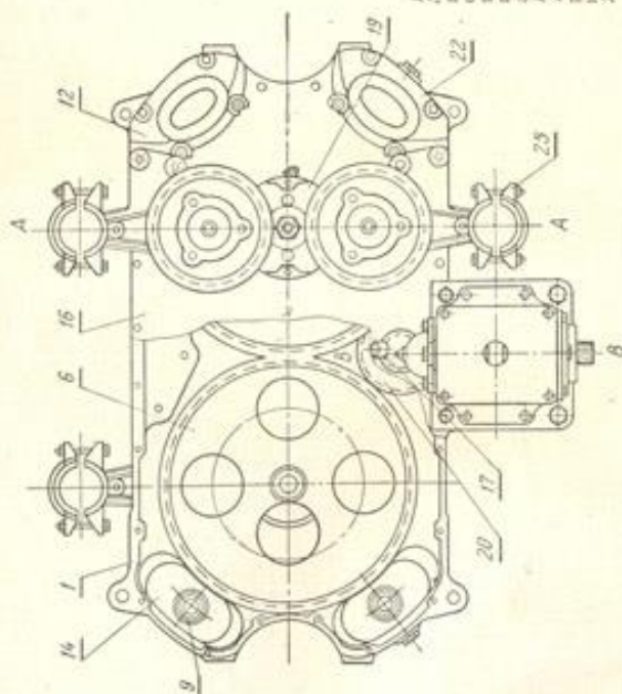
Рис. 25. Распределительная коробка: 1 — корпус коробки; 2 — коническая шестерня Z=19 ; 3 — горизонтальный вал; 4 — вертикальный вал; 5 — шестерня Z=49 ; 6 — большая шестерня Z=108 ; 7 — шестерня Z=17 ; 8 — паразитная шестерня Z=55 ; 9 — шестерня Z=21 ; 10 — поводок барабана верхний; 11 — поводок барабана нижний; 12 — крышка делая; 13 — вал аппарата; 14 — полушарик; 15 — стакан; 16 — крышка; 17 — корпус со штуцером; 18 — корпус редуктора; 19 — крышка подшипника; 20 — шестерня Z=35 ; 21 — это редуктора; 22 — крышка прана; 23 — крышка; 24 — крышка верхняя; 25 — накладка; 26 — валки привода; 27 — крышка подшипника; 28 — крышка лаула; 29 — ось шестерни.
