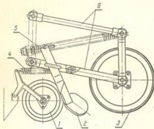
Рис. 12. Заделывающие рабочие органы сеялки СТВХ-4:
