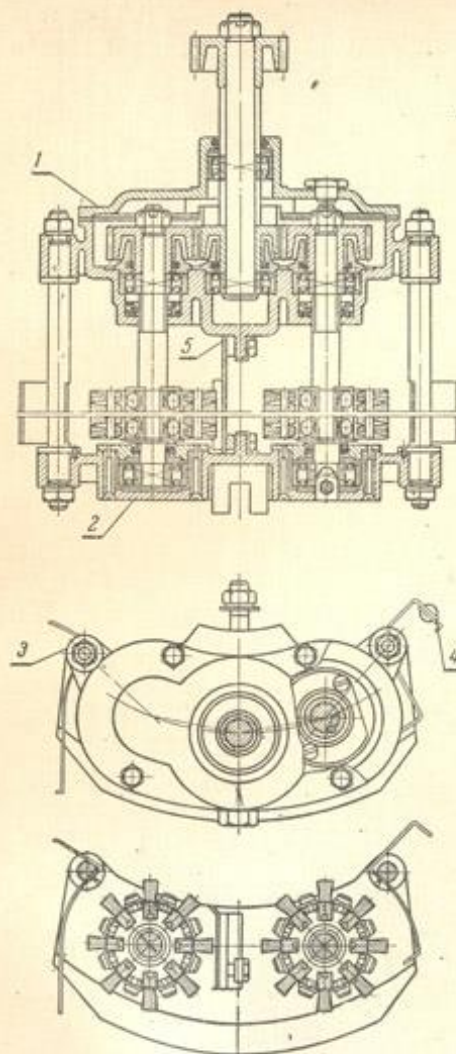
Рис. 24. Щеточный съемник:
