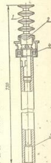
Рис. 23 Шпиндель хлопкоуборочной машины ХВС-1,2:
