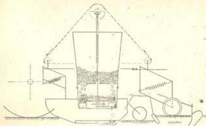
Рис. 11. Схема высева и заделки семян сеялкой СТВХ-4.
