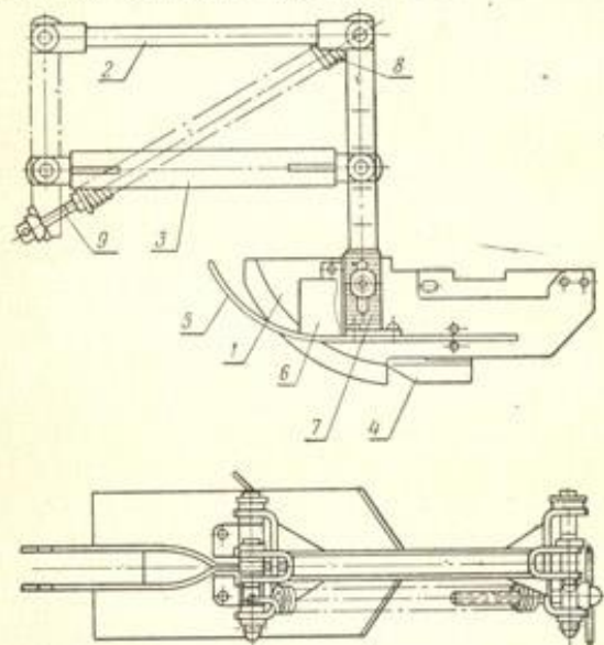
Рис. 9. Сошник сеялки СТВХ-4:
