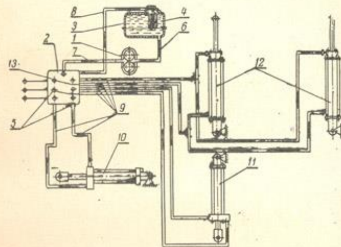
Рис. 27. Гидросистема:
