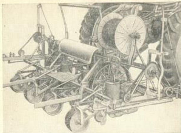
Рис. 8. Сеялка СТВХ-4 (общий вид).
