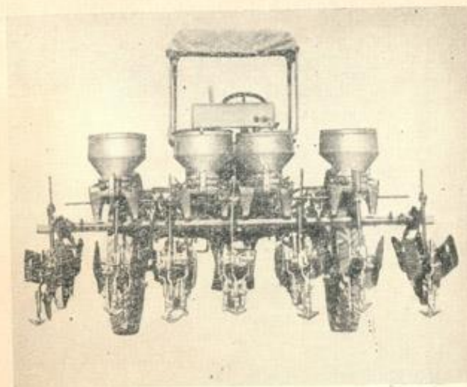
Рис. 15. Культиватор-удобритель НКУ-4-6 (общий вид).
