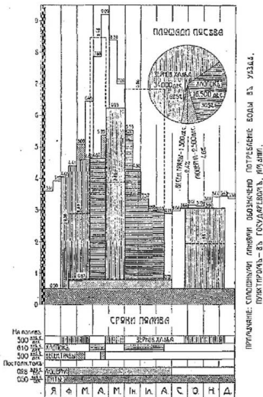
ГРАФИКЪ СРЕДНИХЪ СЕКУНДНЫХЪ ПОЛУМѢСЯЧНЫХЪ РАСХОДОВЪ В. МУРГАЕВЪ И ПОТРЕБЛЕНИЯ ВОДЫ НА ОРОШЕНИЕ 54.300 ДЕС.
