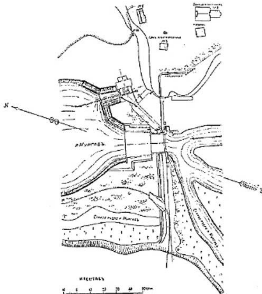
Планъ Гидроузда съ показаніемъ гидроэлектрической станціи
