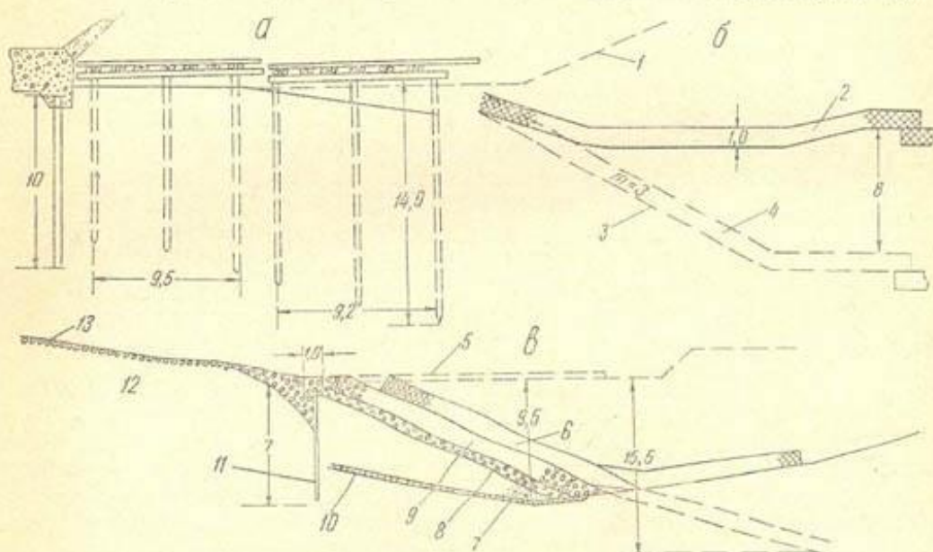
Рис. 42. Крепление нижнего бьефа Кызыл-Ординской плотины.
