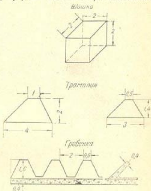
Рис. 27. Типы гасителей четвертой береговой схемы Тахиаташского гидроузла распластанным профилем (размеры в метрах).
