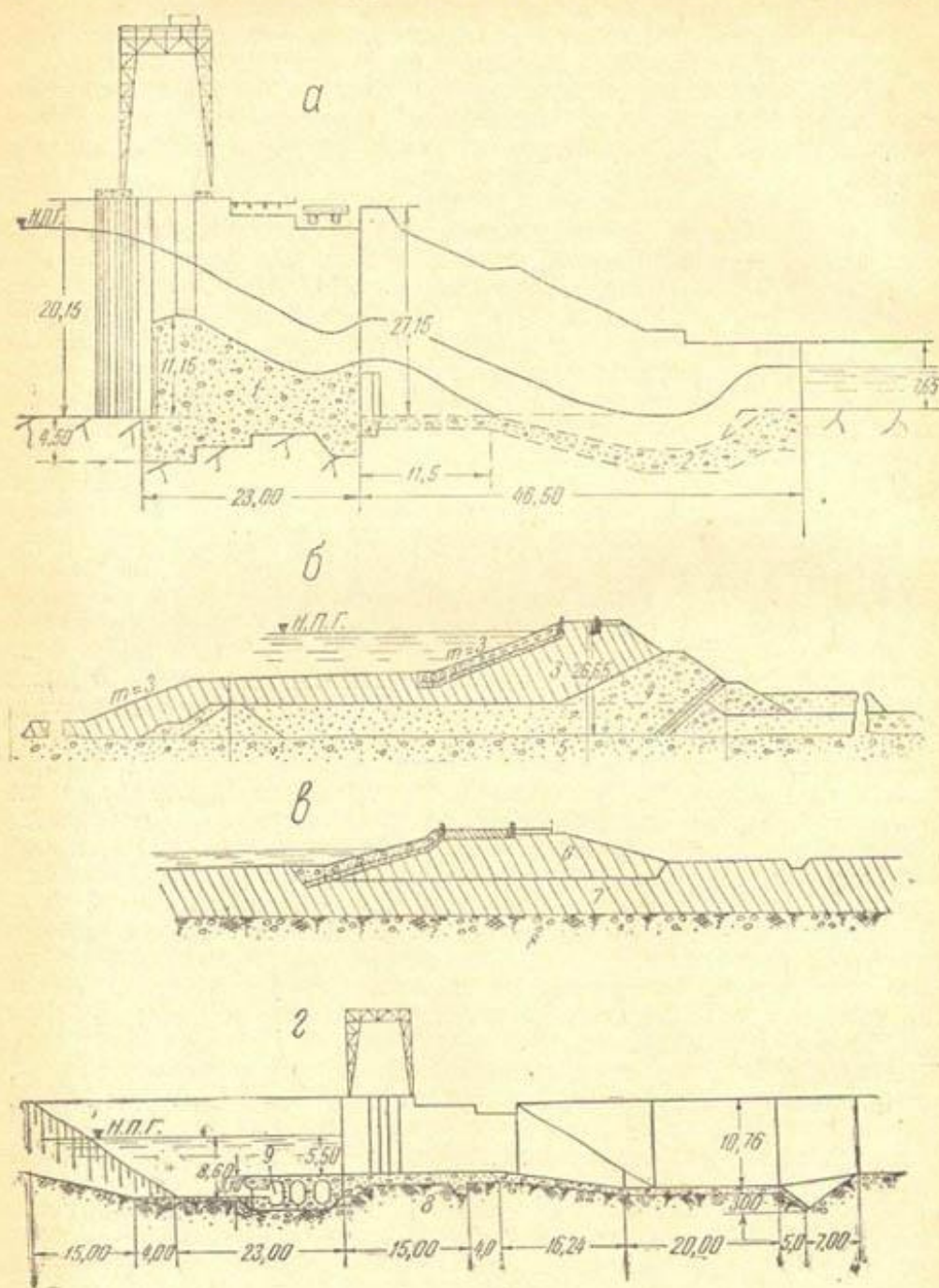
Рис. 36. Разрезы по плотине Фархадской ГЭС:
