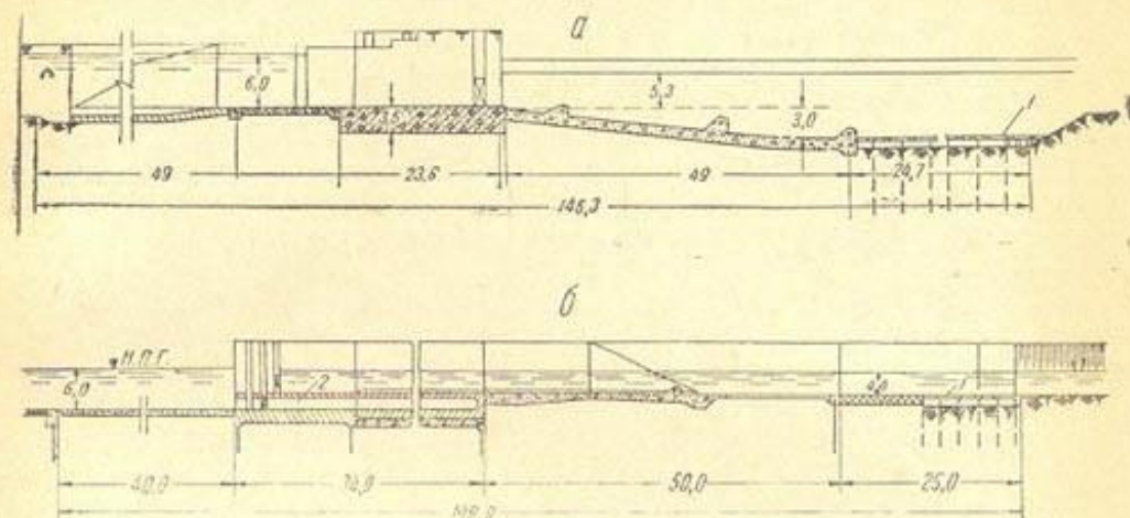
Рис. 41. Продольные разрезы Кызыл-Ординской плотины:
