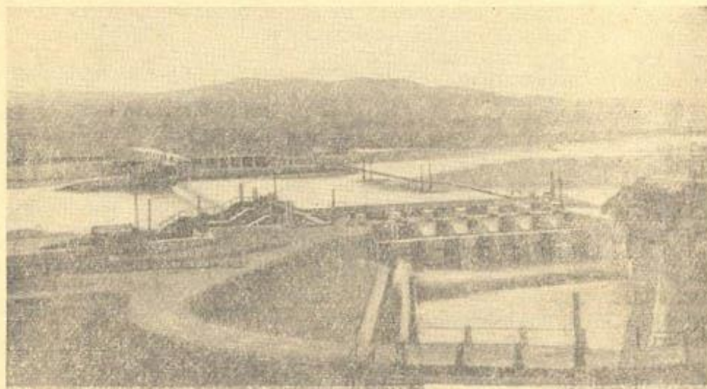
Рис. 7. Первомайская плотина на р. Зарафшан в 1930 г.
