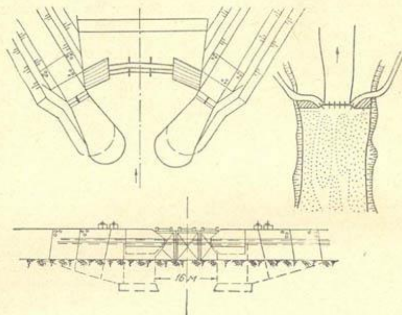
Рис. 48. Схема Караунгурской плотины Артамонова (КиргССР).
