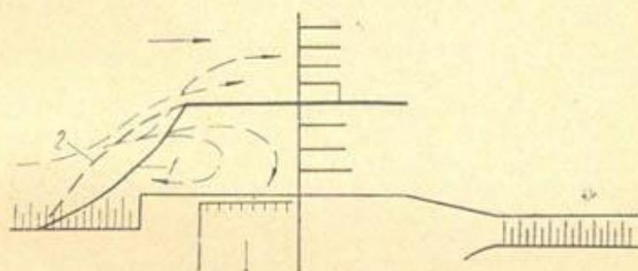
Рис. 58. Два варианта наносостойного порога промывного кармана головного регулятора:
