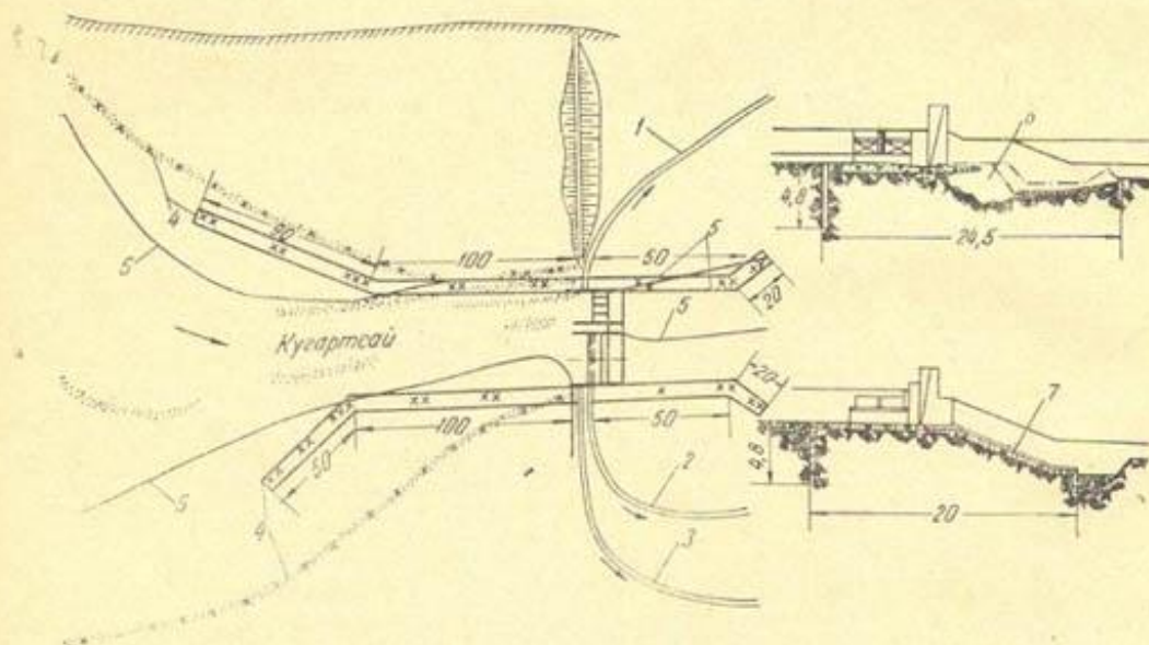
Рис. 4. Схема водозабора на Кугартсае, КиргССР:
