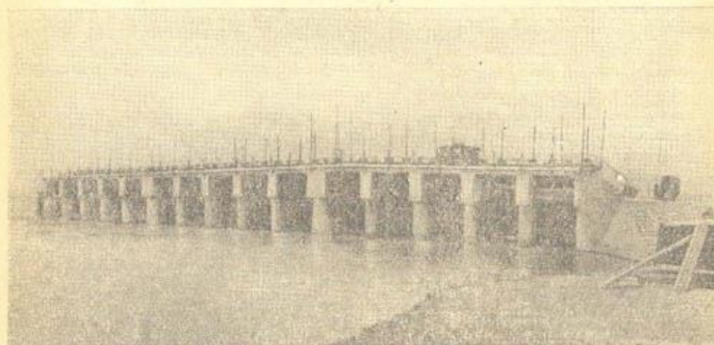
Рис. 29. Головной регулятор Кызкеткен на Амударье у Тахнаташа.
