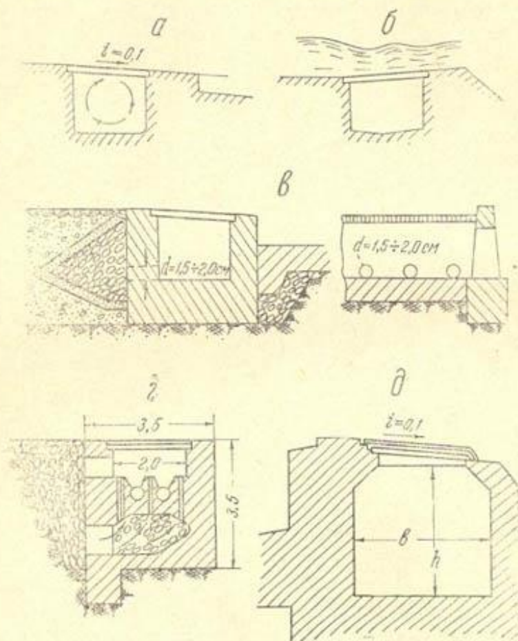
Рис. 52. Развитие конструкций водозахватных и наносоперехватывающих галерей плотины решетчатого типа; варианты а, б, в, г, д (размеры в метрах).
