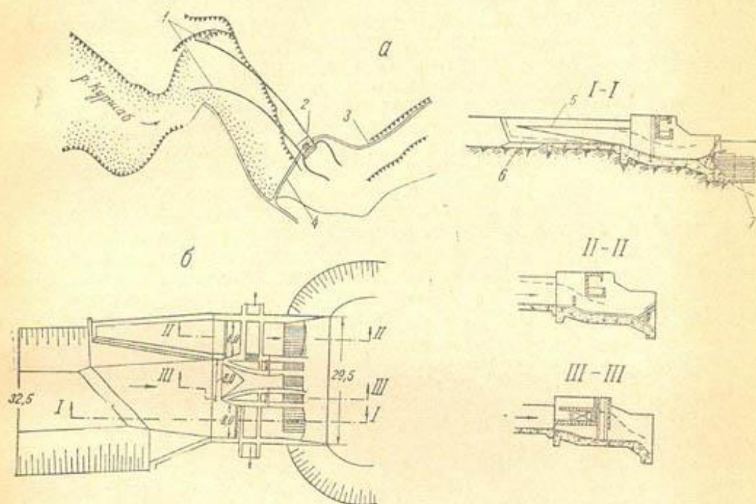
Рис. 39. Схема Куршабской плотины на р. Куршаб:
