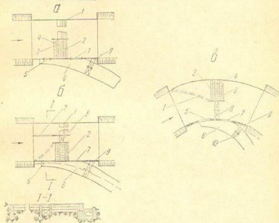
Рис. 51. Компонировка плотин решетчатого водозабора:
