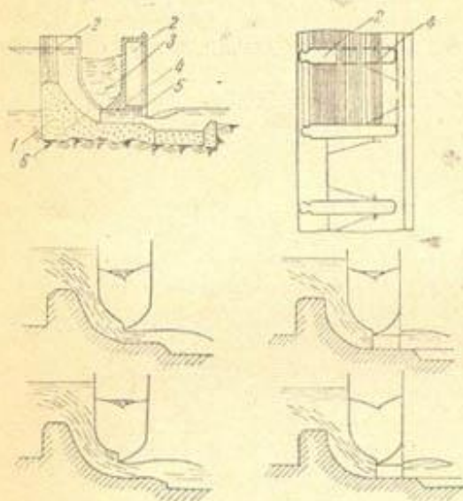
Рис. 56. Гидродинамическая схема водозабора П. Стратоберда:
