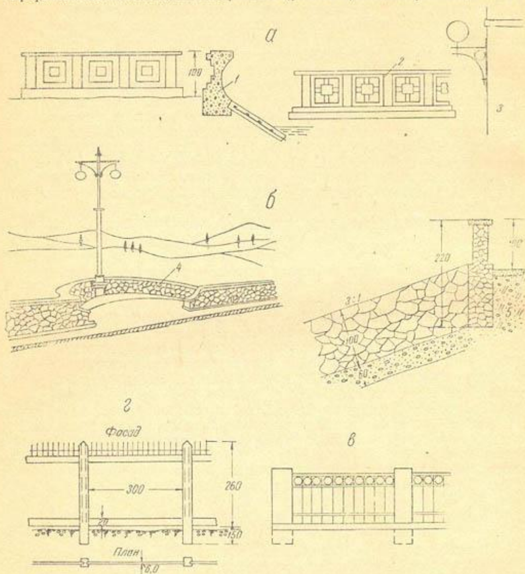
Рис. 63. Архитектурные эскизы некоторых деталей плотин Средней Азии:
