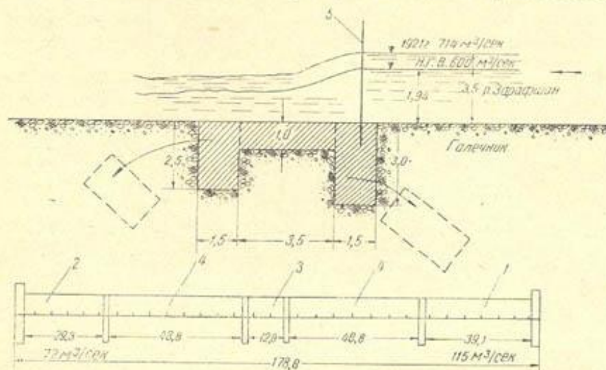
Рис. 2. Вододелитель у местечка Раватходжа на р. Зарафшан: 1—правобережный шлюз-регулятор; 2—левобережный шлюз-регулятор; 3—отверстие плотохода; 4—два щитовых отверстия; 5—стойки-лазы из швеллеров (Размеры в метрах).
