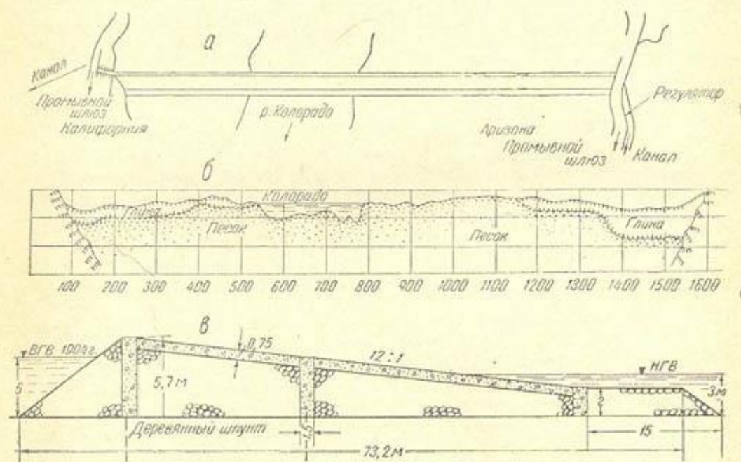
Рис. 30. Плотина Лагуна на р. Колорадо в США:
