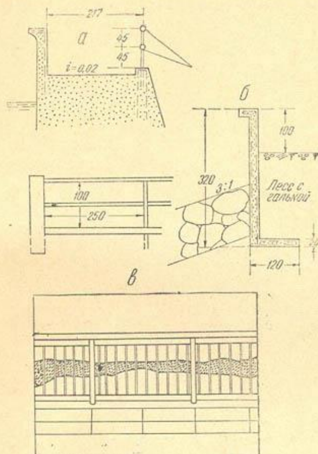
Рис. 64. Архитектурные эскизы некоторых деталей зарубежных плотин:
