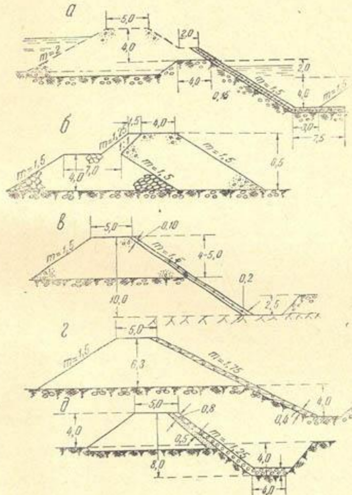
Рис. 60. Поперечные сечения береговых дамб водозаборных плотин:
