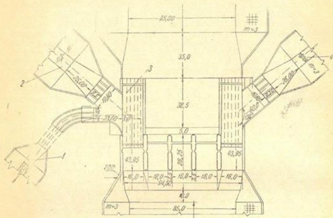
Рис. 43. План Казалинской плотины на Сырдарье по первому варианту 1959 г.: 1—рыбохозяйственный канал; 2—ирригационный канал; 3—промывные галереи; 4—правобережный ирригационно-рыбохозяйственный канал (размеры в метрах).
