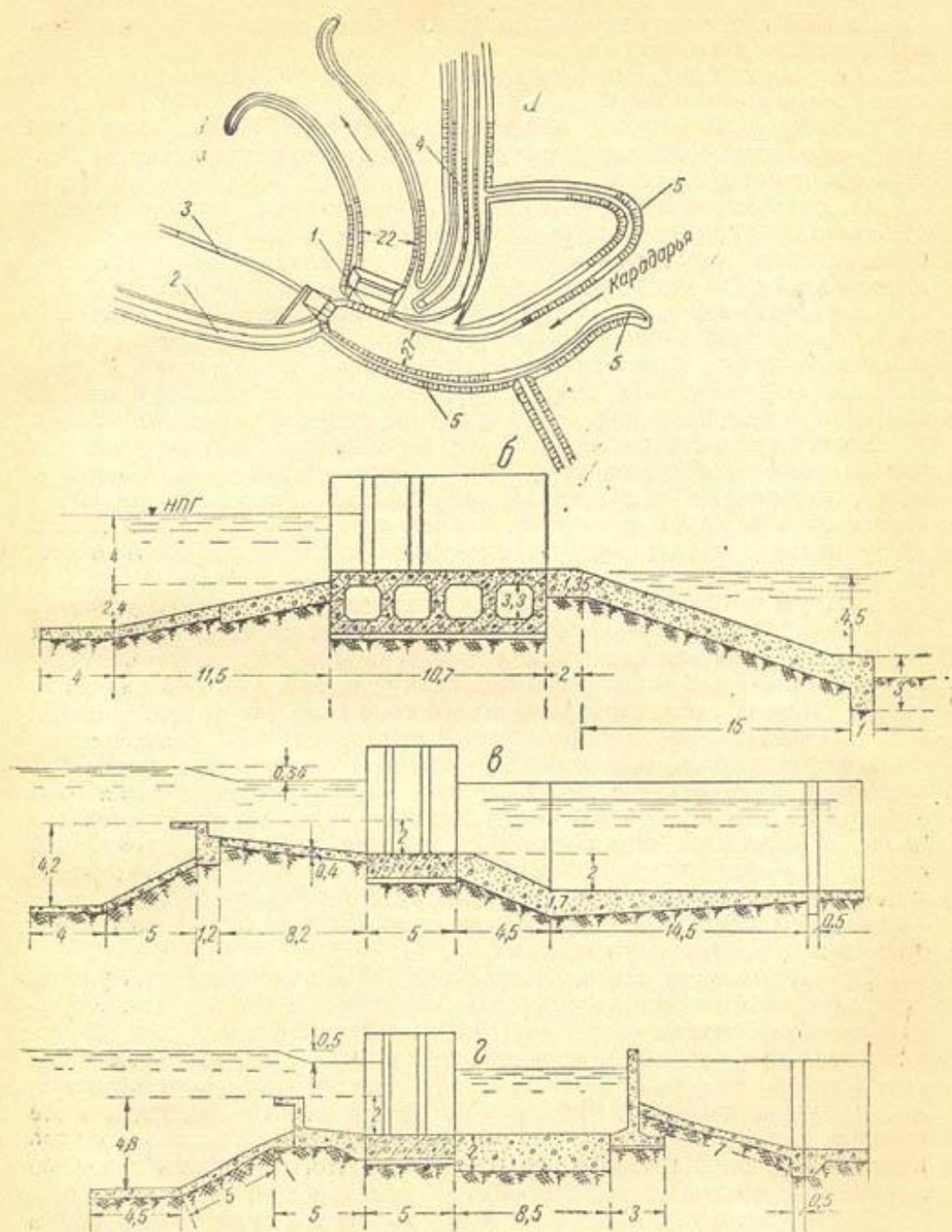
Рис. 21. Схема Дамходжинского гидроузла:
