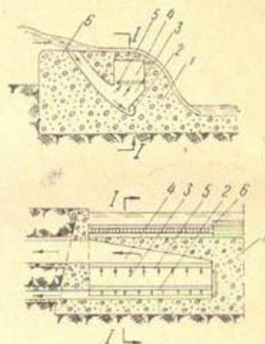
Рис. 57. Схема гидравлического сепаратора Ф. С. Салахова:
