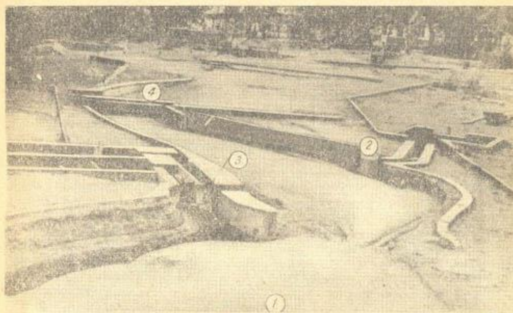
Рис. 28. Модель четвертой береговой схемы двухстороннего последовательного водозабора плотины Тахнаташ после пропуска максимального расхода:
