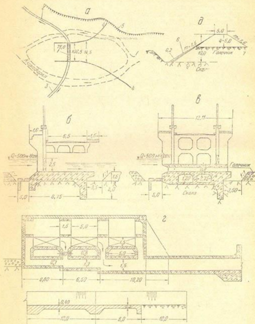
Рис. 47. План и разрезы Тешикташской плотины на Карадарье:
