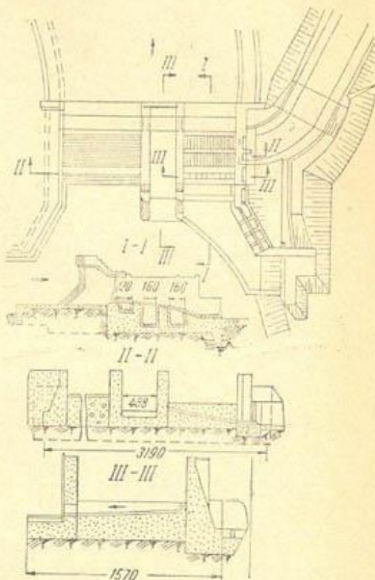
Рис. 54. Верхне-Талгарская плотина решетчатого типа (размеры в сантиметрах).
