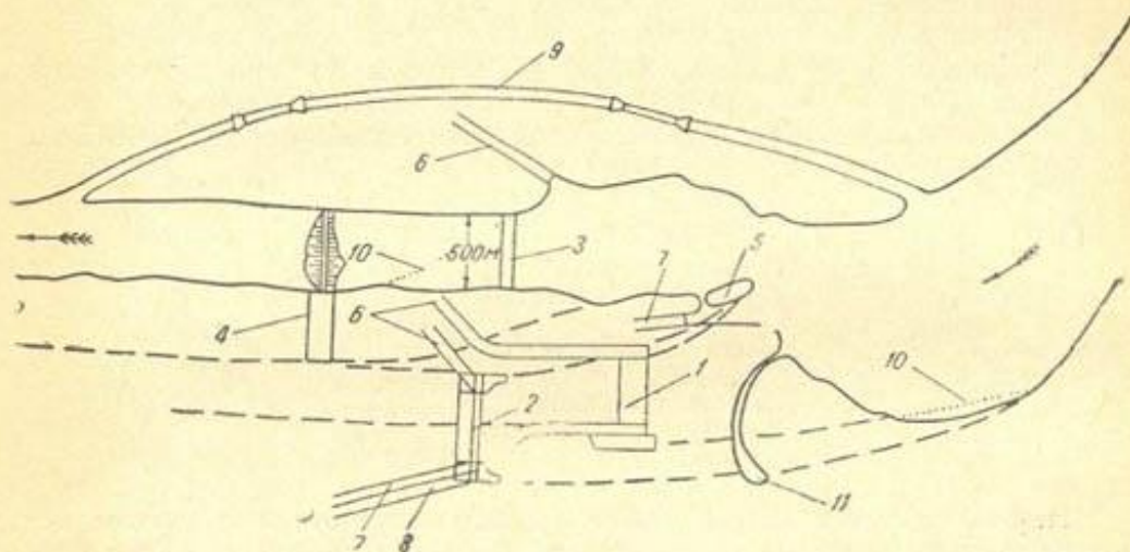
Рис. 24. Схемы водозаборов у мыса Тахиаташ на Амударье.
