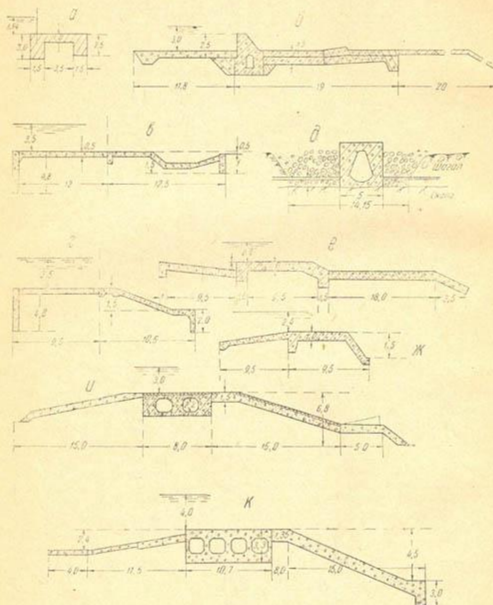
Рис. 59. Флютбеты водозаборных плотин:
