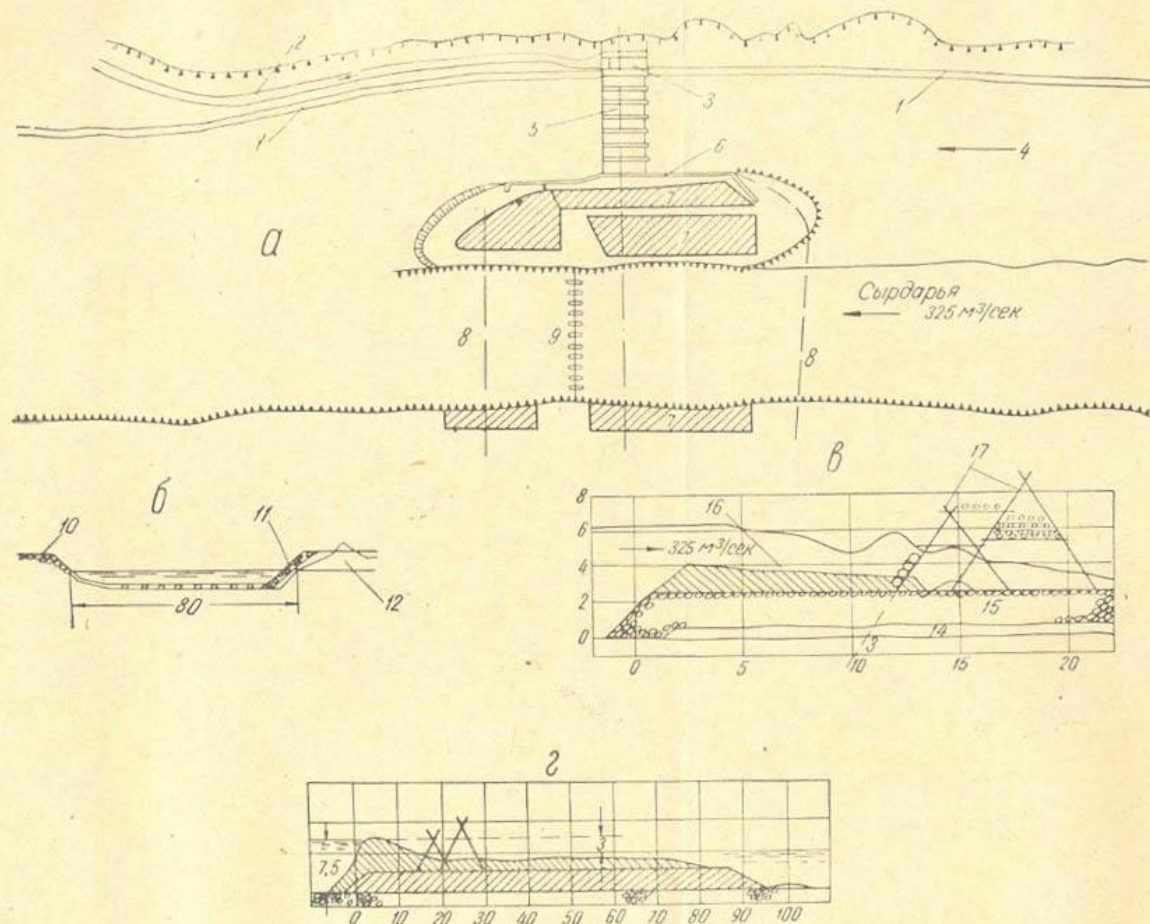
Рис. 37. Перекрытие Сырдарьи на Фархадстрое:
