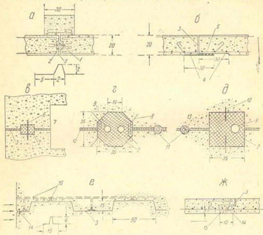
Рис. 61. Осадочные и температурные швы:
