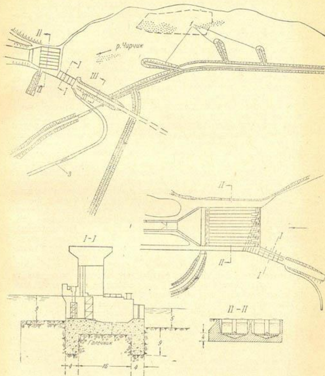
Рис. 35. План и разрезы Газаалкентской плотины на р. Чирчик:
