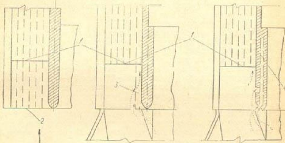
Рис. 45. Схемы конструкций по борьбе с завихрениями на Казалинской плотине, предложенные САНИИРИ:
