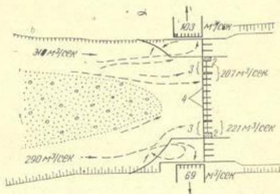
Рис. 8. Восьмой вариант реконструкции Первомайской плотины:
