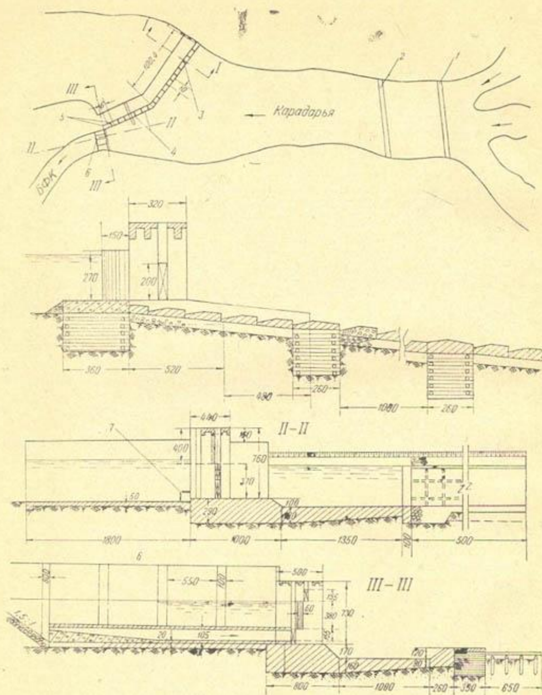
Рис. 16. Детали Куйганьярской плотины после реконструкции в 1957 г.:
