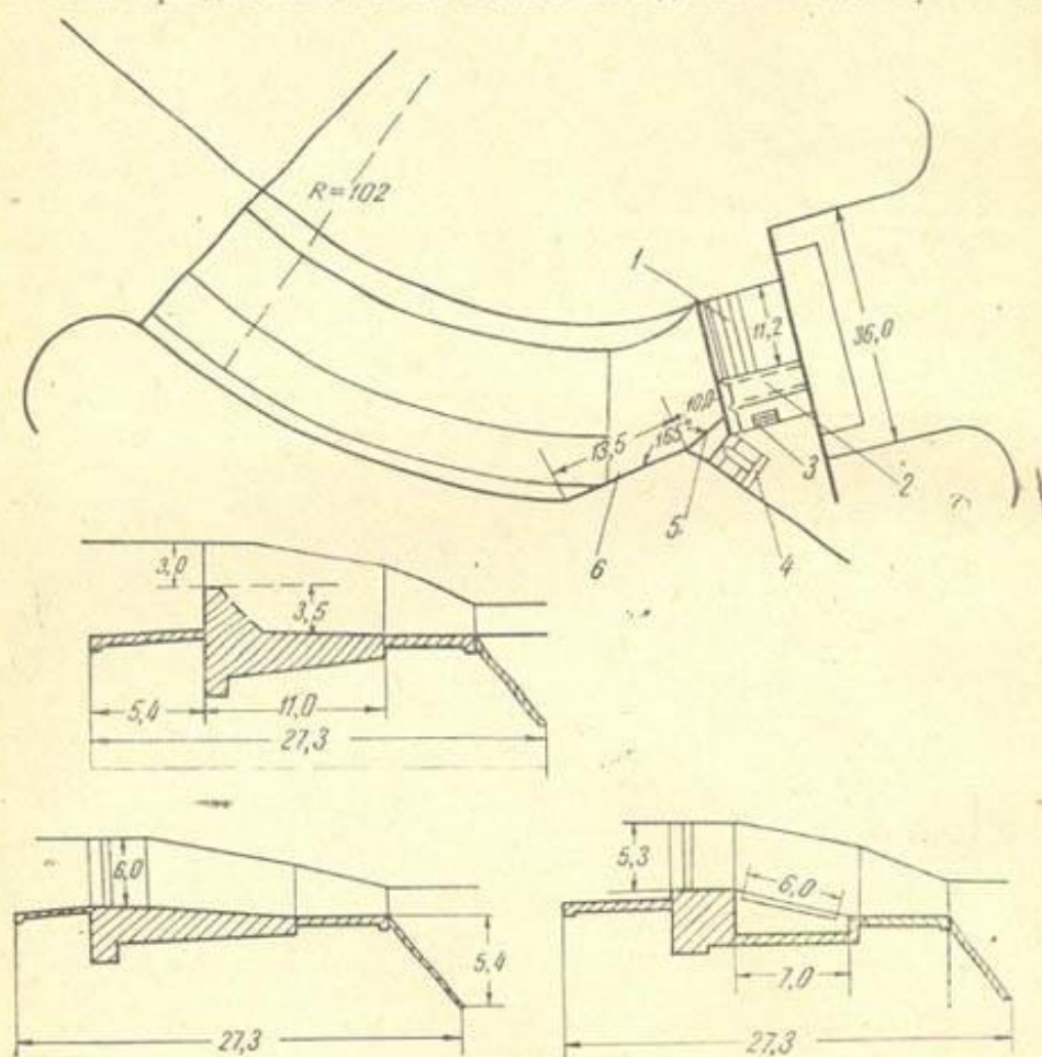
Рис. 55. Водозабор ферганского типа с донной решеткой:
