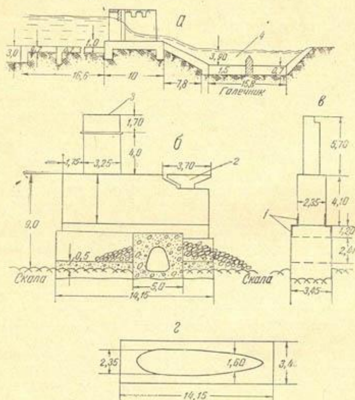
Рис. 11. Конструкции плотины Кампырват:
