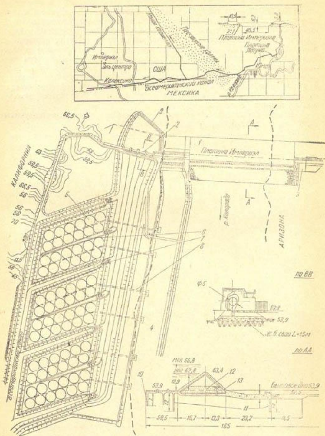
Рис. 31. Головные сооружения Всеамериканского канала США:
