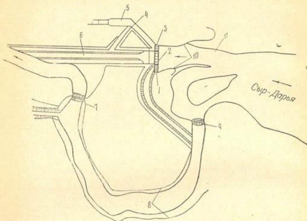
Рис. 40. План расположения Кзыл-Ординского гидроузла на Сырдарье:
