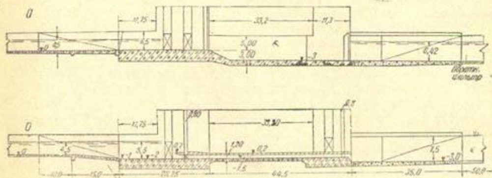
Рис. 44. Продольные разрезы Казалинской плотины на Сырдарье: а—разрез по шлюзовому отверстию плотины; б—разрез по промывному отверстию (размеры в метрах).
