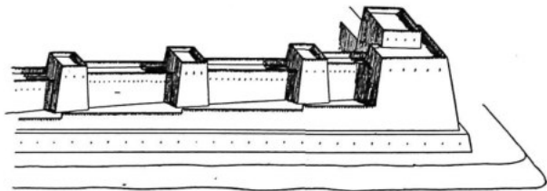
Старая Ниса. Часть стены и пандуса. Реконструкция.
