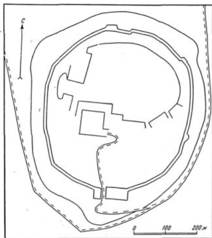
Эрк-кала (архаический Мерв). План.
