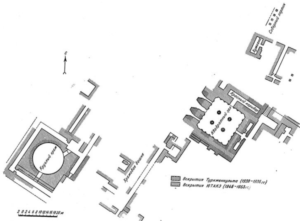
Южный комплекс. План выявленных раскопками строений,
