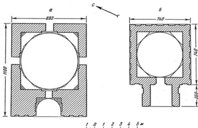
Планы мавзолеев № 2 и № 3.
