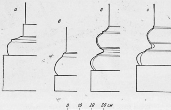
Профили баз из помещений южного комплекса Старой Нисы.
