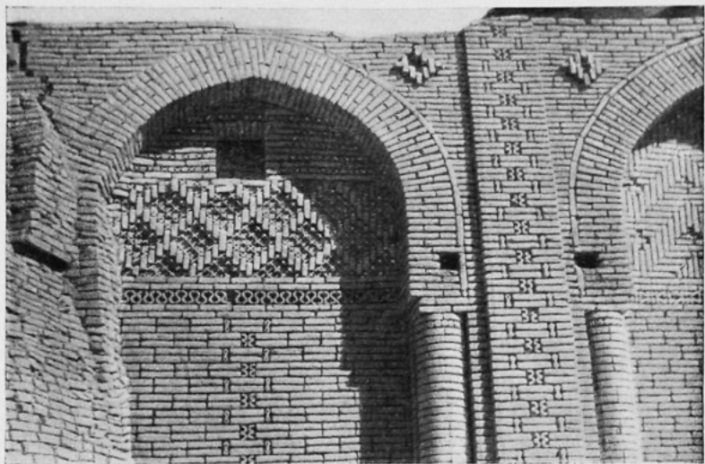
Мечеть Талхатан-баба. Деталь фигурной кладки.
