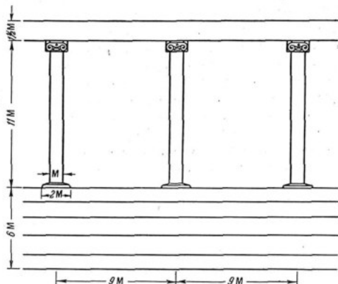
Храм в некрополе Новой Нисы. Пропорции «ордера» Красной стены.
