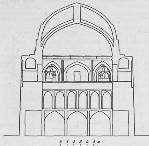
Мавзолей Абу-Саида. Разрез.
