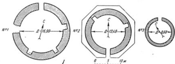
Мерв. Планы снегохранилищ.
