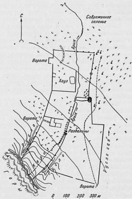
Ферава. План.
