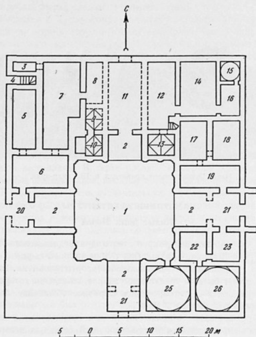
Мерв. Дворец правителя в Шахрияр-арке. План.
