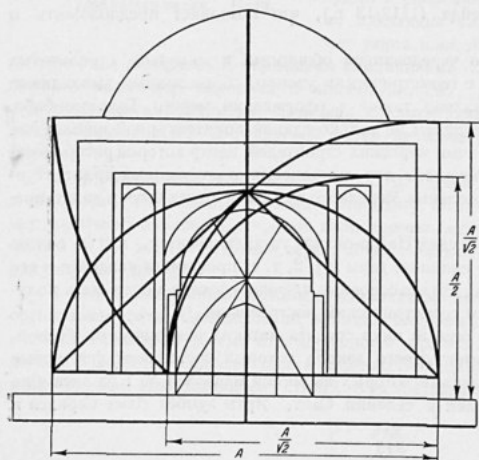
Худай-Назар-овлия. Реконструкция фасада.
