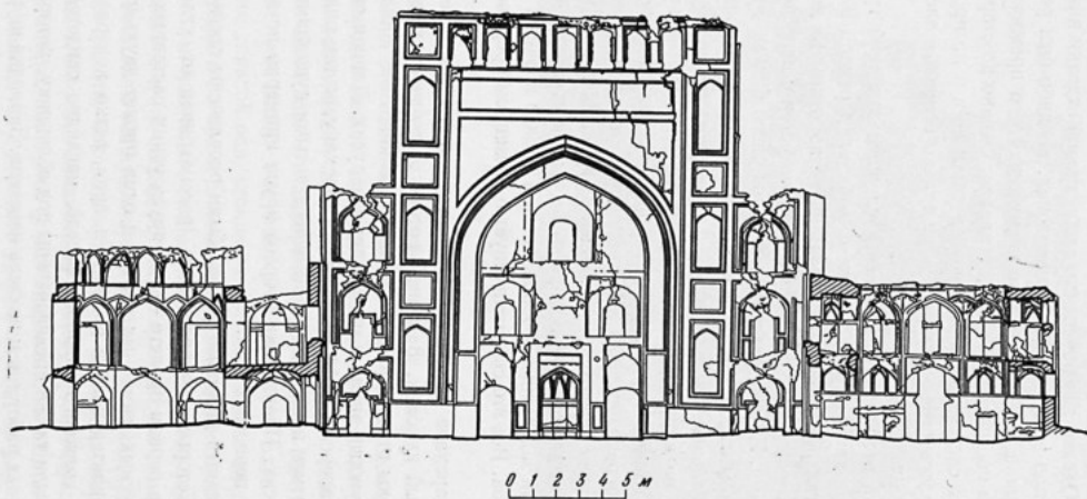
Мечеть Анау. Разрез по дарсханам.
