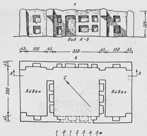
Пештак. Жилой дом. а) Разрез по А—Б; б) план.
