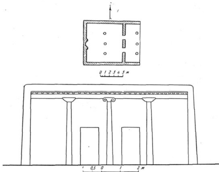
Селение Мурча. План и разрез мечети.
