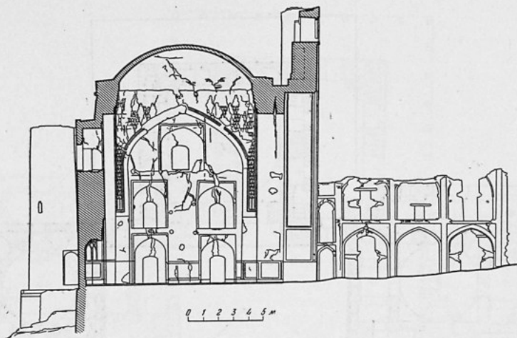
Мечеть Анау. Разрез по главной оси.
