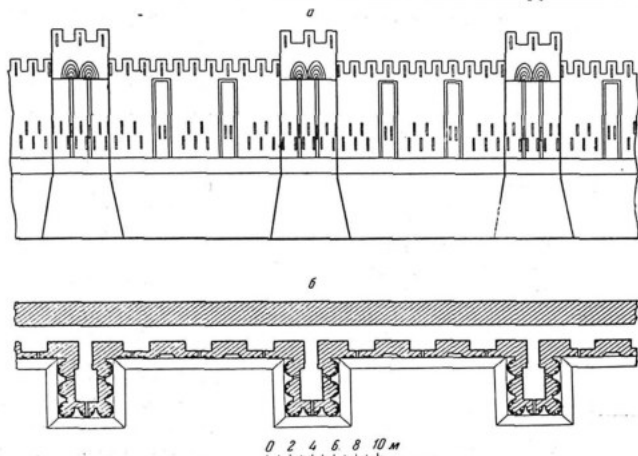
Чильбурдж. Часть стены. Реконструкция.
