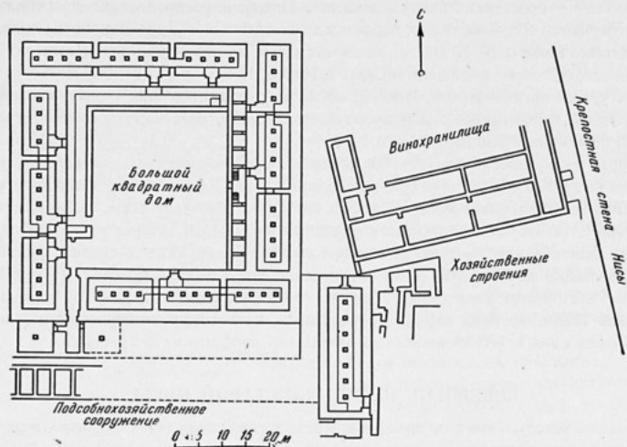
Старая Ниса. План вскрытых строений северного комплекса.
