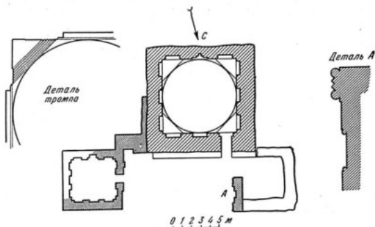
План мазара Шир-Кабир.
