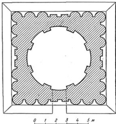
Жилая башня при доме на городище Дурнали. План.
