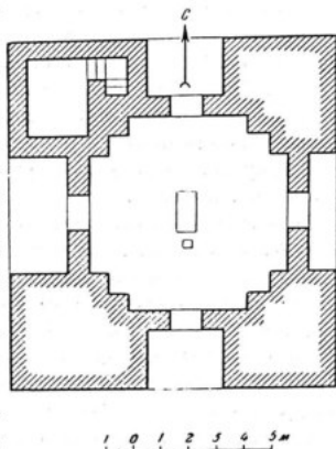
Мазар на кладбище Кумбетли-яйла. План.
