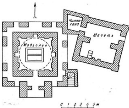
Мазар Шейх-Касим. План.
