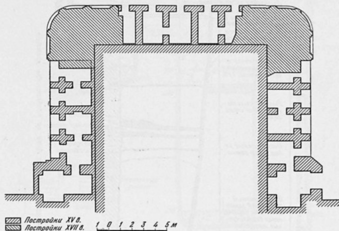
Мечеть Анау. План цокольного этажа. Реконструкция.
