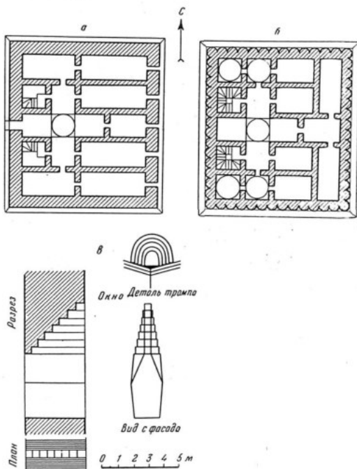
Акули-кошук. Планы и конструктивные детали.
