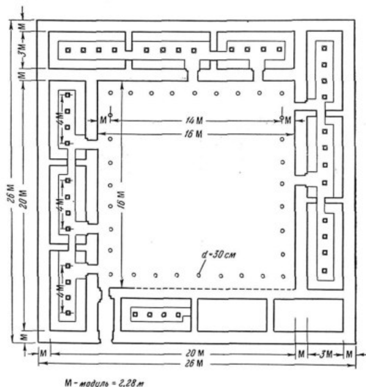
Квадратный дом. Анализ пропорций плана (первый строительный период).
