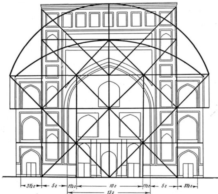
Мечеть Анау. Пропорции фасада.
