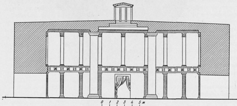
Квадратный зал (первый строительный период). Разрез. Реконструкция.
