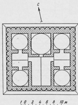
Сулу-кошук. План II этажа.
