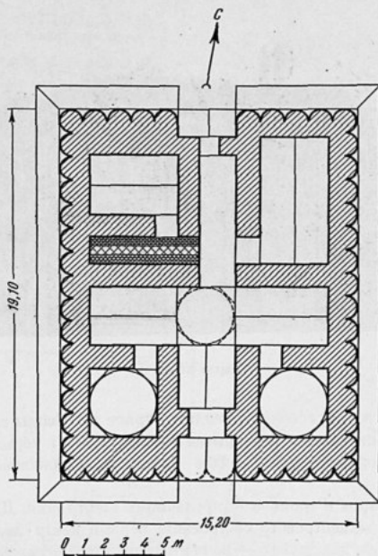
Харам-кёшк. План.
