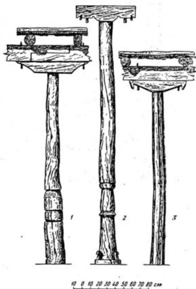
Типы колонн.
