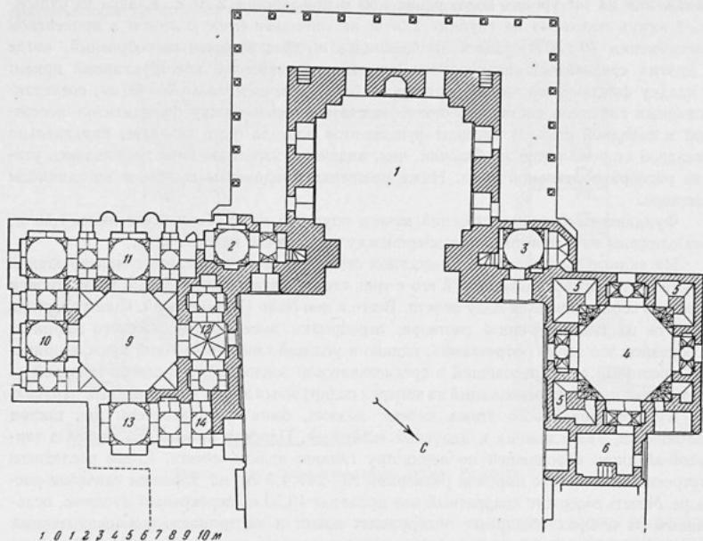
Мечеть Анау. План I этажа. Реконструкция.
