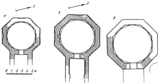
Планы мавзолеев.
