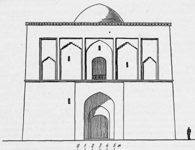
Дом к западу от Султан-калы. Реконструкция фасада.
