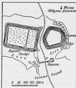
План Хосров-калы.
