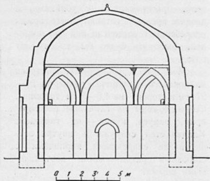
Мавзолей Аламбердара. Разрез.
