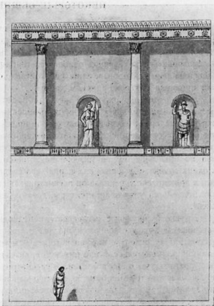
Круглый храм. Ордер. Реконструкция.
