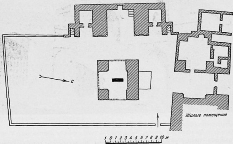
Мечеть Ходжа Юсуфа Хамадани. План строений.
