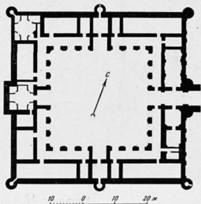
Караван-сарай Дая-Хатын. План.
