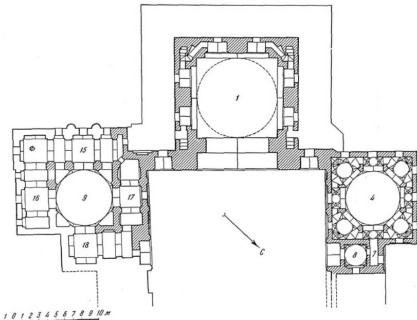
Мечеть Анау. План II этажа. Реконструкция.
