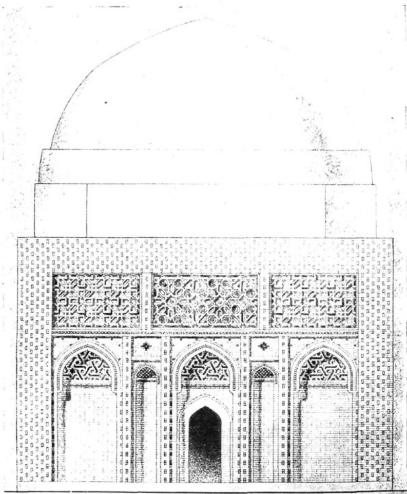
Мавзолей Мухаммеда ибн-Зейда. Реконструкция фасада.
