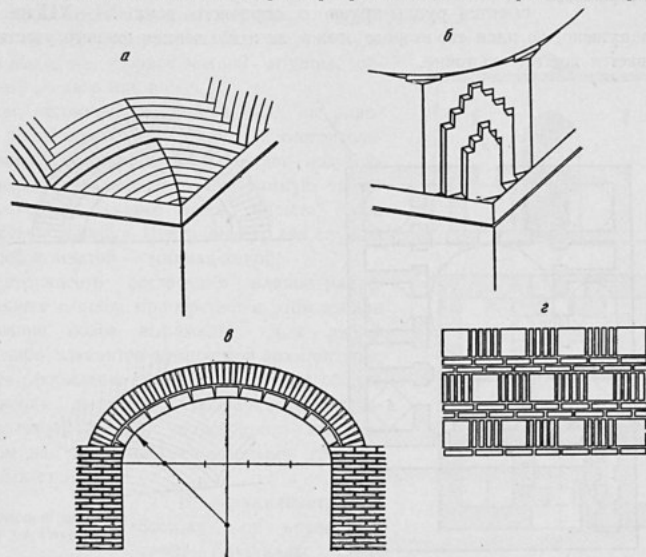
Мерв. Дворец правителя в Шахрияр-арке. Конструктивные детали.
