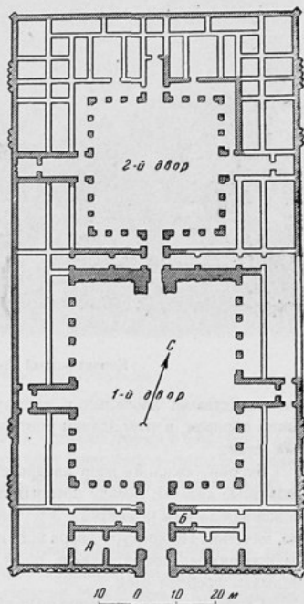
Караван-сарай Акча-кала. План.
