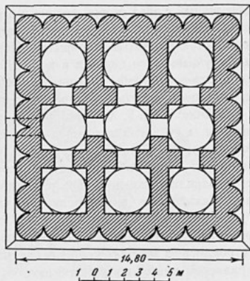
Ат-Такмаладж. План.
