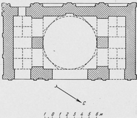
Мечеть Талхатан-баба. План.
