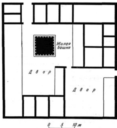
Мунон-тепе. План жилого дома.
