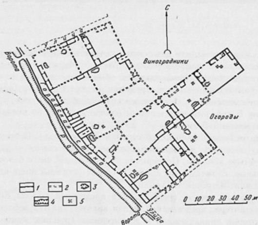
Пештак. Жилой квартал. План.
