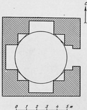
Мавзолей Кыз-биби. План.
