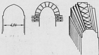
Большая Нагим-кала. Типы арок и перекрытие над окном.
