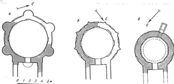
Планы мавзолеев.
