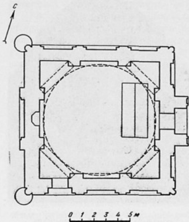
Астана-баба. Мавзолей Аламбердара. План.
