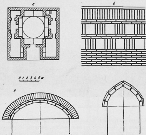
Городище ал-Аскер. План жилого дома XI—XII вв. и конструктивные детали караван-сарая.
