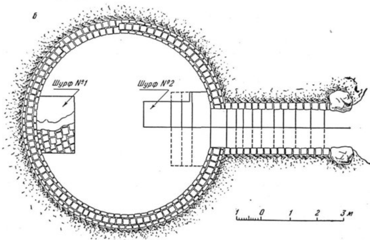
Сардоба в Анау.
