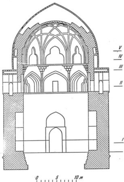
Мавзолей Санджара. Разрез (римскими цифрами обозначены уровни, показанные в плане).
