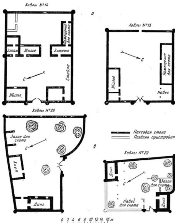
Чарджоуская область. Планы усадеб.
