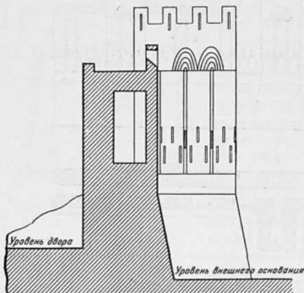
Чильбурдж. Разрез стены. Реконструкция.
