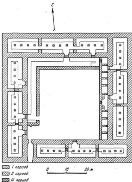
Квадратный дом. План с показанием последовательных изменений.
