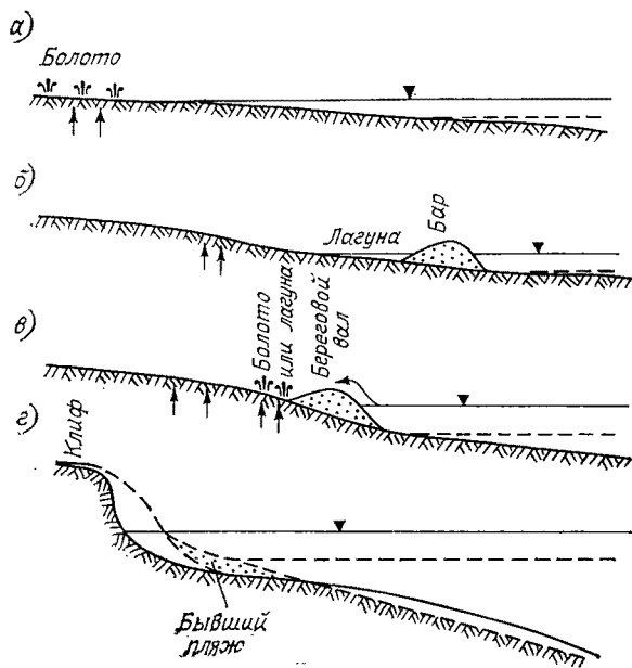
Рис. 22. Схема трангрессивного развития берега в зависимости от уклонов береговой зоны [180].
