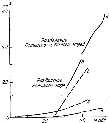
Рис. 12. Зависимость уровня равновесия различных частей Аральского моря от объема водного стока [321].
