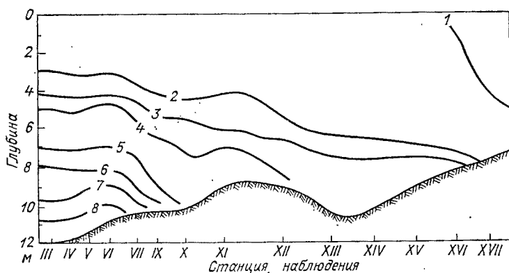
Рис. 30. Вертикальное распределение хлорид-иона (‰) по продольному профилю Днепроовско-Бугского лимана в августе 1983 г. [142].
