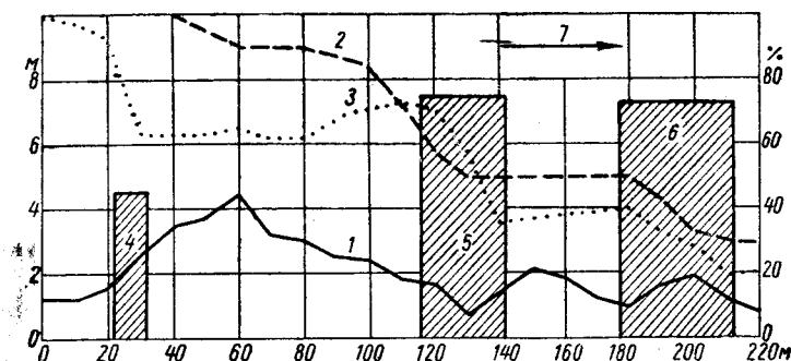
Рис. 20. Высота снега (м) и скорость ветра (в процентах от полевой) на опытном участке № 1 снегозащитных лесонасаждений Томской ж. д. в 1952/53 г., по данным А. А. Комарова (19546). 1 — высота снега, 2 — скорость ветра на высоте 1 м при наличии снежного вала, 3 — то же при отсутствии вала, 4, 5 и 6 — лесные полосы с полнотой насаждения соответственно 50—55, 45—50 и 70—75, 7 — направление ветра.
