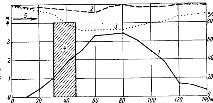
Рис. 19. Высота отложения снега (м) и скорость ветра (в процентах от полевой) на различных расстояниях от одиночной лесной полосы № 1 в 1950/51 г., по данным А. А. Комарова (19546). 1 — высота снега, 2 — скорость ветра на высоте 1 м при наличии снежного вала, 3 — то же при отсутствии вала, 4 — лесная полоса с полнотой насаждения 0,55, 5 — направление ветра.
