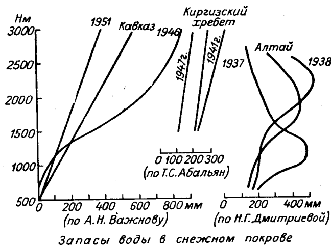
Рис. 25. Кривые изменения снежных запасов по высоте H , близкие к средним многолетним и за отдельные характерные годы для Кавказа, Киргизского хребта и Алтая.
