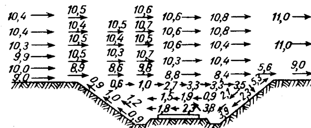
Рис. 7. Спектр скоростей воздушного потока в выемке в м/сек.
