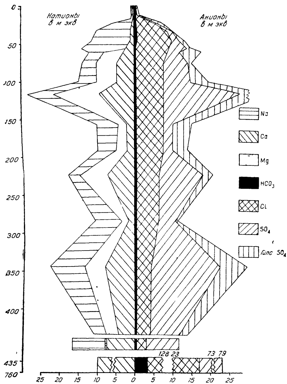
Фиг. 14 Сочетан профиль остаточного олончающего солонца, II терраса р. Мисли Узень Разрез № 5
