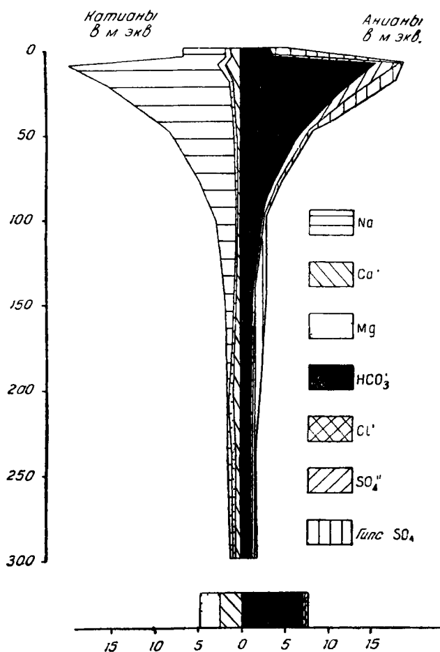
Фиг. 12. Солевой профиль седового солонца-солончака; III терраса р. Самарки. Разрез № 23
