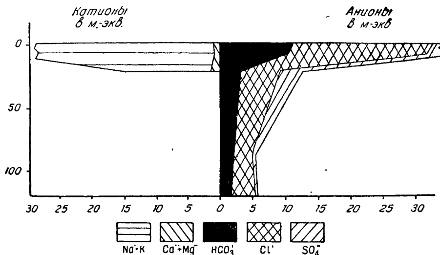
Фиг. 5. Солевой профиль содового солончака Араздаянской степи
