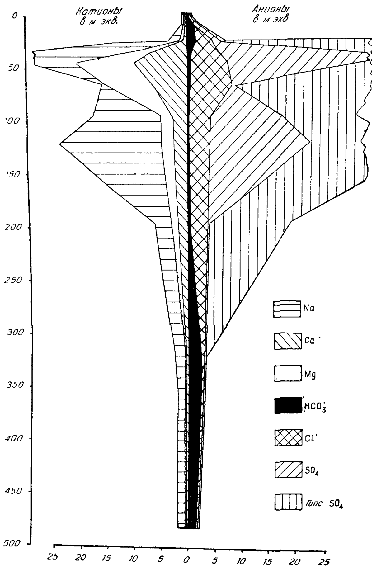
Фиг. 13. Солевой профиль остаточносолончаковатого солонца; II терраса р. Торгун. Разрез № 7
