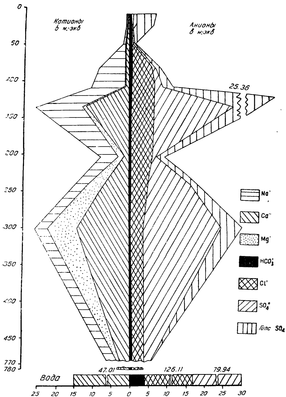
Фиг. 16. Солевой профиль острепленного солонца; II терраса р. Малый Узень. Алексашкино. Разрез № 6
