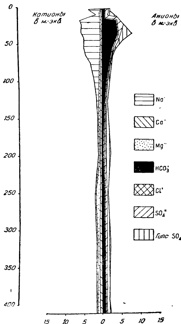
Фиг. 11. Солевой профиль содового солонца; III терраса р. Самарки. Разреза № 43
