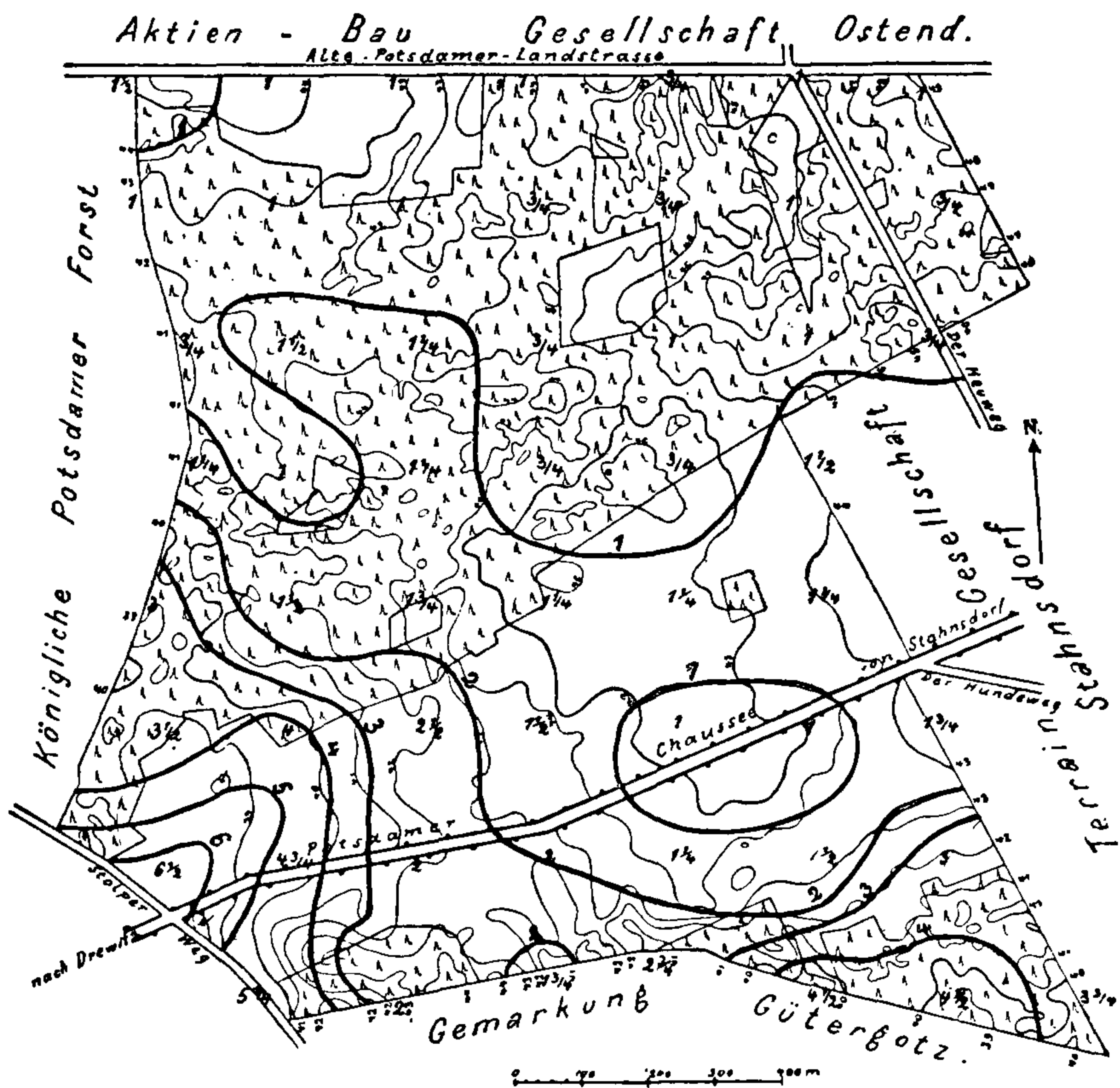
Фиг. 58. Температурныя колебанія грунтовой воды въ области Штансдорфскаго центрального кладбища, представленныя линіями одинаковыхъ температурныхъ разностей. Масштабъ 1:15,000.
