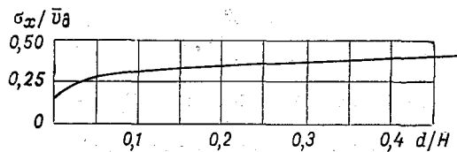
Рис. 33. График \frac{\sigma_x}{v_d} (d/H) .
