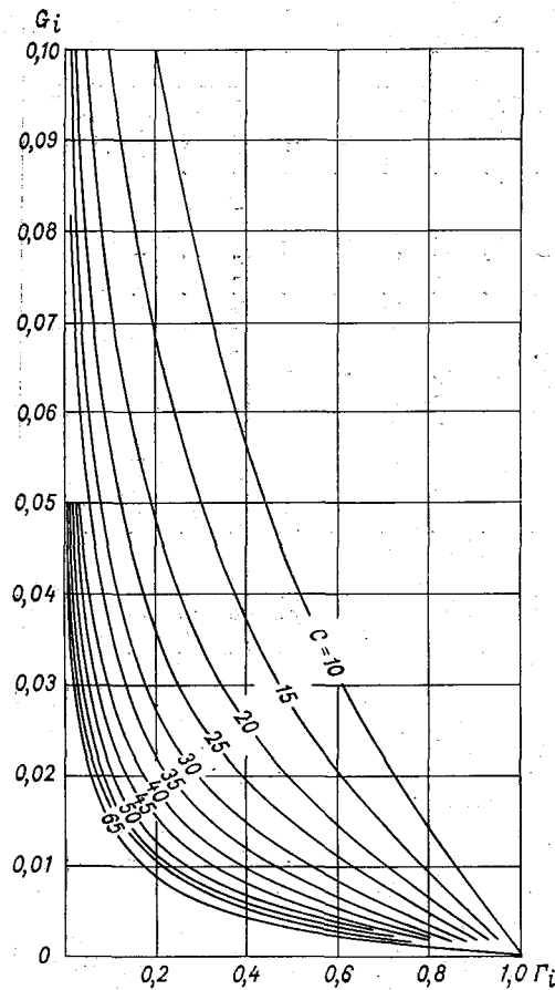
Рис. 27. График функции \Gamma_i(G_i, C) .
