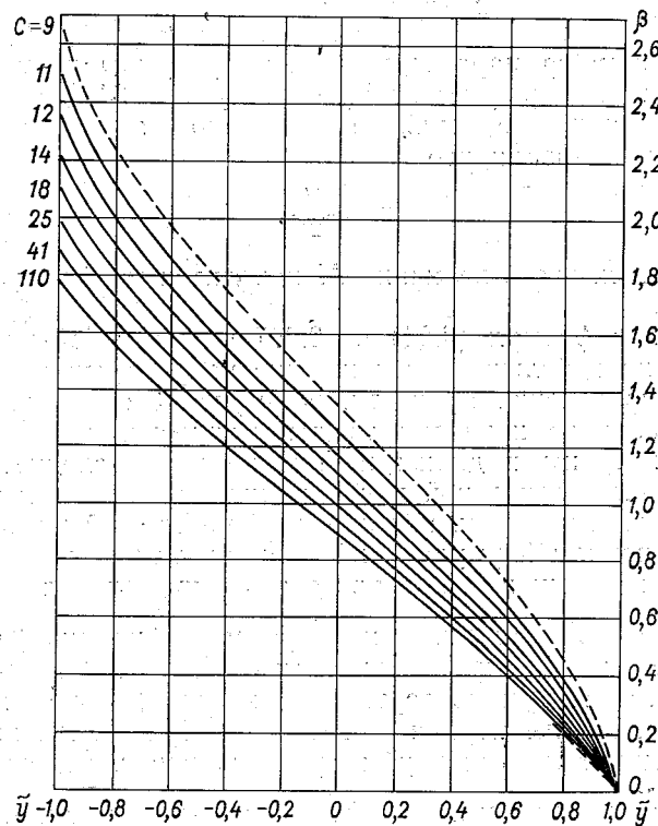
Рис. 20. Графики функции \beta(\tilde{y}) для расчета распределения мутности по вертикали открытого потока ( 0 < \tilde{y} < 1 ) и по вертикальному диаметру трубы ( -1 < \tilde{y} < 1 ).
