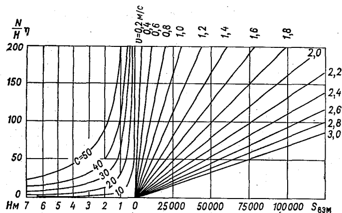
Рис. 29. Номограмма для вычисления S_{\text{взм}} .
