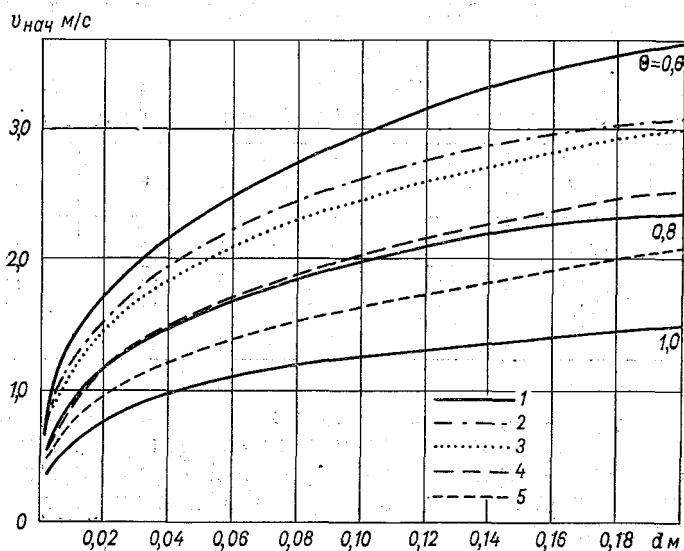
Рис. 8. Зависимость v_{\text{нач}} от размера частиц d и их формы \Theta .
