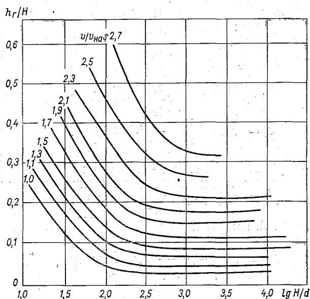
Рис. 15. Зависимость относительной высоты гряды h_r/H от безразмерных величин v/v_{H0} и H/d [46].
