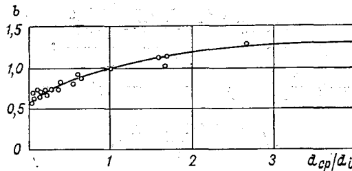
Рис. 32. График b(d_{\text{ср}}/d_i) .
