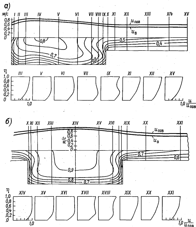
Рис. 10.14. Изотакхи в прямоугольном русле с односторонней (а) и двухсторонней (б) поймами.
