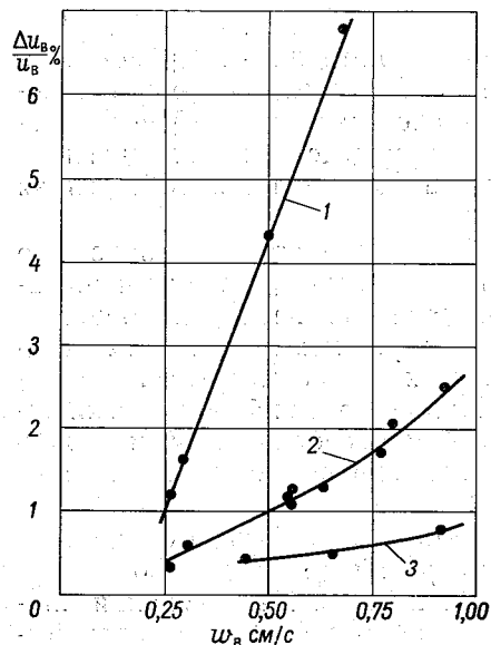
Рис. 6.4. Зависимость относительной погрешности \frac{\Delta u_B}{u_B} определения средней скорости на вертикали u_B интеграционным способом от величины скорости подъема w_B датчика скорости.
