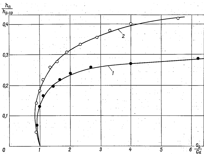
Рис. 11.8. Связь относительного расхода донных наносов \frac{G_p}{G_b} с относительной глубиной в пойме \frac{h_p}{h_{p.c.p}} 1 — первая модель, 2 — вторая модель.
