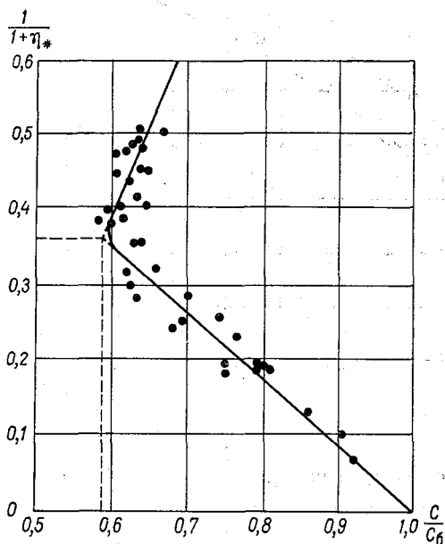
Рис. 10.16. Зависимость относительного коэффициента Шези \frac{C_p}{C_6} от \frac{1}{1+\eta_*} , по данным ВНИИГиМ.
