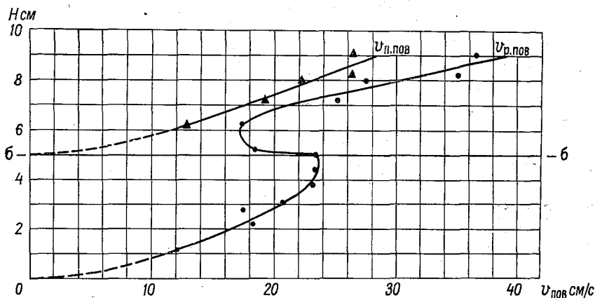
Рис. 10.6. Зависимость средней поверхностной скорости в основном русле v_{р. пов} и средней поверхностной скорости в пойме v_{п. пов} от уровня воды, по опытам (1947 г.) на русловой площадке.
