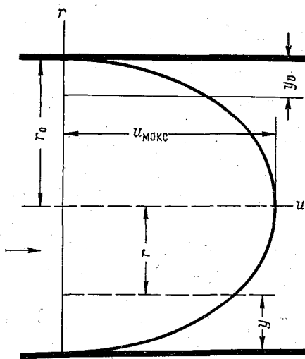
Рис. 2.5. Профиль скоростей напорного потока.
