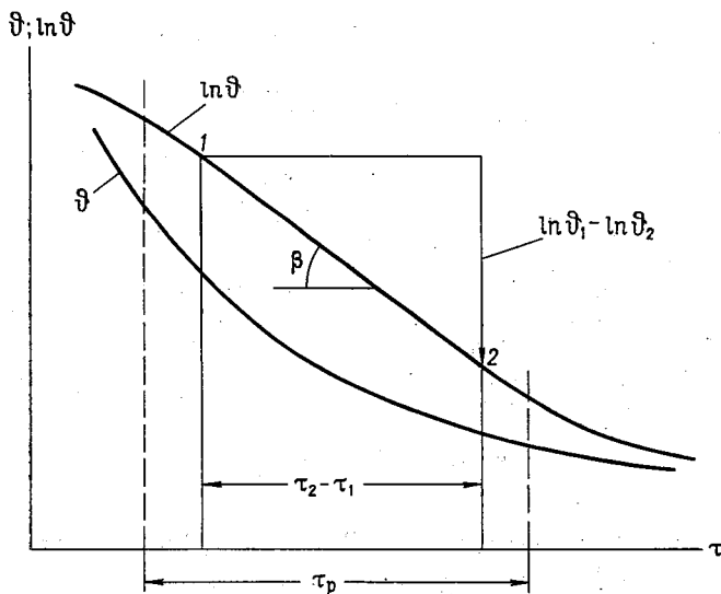
Рис. 6.8. График функции \vartheta = \vartheta(\tau) в обычных и полулогарифмических координатах.
