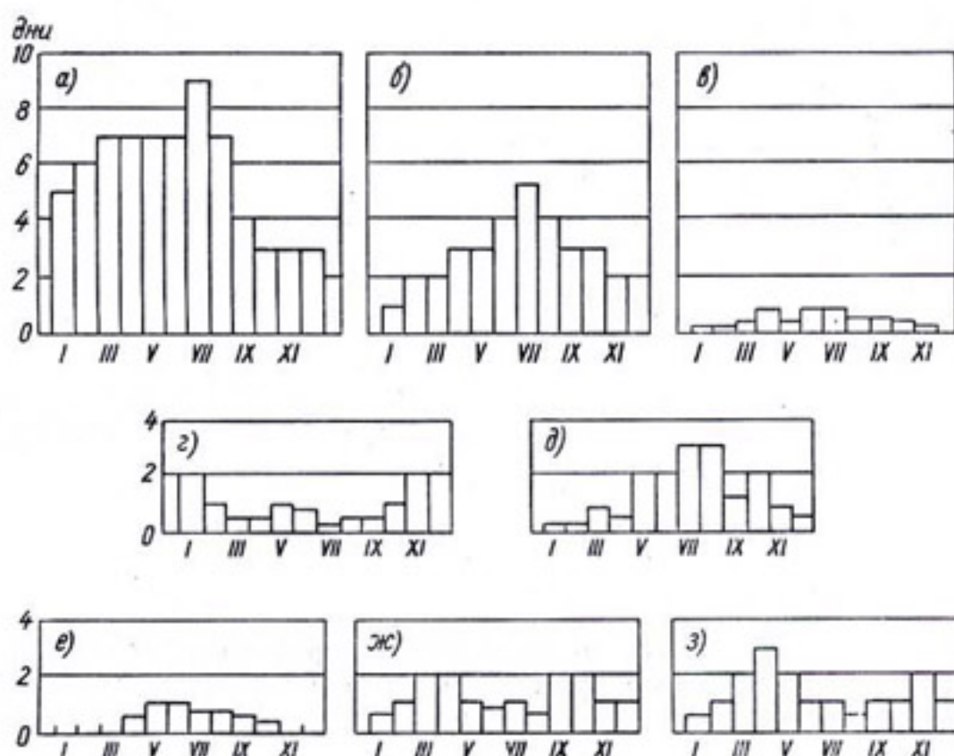
Рис. 92. Годовой ход числа дней с пыльными бурями. Равнины: а — Репетек, б — Тамды, в — Кунград; предгорья: з — Кушка, д — Карши; горы: е — Нарын, ж — Рыбачье, з — Мургаб.
