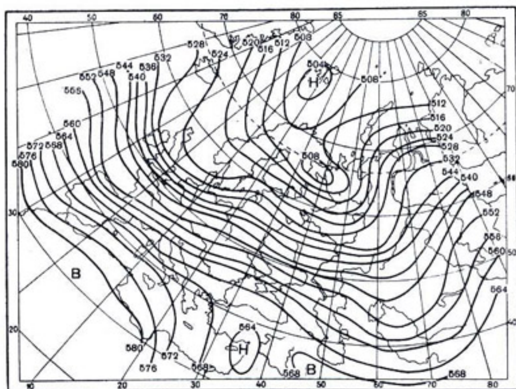
Рис. 14. Карта АТ 500 . 06 час. 19/III 1951 г.
