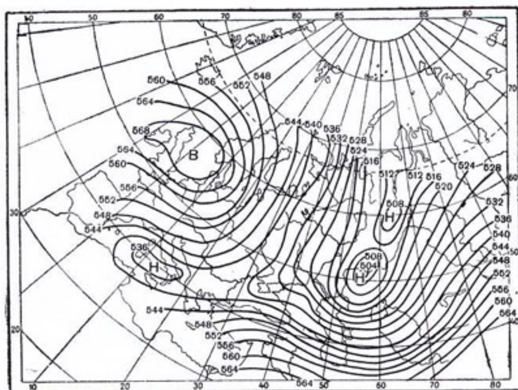
Рис. 18. Карта AT_{500} . 18 час. 20/I 1950 г.
