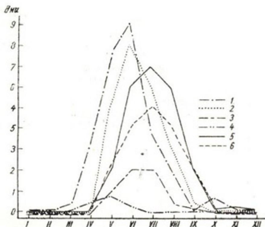
Рис. 90. Годовой ход числа дней с грозой.
