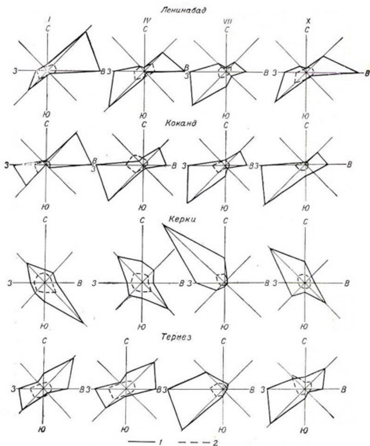
Рис. 39. Направление и скорость ветра. 1 — направление (°), 2 — скорость (м/сек.).
