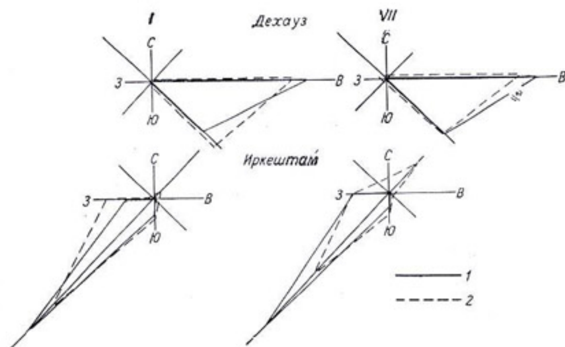
Рис. 48. Направление ветра в различные часы суток. I — 7 час., 2 — 13 час.
