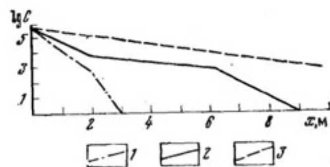
Рис. 12. Дальность распространения микроорганизмов за 60 суток при фильтрации в песках бактериально загрязненной воды со скоростью 1,5 м/сут. (Эффективный диаметр частиц песка 0,2 \text{ мм} < d_{эф} < 0,5 \text{ мм} ): C — количество микробных тел в 1 л воды; x — путь фильтрации; 1 — споры антраконда; 2 — кишечная палочка; 3 — энтерококк
