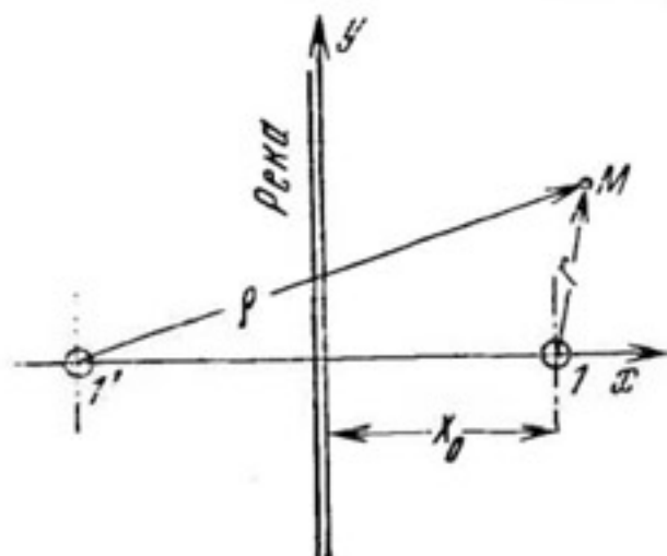
Рис. 16. Схема к расчету скважины у совершенной реки:
