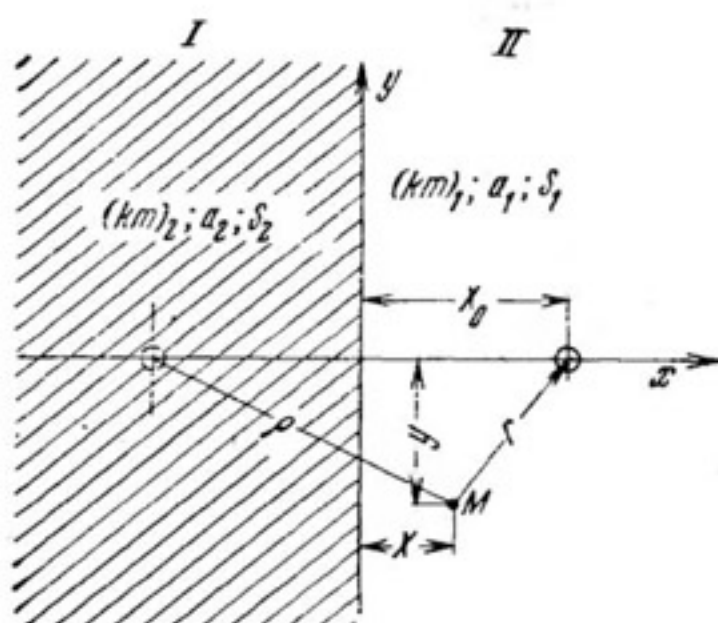
Рис. 24. Схема к расчету скважины в неоднородном пласте с прямой границей раздела зон:
