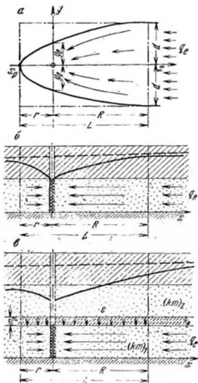
Рис. 57. Схемы фильтрации к водозабору в удалении от реки: а — план; б — разрез для изолированного пласта; в — разрез для пласта с перетеканием
