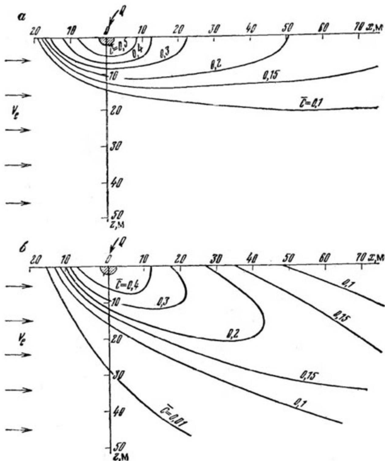
Рис. 35. Ареал распространения загрязнений в подземных водах в районе хранилища при \frac{Q}{2l} = 5 \text{ м}^2/\text{сут} , Kl_e = 0,05 \text{ м/сут} , D_x^* = D_y^* = 0,1 \text{ м}^2/\text{сут} .
