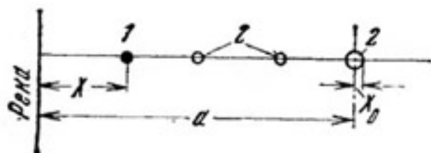
Рис. 69. Схема расположения скважин при запуске индикатора в наблюдательную скважину при откачке вблизи реки: 1 — скважина запуска; 2 — наблюдательные скважины и откачная скважина
