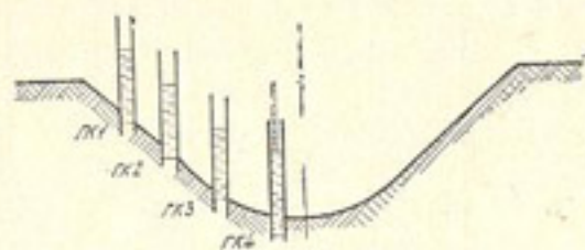
Рис. 41. Схема расположения измерительных труб в выемке
