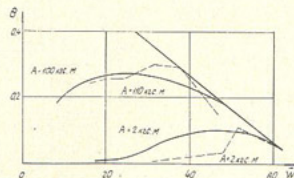
Рис. 33. График зависимости объемной деформации от влажности грунтов: 1 — предельная расчетная деформация; 2 — фактическая предельная деформация (сплошные линии — расчетные кривые, пунктир — фактические изменения деформации от влажности при затратах 100 и 2 кгс·м работы уплотнения)
