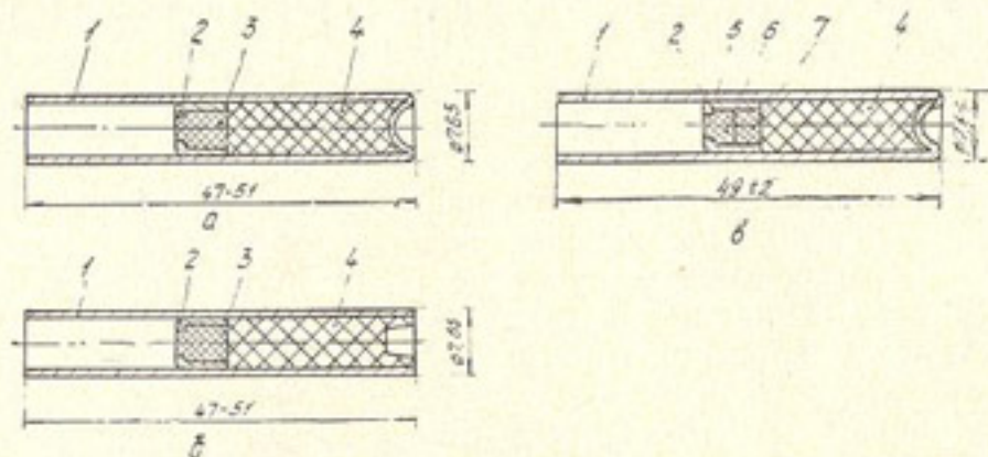
Рис. 6. Капсюли-детонаторы:
