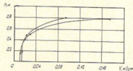
Рис. 44. Характер изменения поглощения воды по периметру выемки
