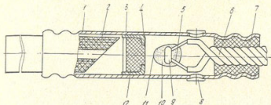
Рис. 18 Электрозажигательная трубка ЭЗТ-2:
