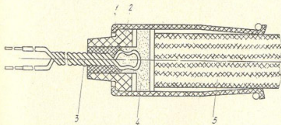
Рис. 19. Разрез патрона электрозажигателя ЭЗП-Б:
