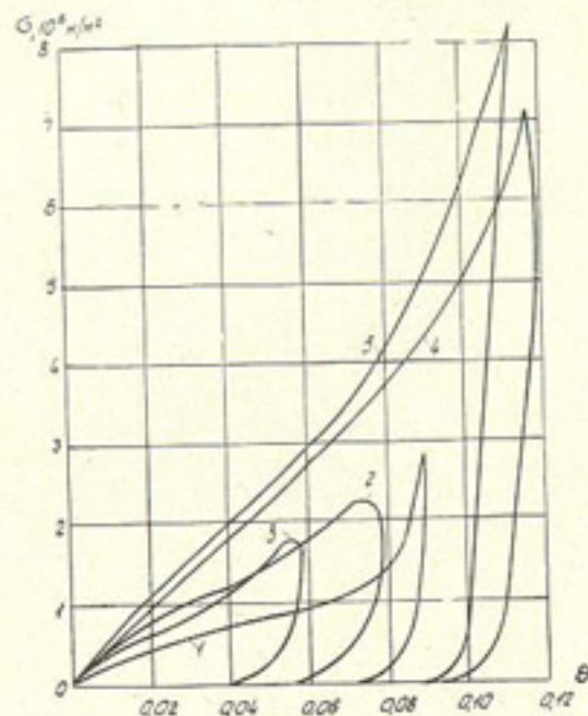
Рис. 32. Кривые напряжения — деформации, полученные путем испытаний образцов суглинков на установке одноосного динамического сжатия при нагружении с различными скоростями:
