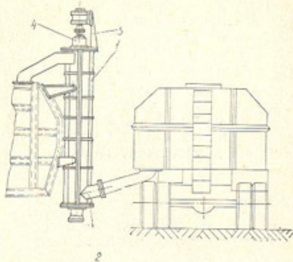
Рис. 61. Транспортер винтовой для загрузки аммиачной селитры в бункер машины:
