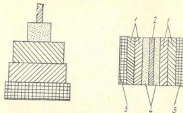
Рис. 17. Разрез огнепроводного шнура:
