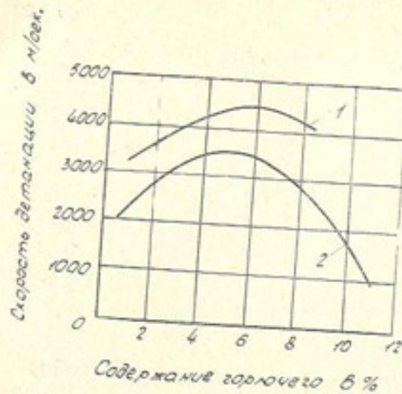
Рис. 45. Изменение скорости детонации игданита от содержания дизельного топлива: 1 — для гранулированной селитры; 2 — для комковой селитры
