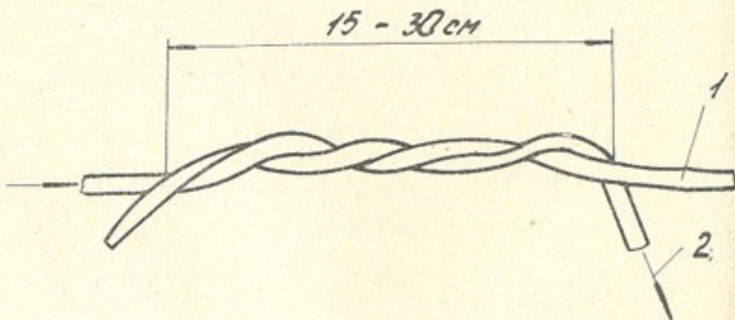
Рис. 14. Схема соединения детонирующего шнура внакрутку: 1 — магистральная ветвь из детонирующего шнура; 2 — отрезок детонирующего шнура (стрелкой показано направление детонационной волны)
