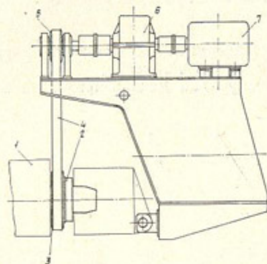
Рис. 55. Ходоуменьшитель:
