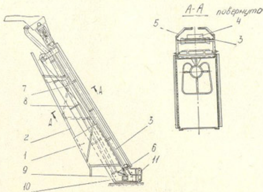
Рис. 62. Камера обслуживания с транспортером подачи иницирующих боевиков и механизмом заворачивания заряда в пленку:
