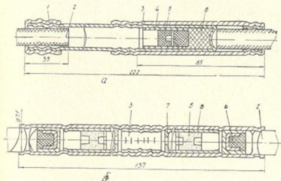
Рис. 15. Схема пиротехнических замедлителей:
