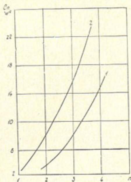
Рис. 20. Графики функции показателя действия взрыва при взрывании в легких, тяжелых (1) и лессовидных (2) суглинках
