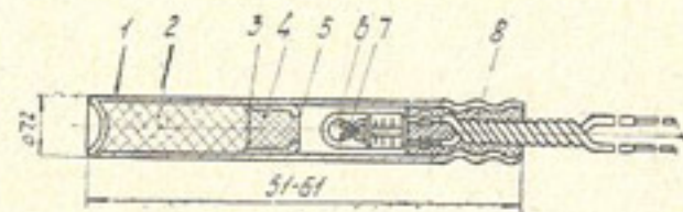
Рис. 8. Конструкция электродетонатора мгновенного действия:
