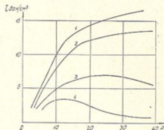
Рис. 34. Изменение интенсивности касательных напряжений грунтов различной весовой влажности: 1 — влажность 9%; 2 — 17%; 3 — 14%; 4 — 9%.
