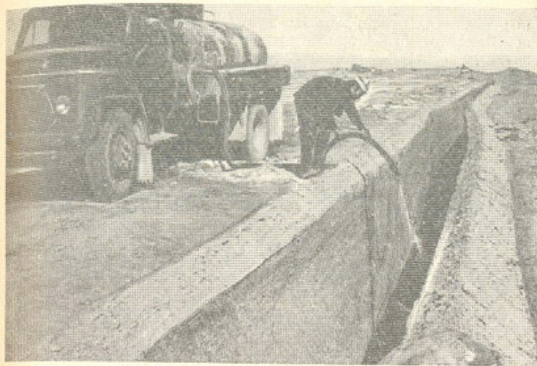
Рис. 5. Получение линейного заряда игданита путем заливки аммиачной селитры дизельным топливом.
