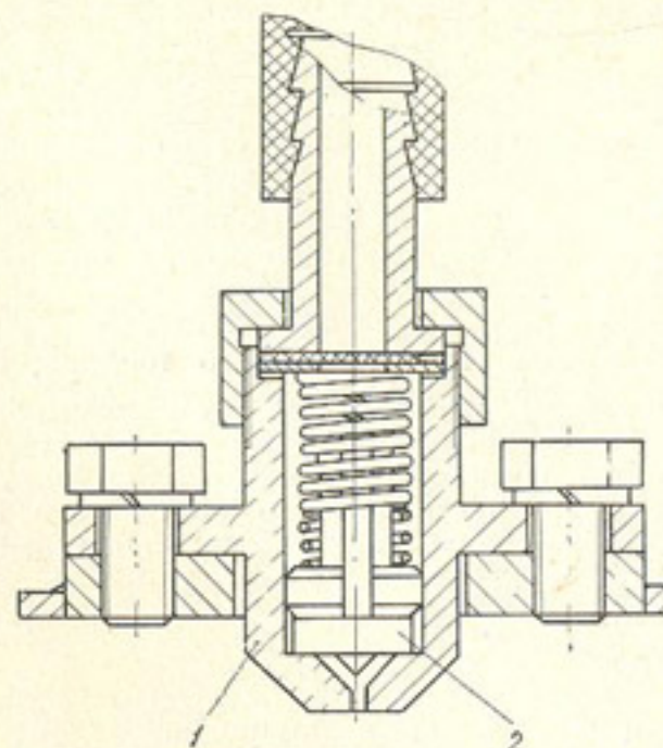
Рис. 67. Форсунка: 1 — корпус; 2 — завихритель
