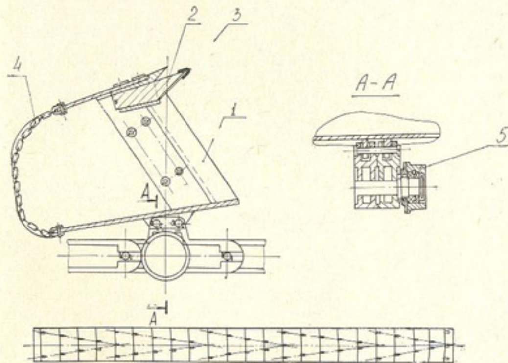
Рис. 59. Ковш и схема расположения зубьев
