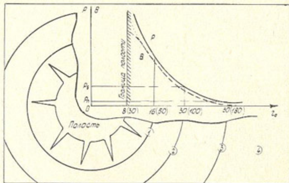
Рис. 36. Распределение зон влияния взрыва в грунтах
