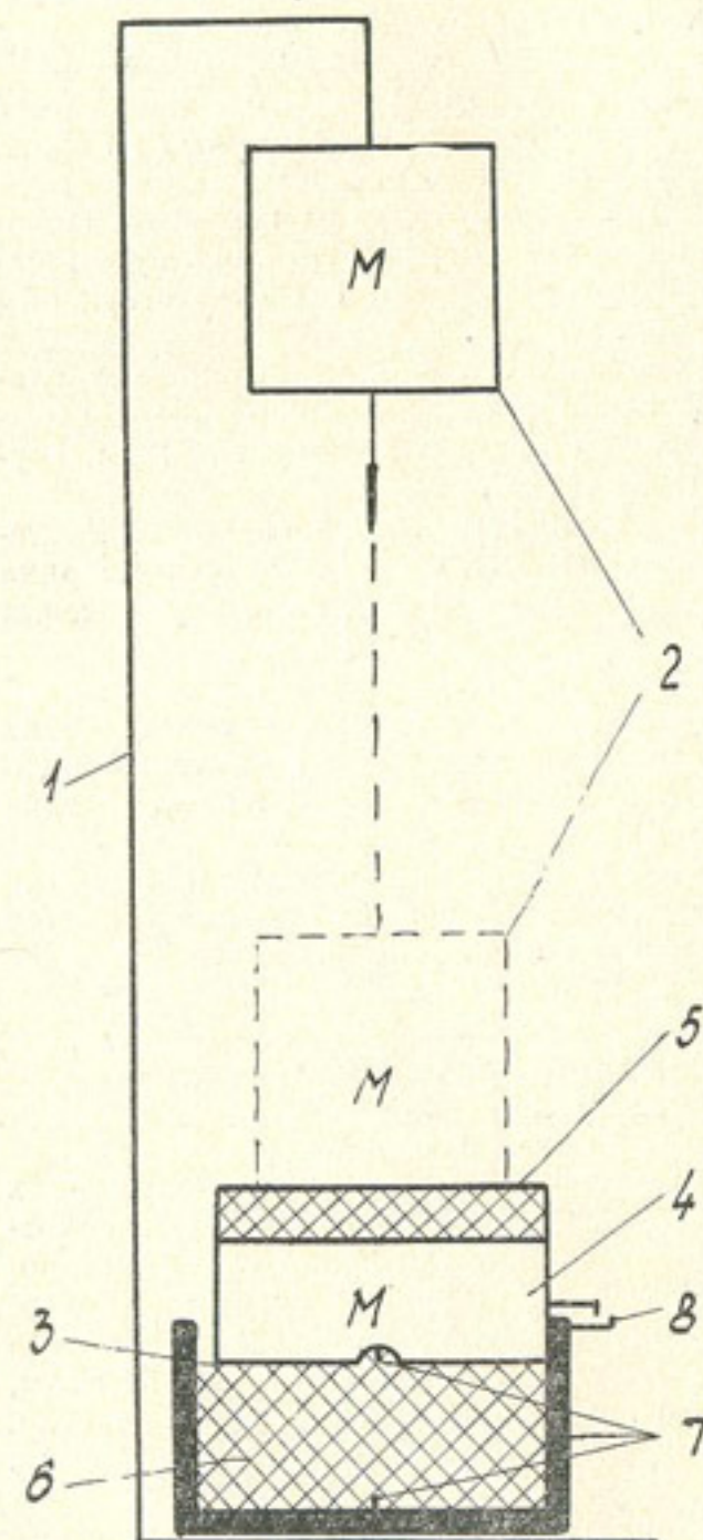
Рис. 30. Схема установки одноосного динамического сжатия: 1 — копер; 2 — груз (M); 3 — обойма-цилиндр; 4 — поршень (M); 5 — прокладка; 6 — образец; 7 — датчик напряжений; 8 — датчик деформаций
