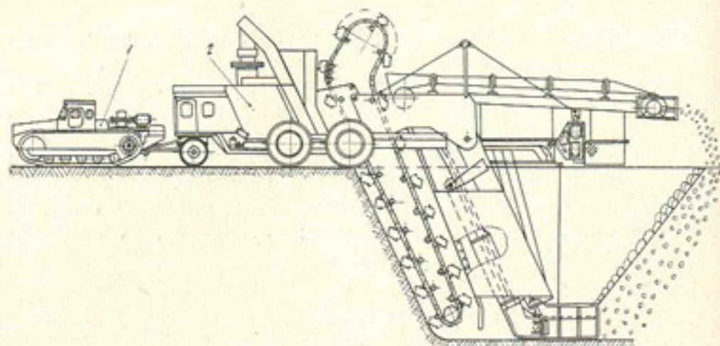
Рис. 50. Установка для механизированной укладки линейных зарядов ВВ:
