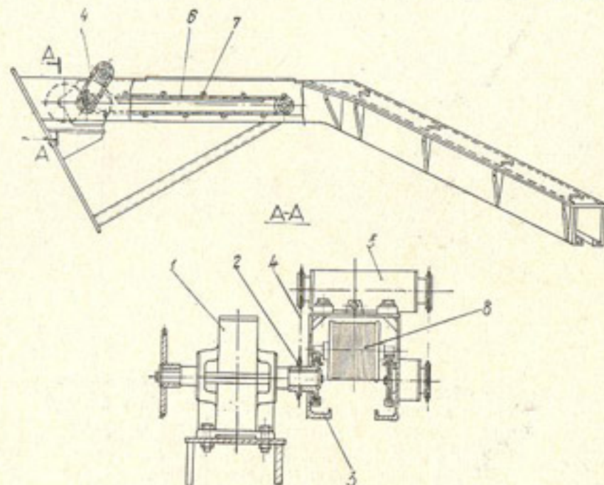
Рис. 63. Механизм автоматического выведения детонирующего шнура на поверхность грунта:
