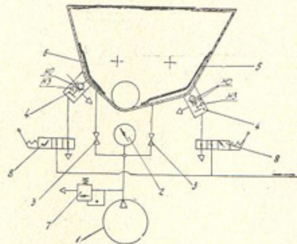
Рис. 57. Схема пневмосистемы бункера:
