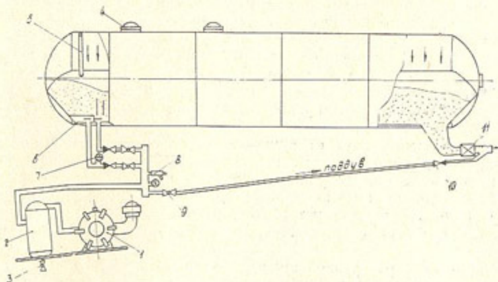
Рис. 53. Схема аэропневматической цистерны: 1 — ротационный компрессор; 2 — маслоотделитель; 3 — кран; 4 — люк; 5 — уравнивающая труба; 6 — аэролоток; 7 — манометр; 8 — предохранительный клапан; 9 — муфтовый кран; 10 — обратный клапан; 11 — разгрузочное устройство
