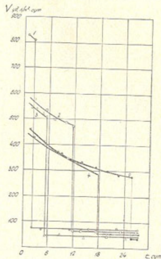
Рис. 39. Удельное водопоглощение из выемок до взрыва (кривые вверх) и после взрыва (прямые вниз)
