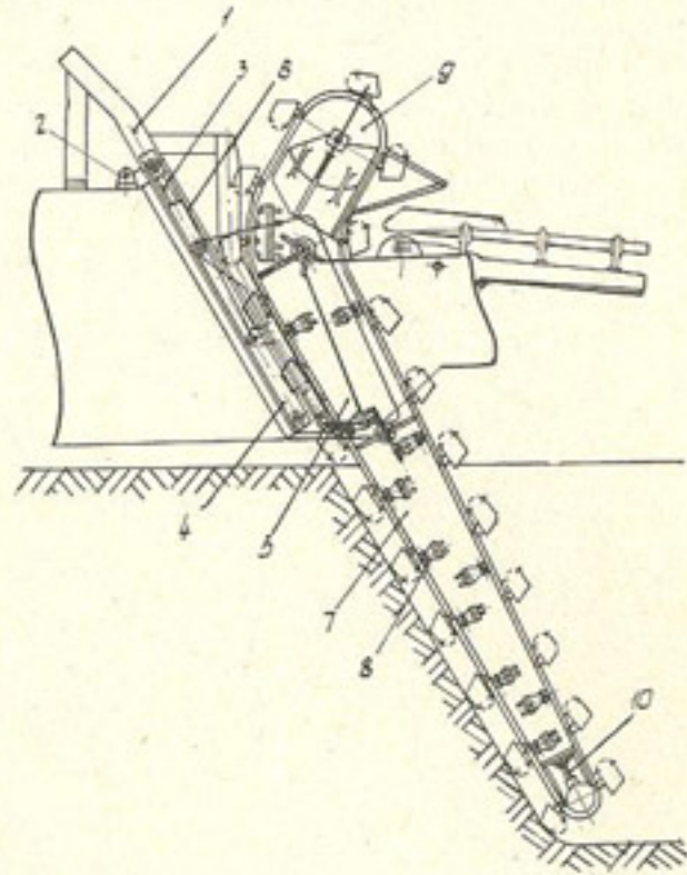
Рис. 58. Копаящий орган:
