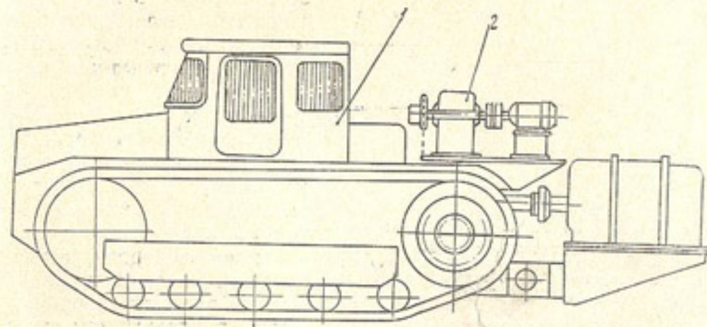
Рис. 54. Агрегат силовой.
