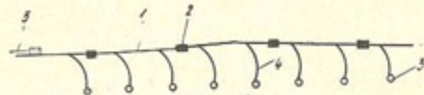
Рис. 16. Схема расположения детонационных реле при массовых взрывах скважинных зарядов:
