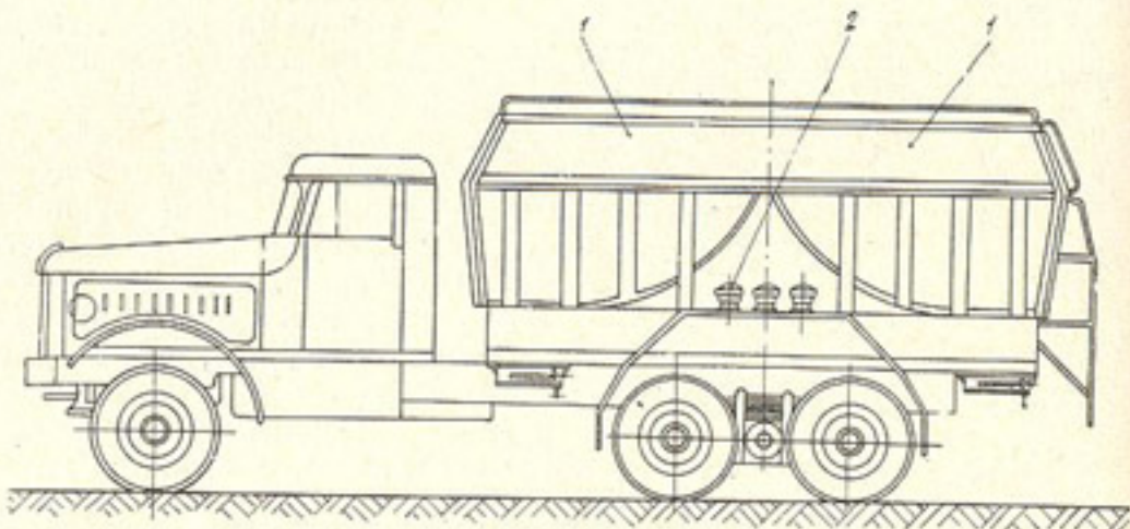
Рис. 51. Машина доставочная: 1 — бункер; 2 — пневмосистема
