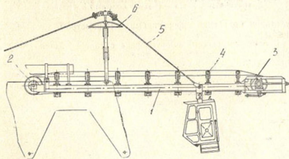
Рис. 64. Транспортер забойки траншеи:
