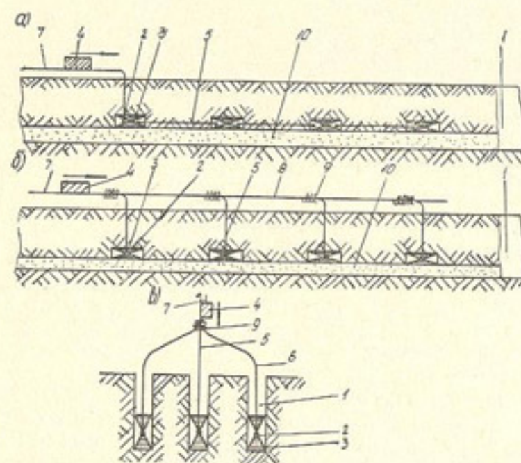
Рис. 12. Схемы соединения отрезков детонирующих шнуров:
