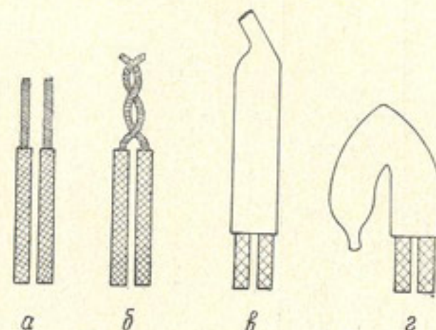
Рис. 10. Соединения проводов электродетонаторов с помощью зажима: а-г — последовательность операций
