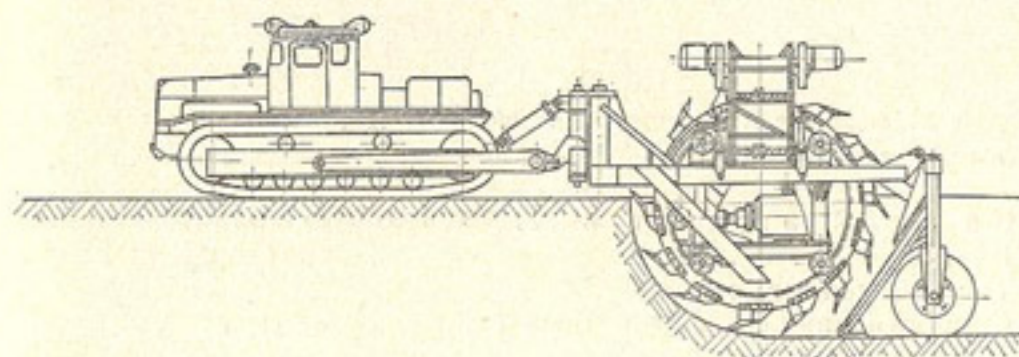
Рис. 49. Роторный траншейный экскаватор ЭТР-253
