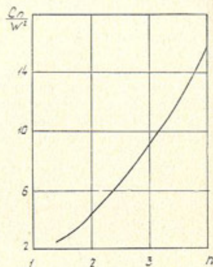
Рис. 21. График функции показателя действия взрыва при взрывании в глинах
