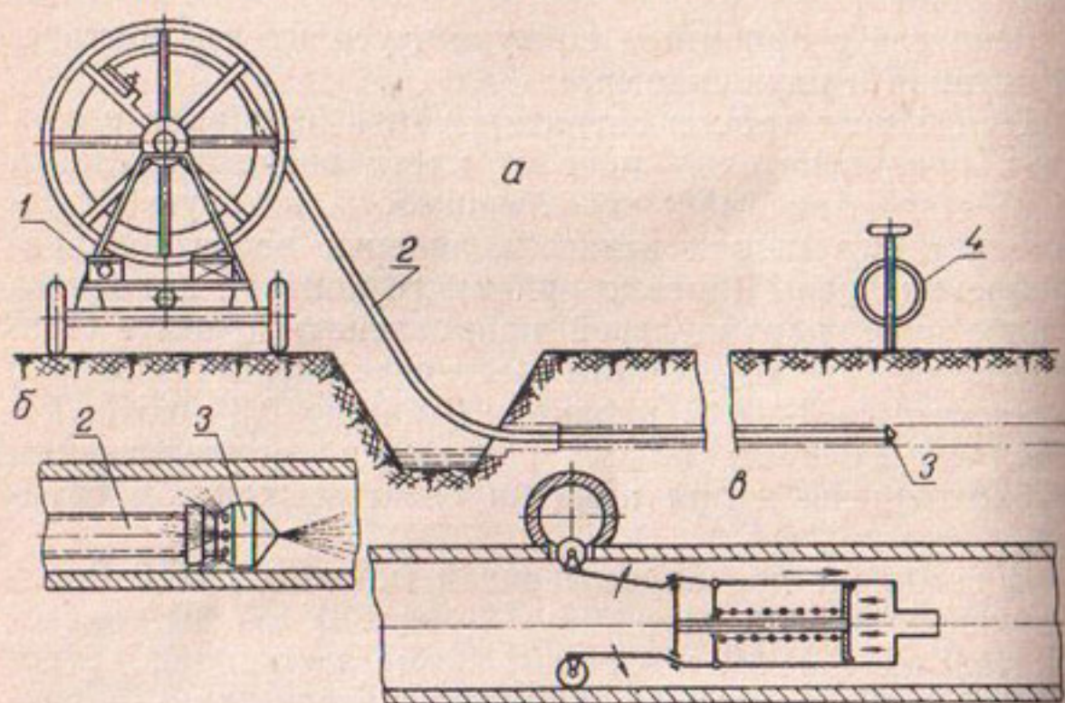
Рис. 78. Схема дренопромывочной машины, трассоискателя и зонда: а — отыскание трассы трассоискателем; б — реактивная головка в действии; в — действие зонда; 1 — генератор; 2 — шланг с проводом; 3 — головка; 4 — трассоискатель с приемным контуром.
