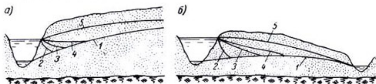
Рис. 8-10. Схемы развития подпора грунтовых вод от водохранилища.
