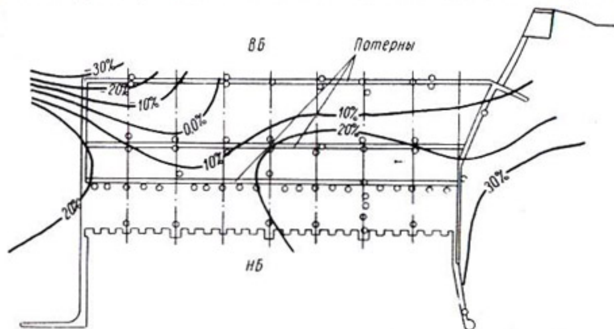
Рис. 3-21. План изолиний разности напоров (в %) между ниже-соликамским и выше-соликамским горизонтами Камской ГЭС.
