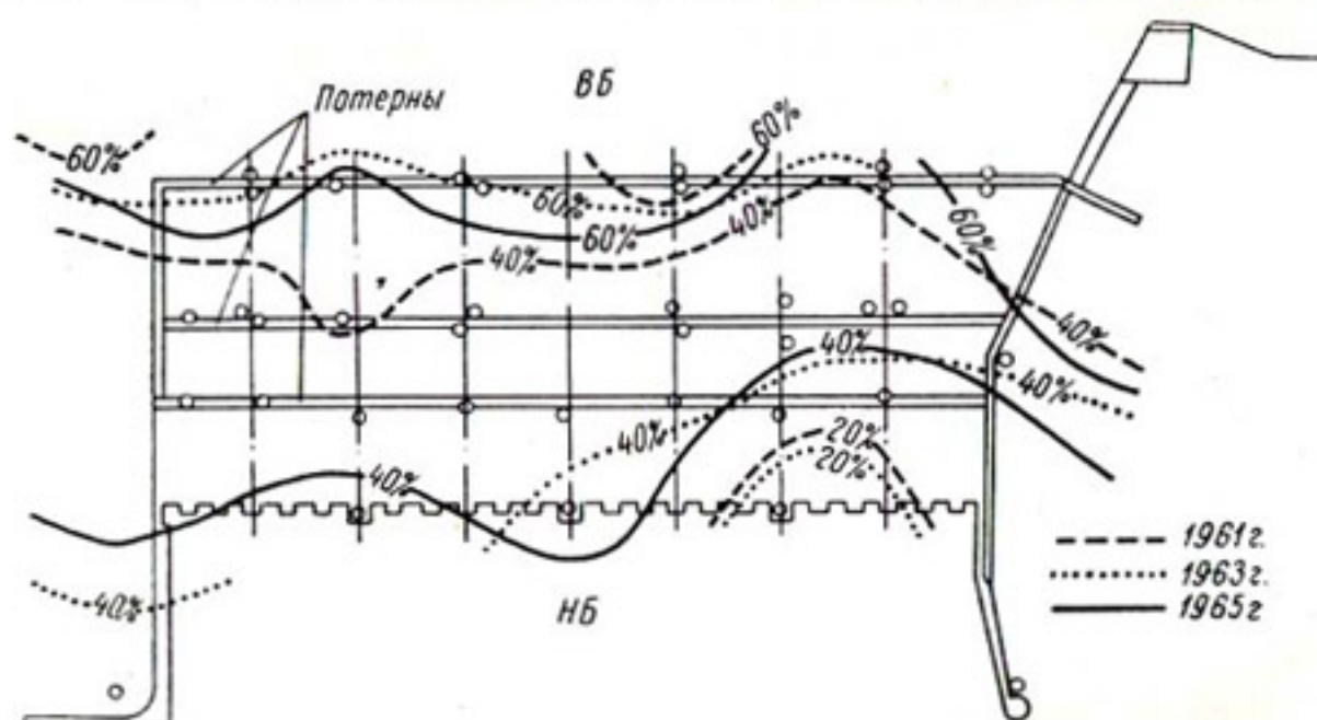
Рис. 3-19. План гидроизопьез верхне-соликамского горизонта Камской ГЭС.
