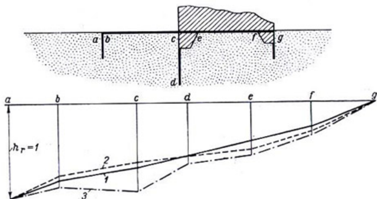
Рис. 8-20. Схема флюتبета и эпюры приведенных напоров.
