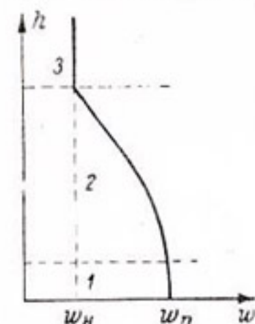
Рис. 2-3. Распределение влагосодержания по высоте пласта.
