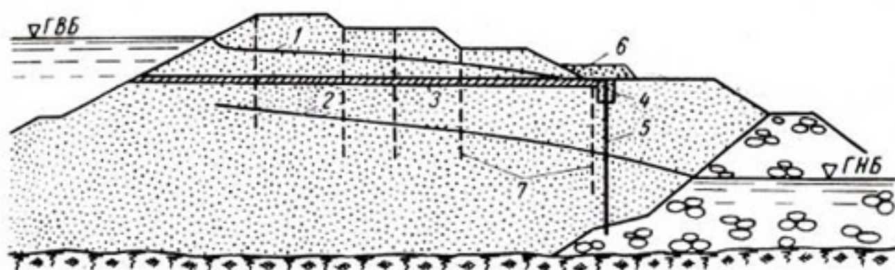
Рис. 9-4. Схема образования двух потоков в намывной плотине.
