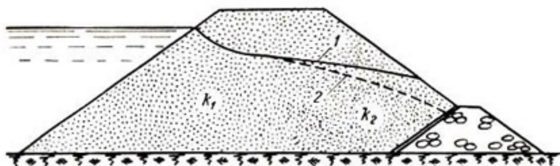
Рис. 9-6. Подъем кривой депрессии вследствие неравномерности укладки тела плотины ( k_1 > k_2 ).
