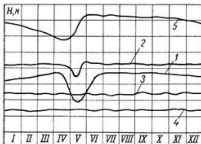
Рис. 6-6. Типовые графики приведенного пьезометрического напора.
