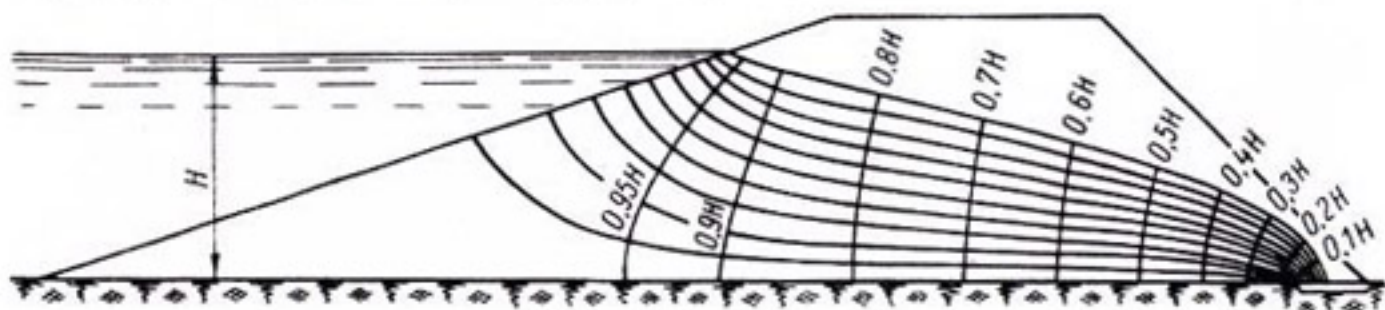
Рис. 3-8. Сетка фильтрации в теле земляной плотины.
