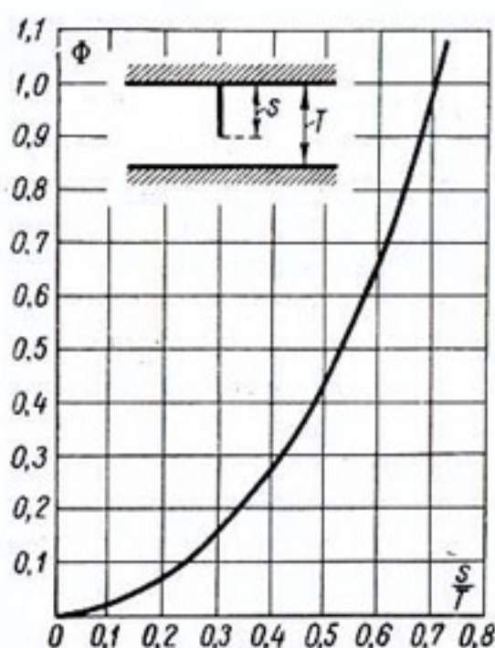
Рис. 8-31. График фильтрационного сопротивления водонепроницаемого шпунта.
