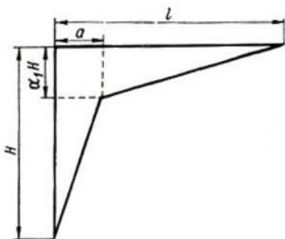
Рис. 8-26. Расчетная эпюра противодействия.
