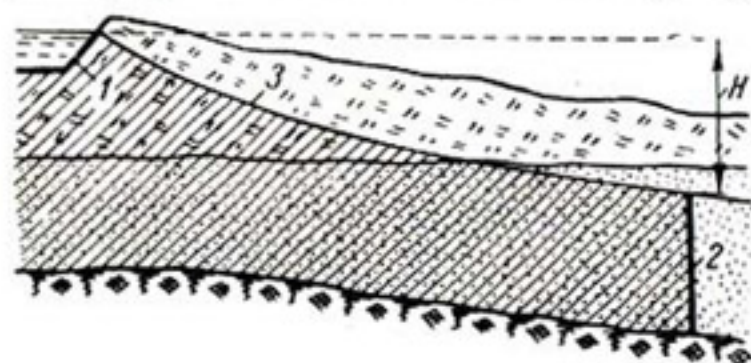
Рис. 8-40. Схема модели области фильтрации.
