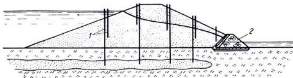
Рис. 3-9. Пьезометрический створ в земляной плотине.
