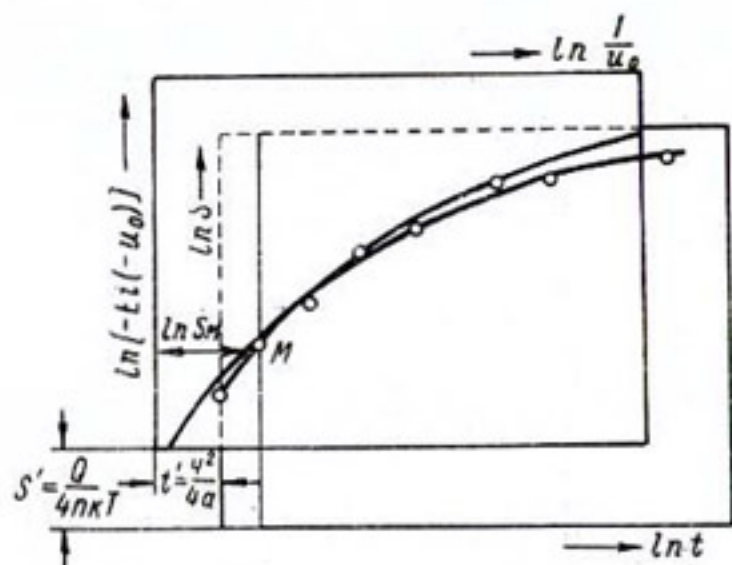
Рис. 6.11. Эталонная кривая для расчета фильтрационных характеристик пласта по опытными данным в период неустановившейся фильтрации.
