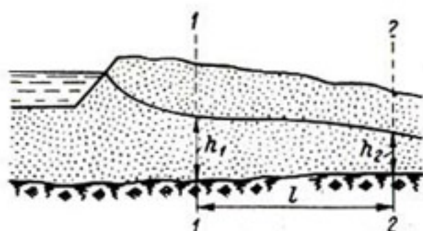
Рис. 8-38. Схема фильтрации из канала при наличии водоупора.
