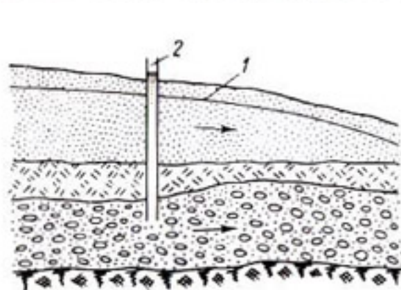
Рис. 3-3. Схема фильтрации в напорном и безнапорном пластах. 1 — кривая депрессии; 2 — пьезометр в напорном пласте.
