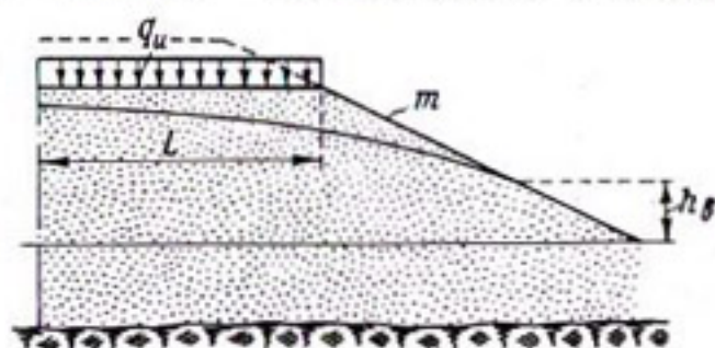
Рис. 8-5. Схема беспрудкового намыва плотины.
