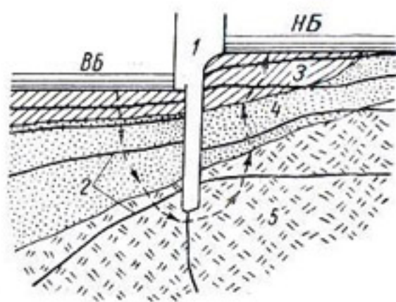
Рис. 3-18. Схема плановой фильтрации в неоднородном пласте.
