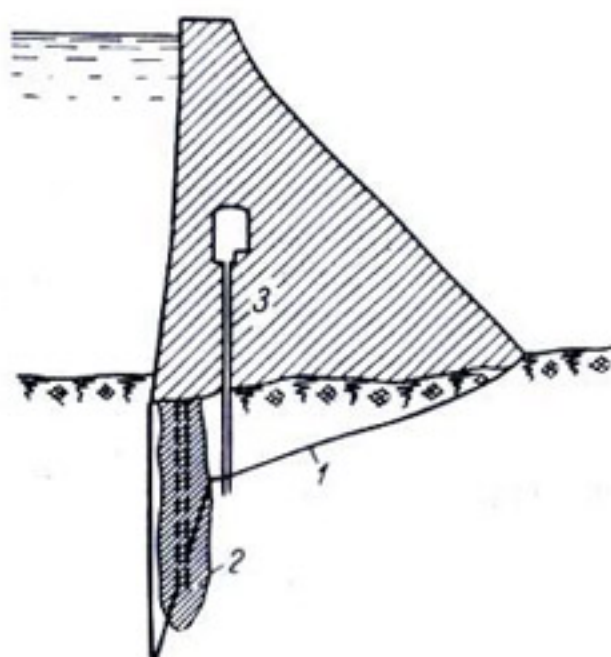
Рис. 8-25. Эпюра приведенного противодействия плотины.
