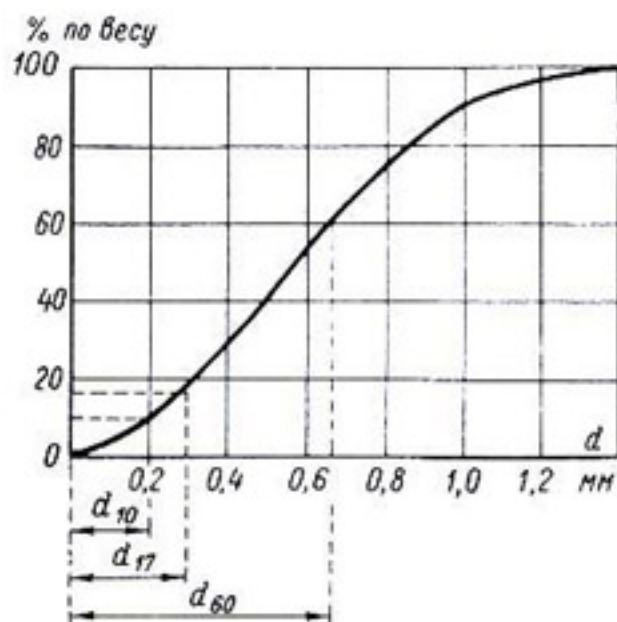
Рис. 2-2. Характерные диаметры фракций грунта.
