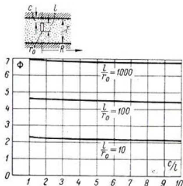
Рис. 5-5. Зависимость фильтрационного сопротивления несовершенных скважин от отношения c/l .
