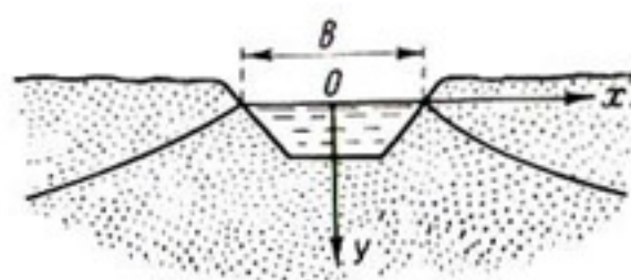
Рис. 8-39. Схема подпертой фильтрации из канала при глубоком залегании водоупора.
