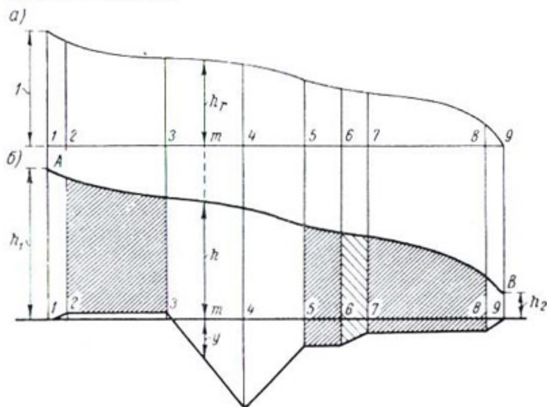
Рис. 2-11. Эпюры: а — приведенных напоров h_r ; б — давлений
