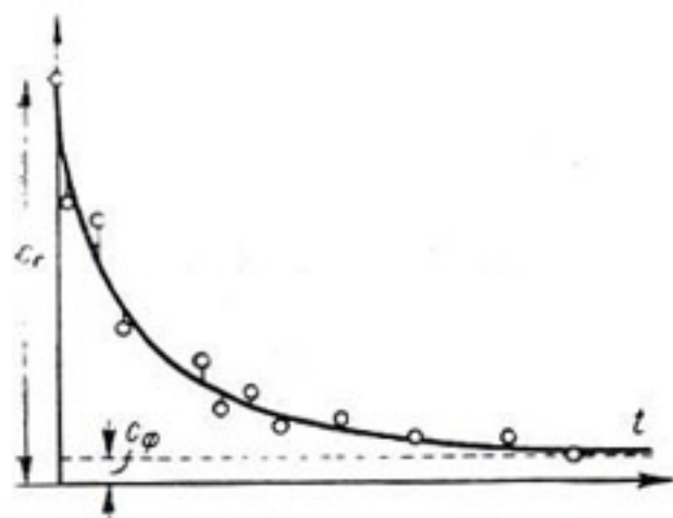
Рис. 4-3. Кривая разбавления. c_0 — начальная концентрация индикатора; c_\phi — концентрации вещества индикатора в условиях естественного потока (фон).
