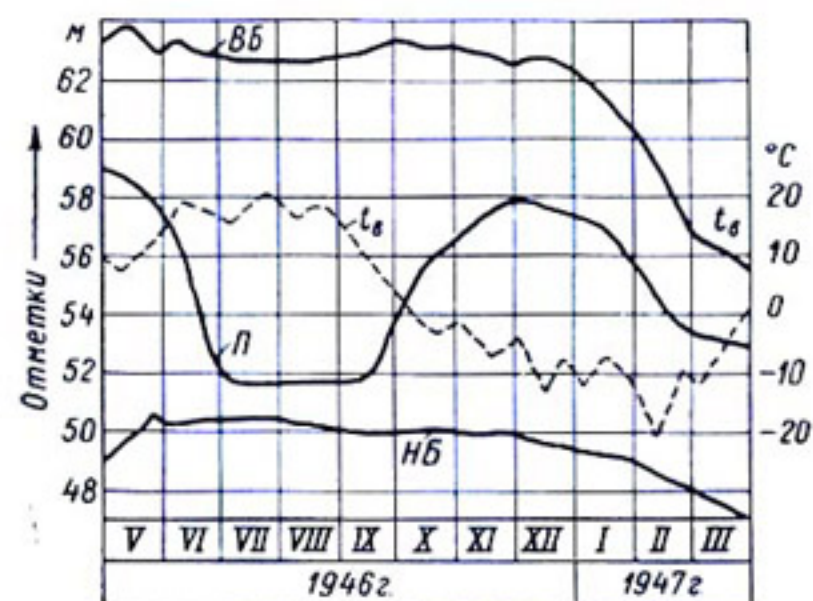
Рис. 8-14. Кривые изменения уровней бьефов ВБ и НБ, воды в пьезометре П и температуры воздуха t_{\text{в}} .
