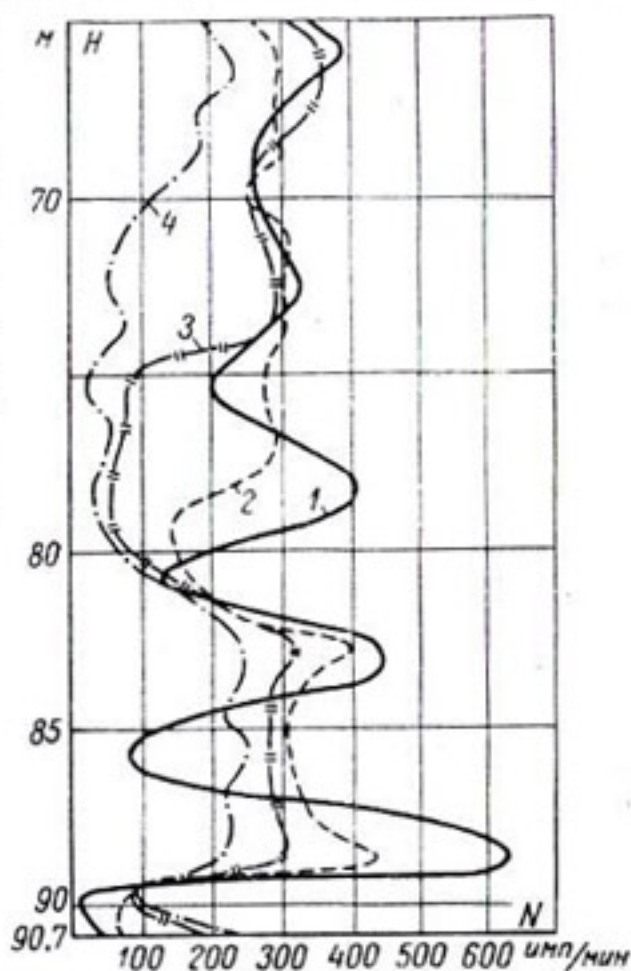
Рис. 4-4. Распределение радиоактивного индикатора по высоте пусковой скважины в различные моменты времени.
