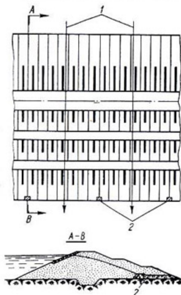
Рис 4-1. Схема к определению скоростей фильтрации по расходам из горизонтального дренажа низовой грани земляной плотины.
