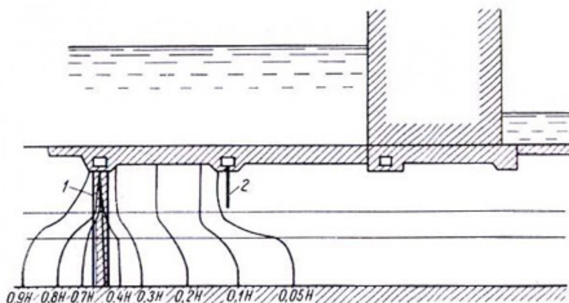
Рис. 4-2. Схема к определению скоростей фильтрации по расходу вертикального дренажа в основании бетонной плотины.
