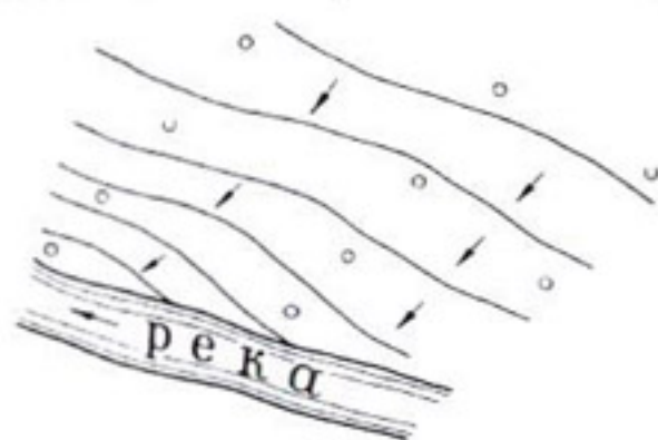
Рис. 3-1. План гидроизогипс и пьезометрическая сеть. о — пьезометры.
