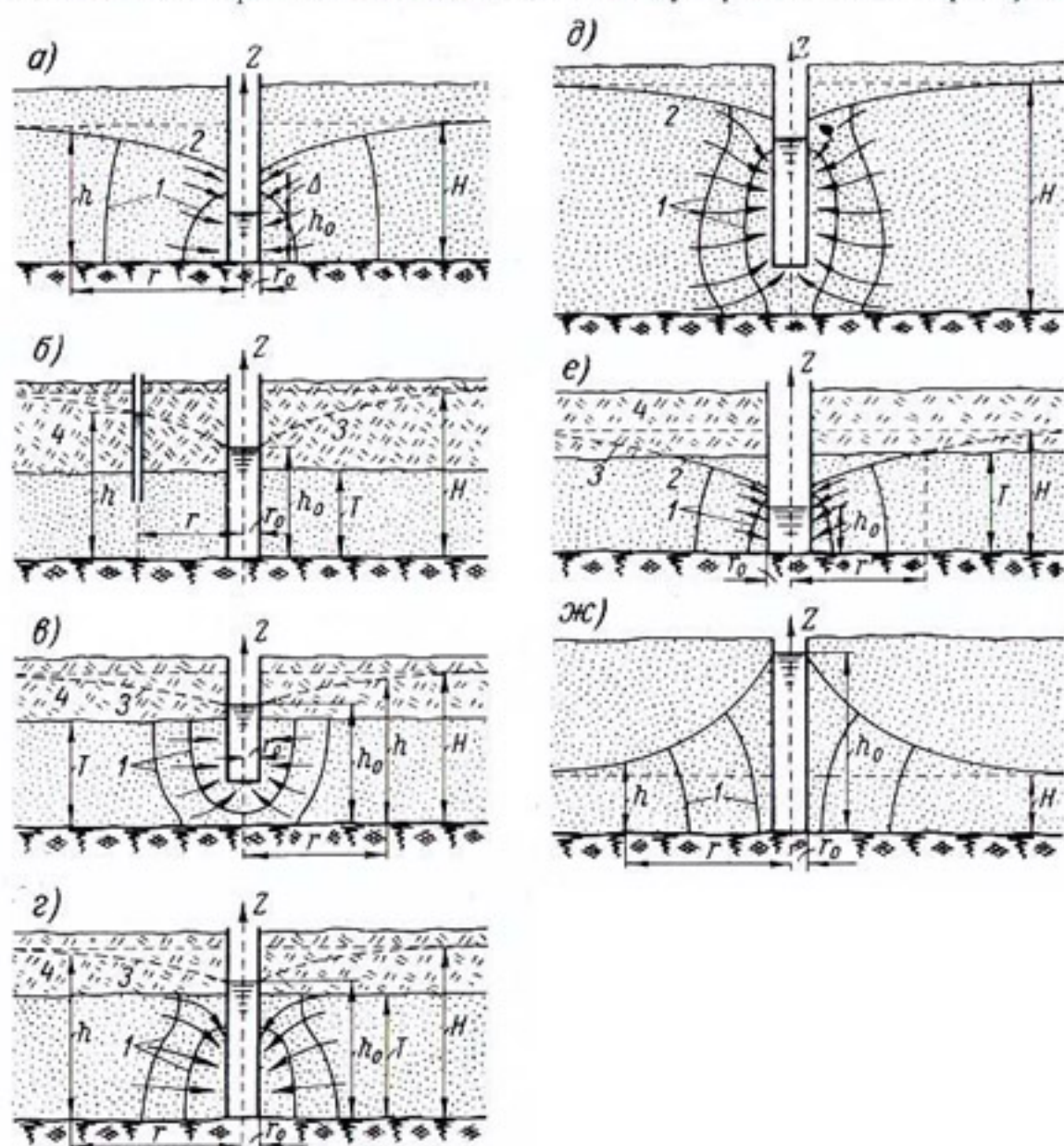
Рис. 2-6. Схемы фильтрации при различных типах скважин: а — безнапорная совершенная скважина; б — напорная совершенная скважина; в — напорная несовершенная по степени вскрытия пласта скважина; г — напорная несовершенная по характеру вскрытия пласта скважина; д — безнапорная несовершенная по степени и характеру вскрытия пласта скважина; е — напорно-безнапорная совершенная скважина; ж — безнапорная совершенная поглощающая скважина.
