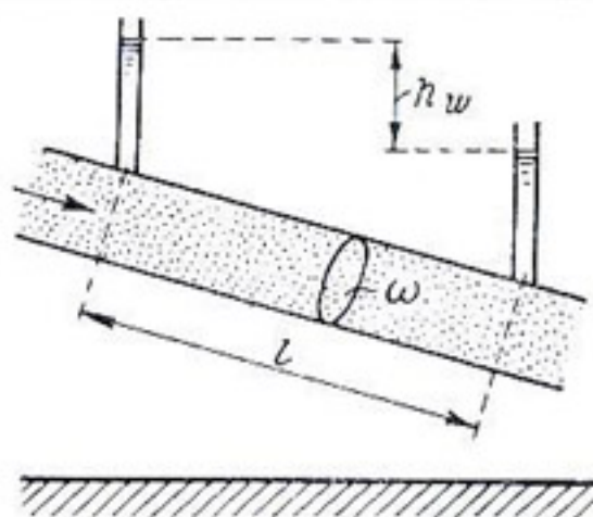
Рис. 2-4. Схема фильтрации в цилиндрической трубе.
