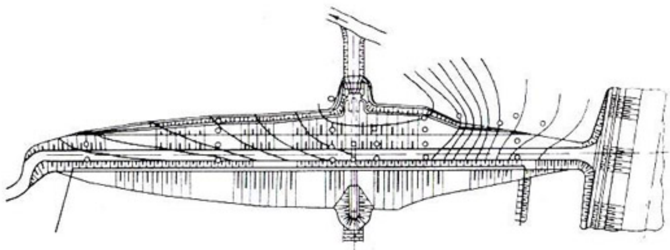
Рис. 9-7. Гидроизогины в земляной плотине с экраном.
