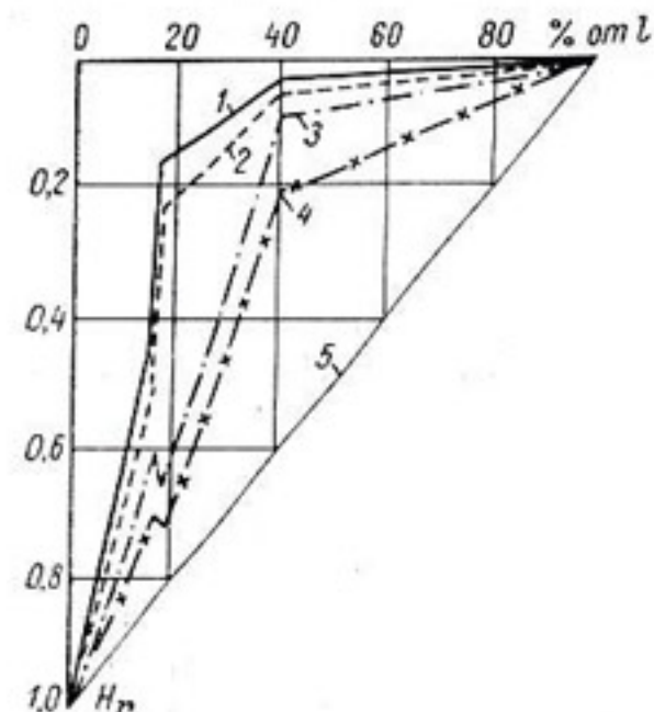
Рис. 8-24. Эпюра приведенного противодействия.
