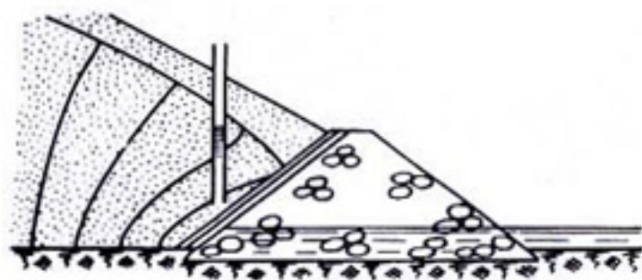
Рис. 7-7. Пьезометр в зоне обратного фильтра.
