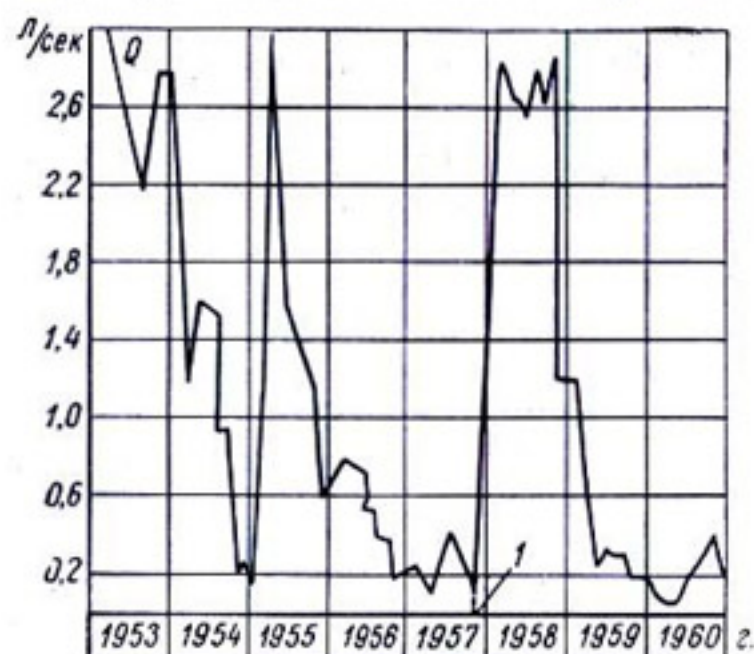
Рис. 8-15. График дебита скважины. 1 — момент смены фильтра.
