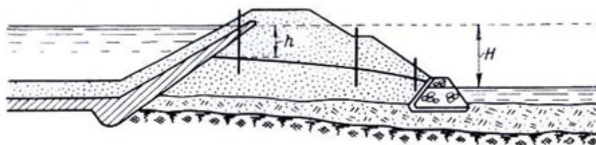
Рис. 3-10. Пьезометрический створ в земляной плотине с экраном.
