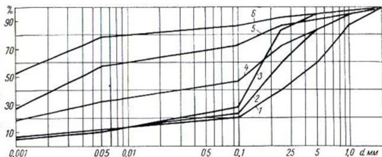
Рис. 2-1. Кривые гранулометрического анализа грунтов.
