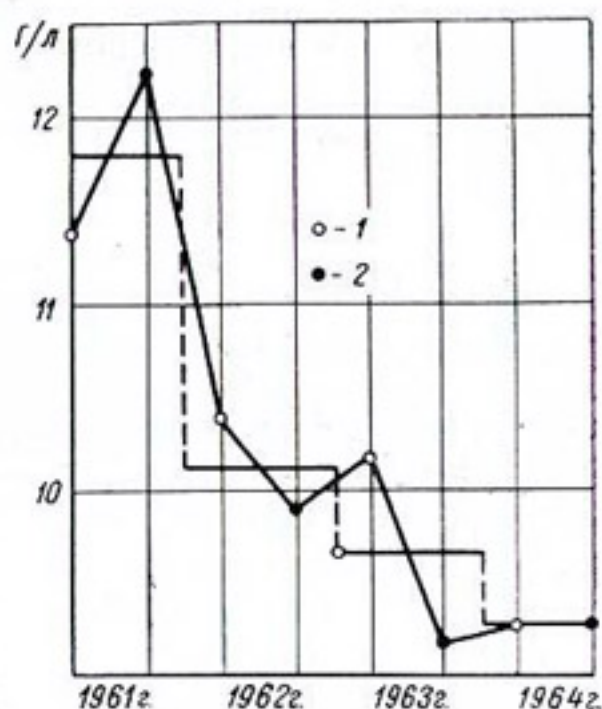
Рис. 8-18. График сезонных изменений осредненных значений минерализации по пробам воды из пьезометров нижне-соликамского горизонта в цементационной потерне.
