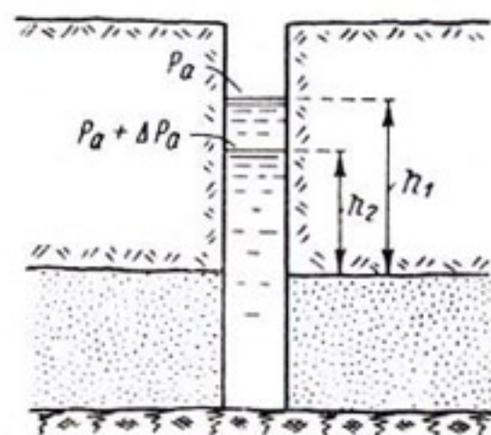
Рис. 3-14. Изменение уровня воды в пьезометре при изменении атмосферного давления.
