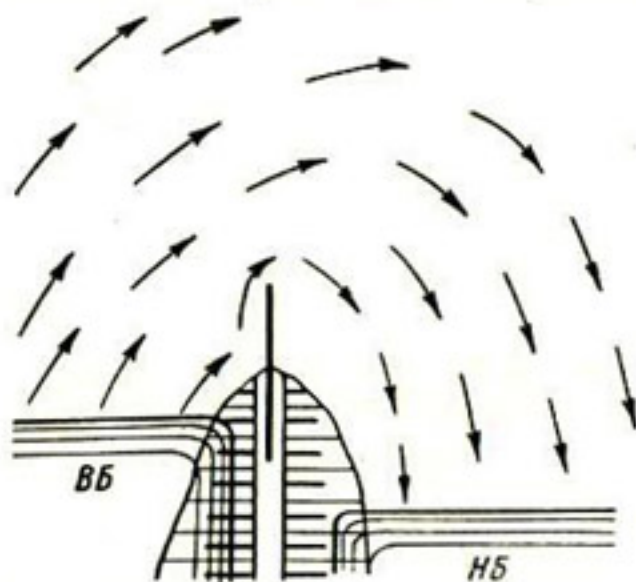
Рис. 8-9. Схема фильтрации в береговом примыкании земляной плотины.
