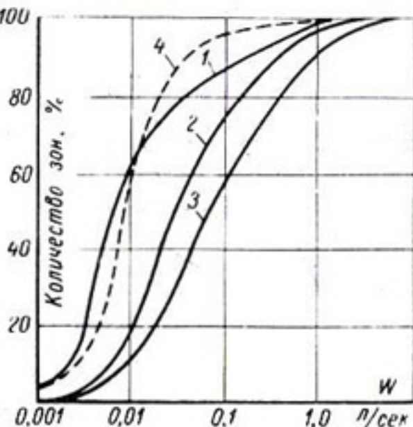
Рис. 8-28. Статистические кривые удельного водопоглощения.
