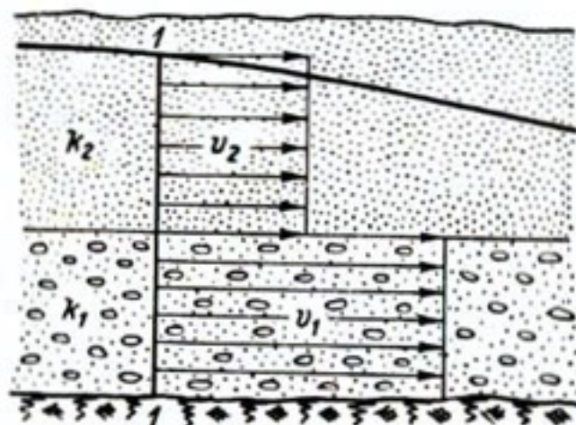
Рис. 2-7. Эпюра скоростей фильтрации в слоистом пласте.
