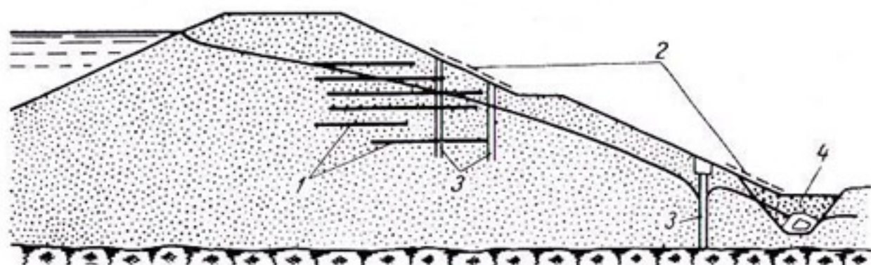
Рис. 9-5. Высачивание на откос намывной плотины.
