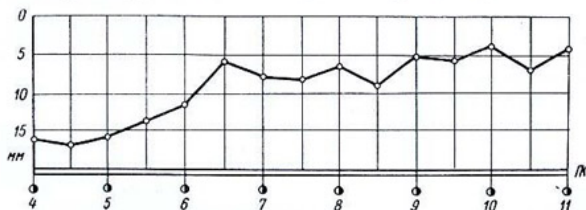
Рис. 7-4. Типовой график распределения осадок вдоль фронта сооружения.
