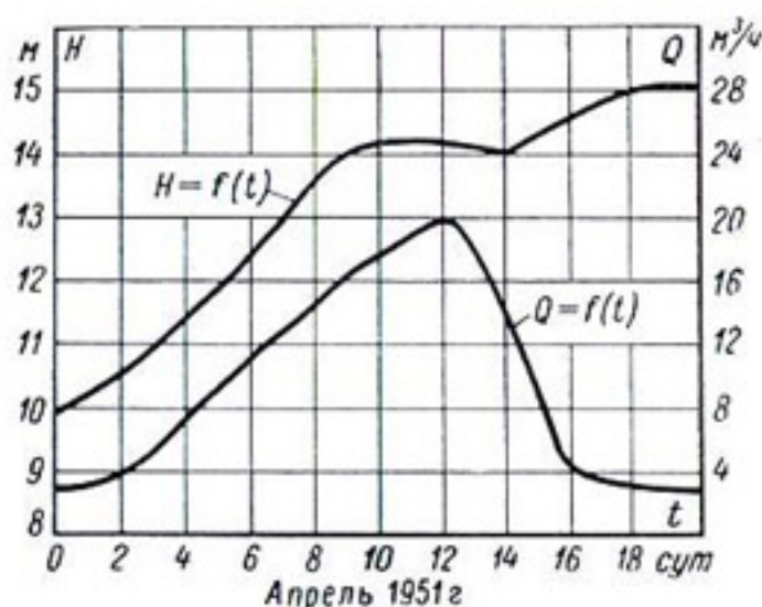
Рис. 8-3. Графики расхода Q и напора H перемычки.
