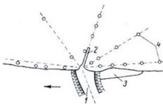
Рис. 3-6. Схема лучевого расположения пьезометров в береговом примыкании.
