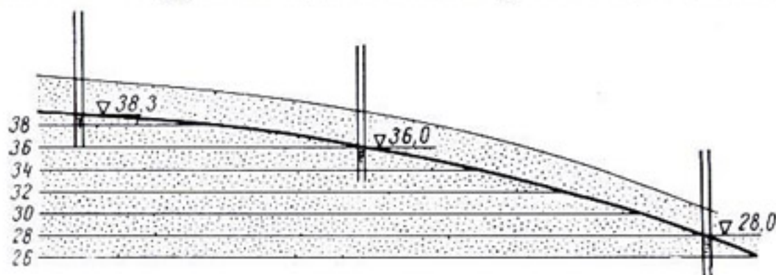
Рис. 3-16. Кривая депрессии в пьезометрическом створе.
