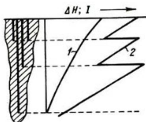
Рис. 8-29. Эпюры падения напора и градиентов напора по длине трехъярусной завесы.
