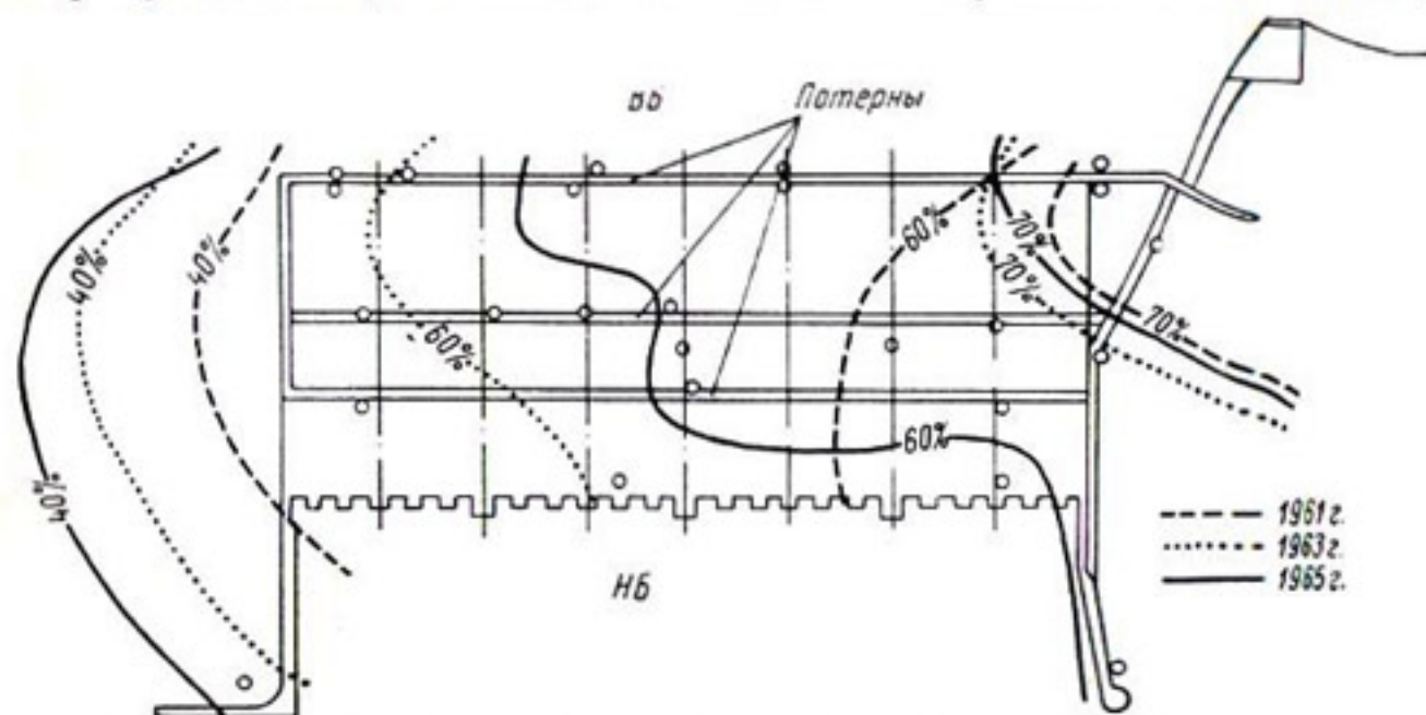
Рис. 3-20. План гидроизопьез ниже-соликамского горизонта Камской ГЭС.
