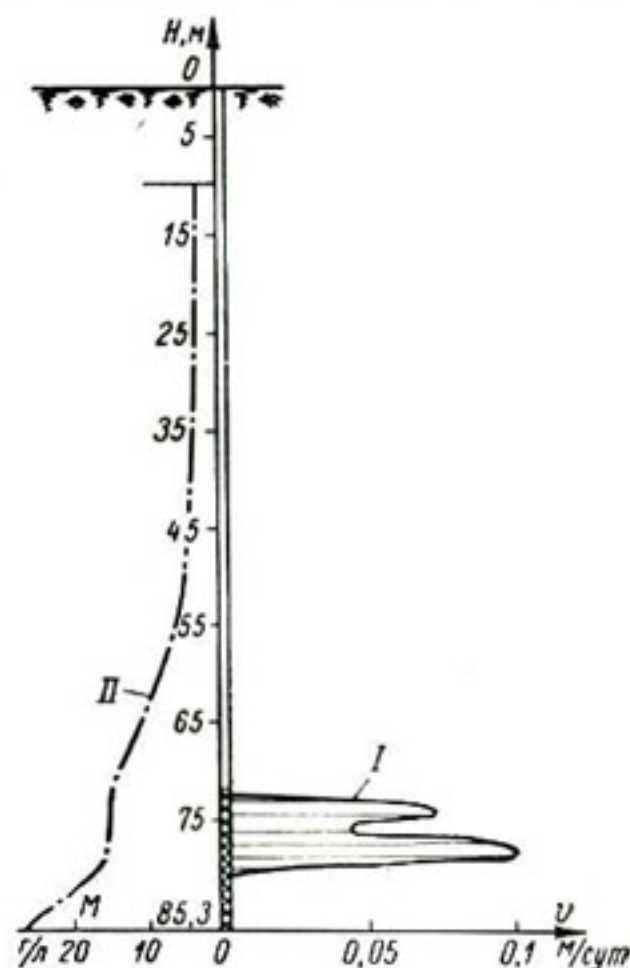
Рис. 7-9. Результаты фильтрационного каротажа пьезометра.
