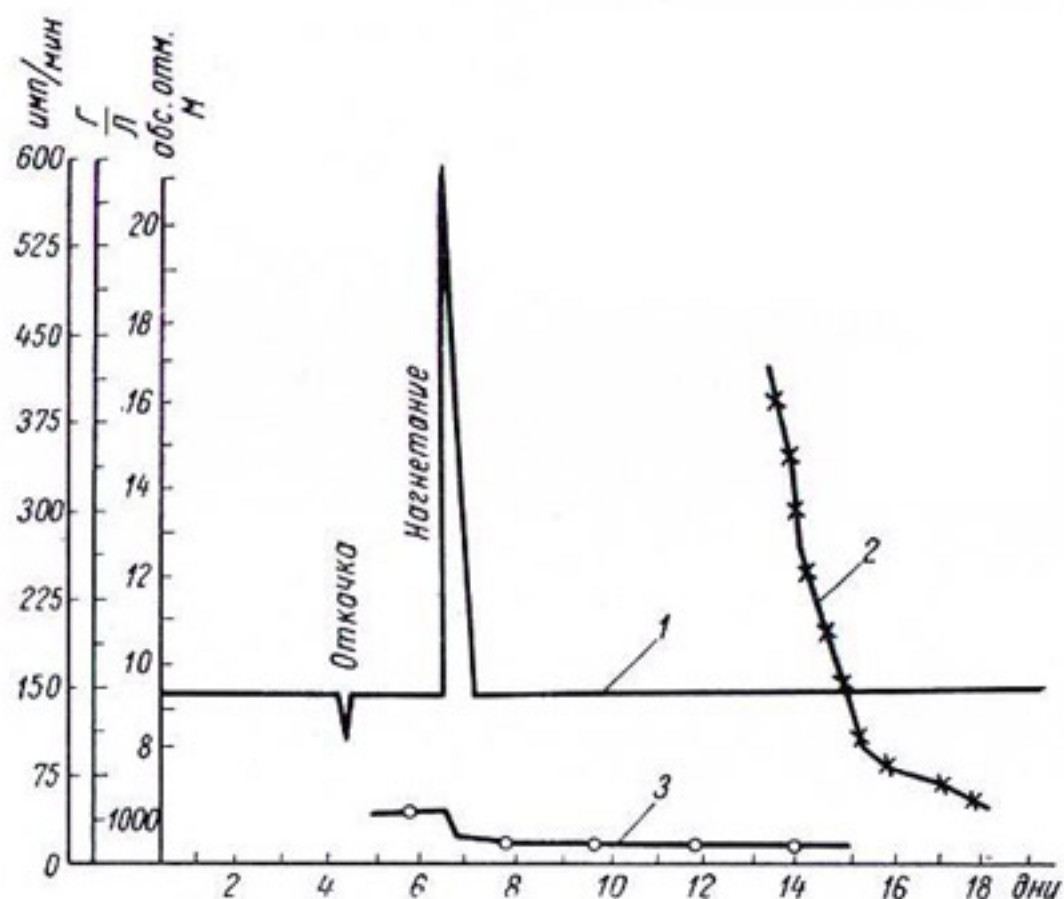
Рис. 5-8. Результаты экспериментального обследования типового пьезометра.
