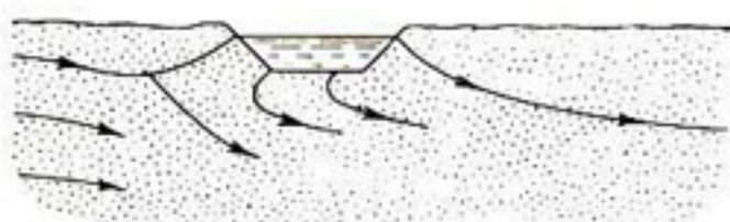
Рис. 8-36. Схема подпертой фильтрации из канала.
