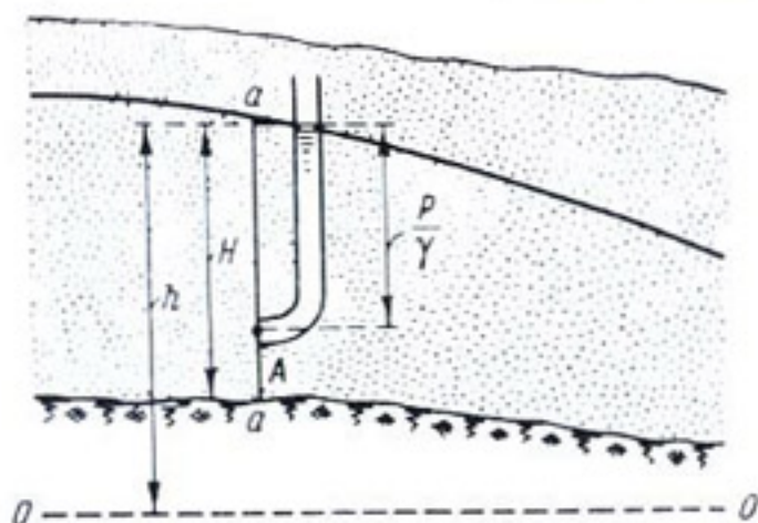
Рис. 2-9. Схема плавно изменяющейся фильтрации.
