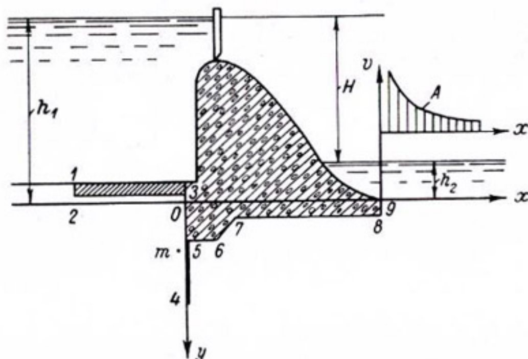
Рис. 2-10. Схема подземного контура плотины.
