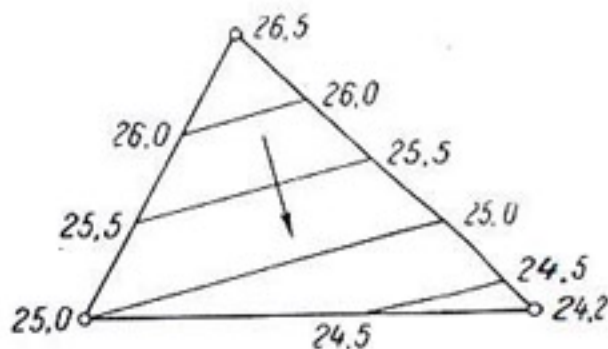
Рис. 3-15. Определение направления фильтрации по уровням трех скважин.
