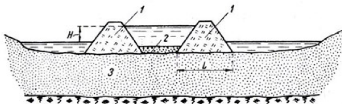
Рис. 8-6. Схема полевых опытов по исследованию суффозии цементированного грунта.
