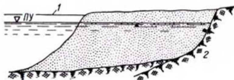
Рис. 3-7. Распространение подпора в аллювиальной террасе.
