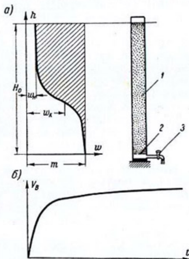
Рис. 6-1. Расчетная схема для определения количественных характеристик водоотдачи грунта: а — эпюра распределения остаточного влагосодержания по высоте осушенного образца грунта; заштрихованная площадь соответствует количеству воды, вытекшей из образца к моменту времени t ; б — зависимость объема дренированной воды от времени.
