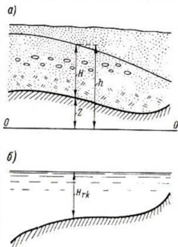
Рис. 5-3. Схема плановой фильтрации и ее модели.
