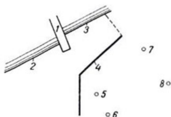
Рис. 3-17. Случай недостаточного количества наблюдательных скважин.
