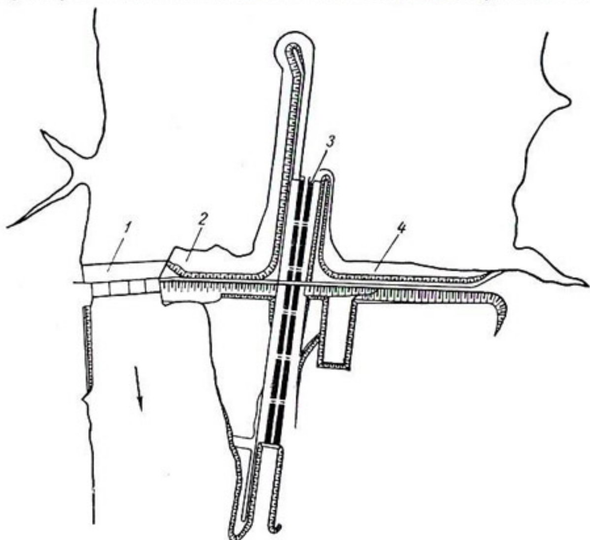
Рис. 8-16. Схематизированный план Камского гидроузла.
