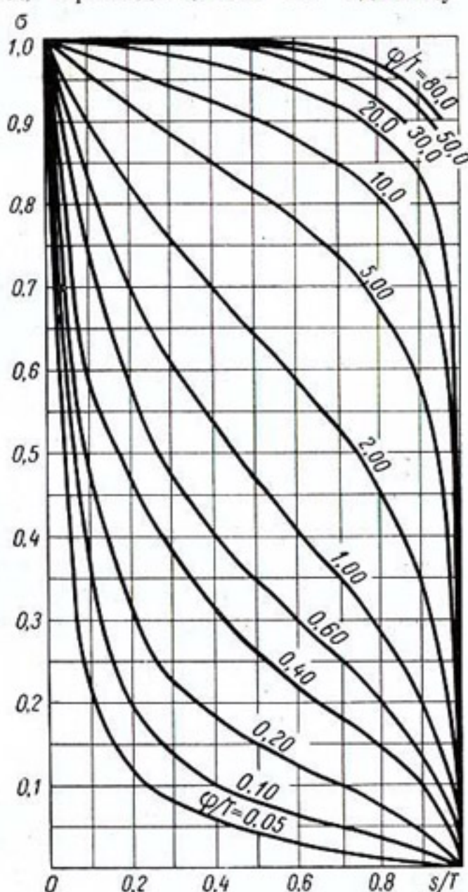
Рис. 8-32. График для расчета шпунтовых рядов.
