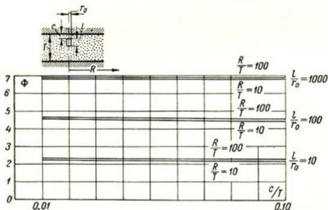
Рис. 5-6. Зависимость фильтрационного сопротивления несовершенных скважин от c/T .
