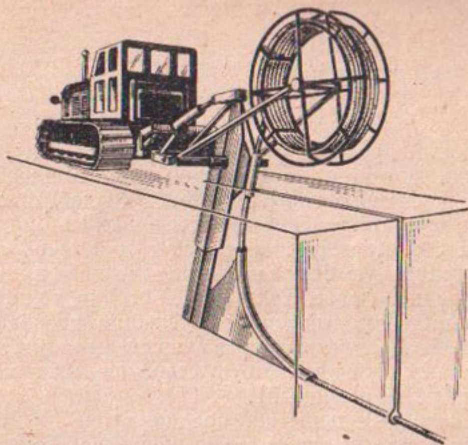
Рис. 1. Бестраншейный дрепоукладчик ДПБН-1,8.
