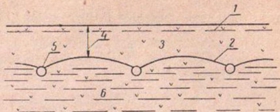
Рис. 5. Действие дренажа:
