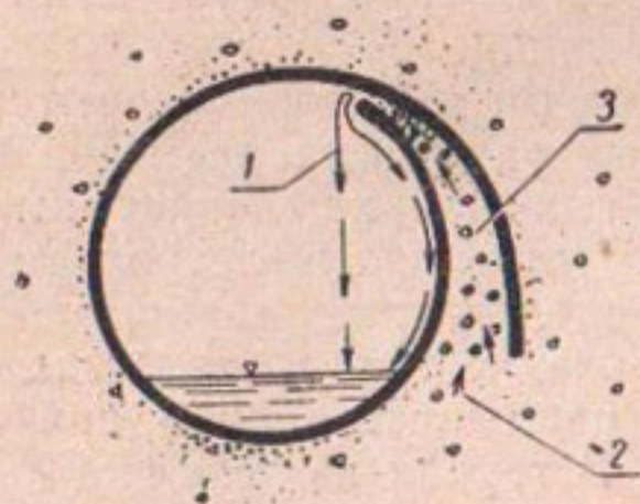
Рис. 8. Незаиляемая дренажная труба из упругой ленты:
