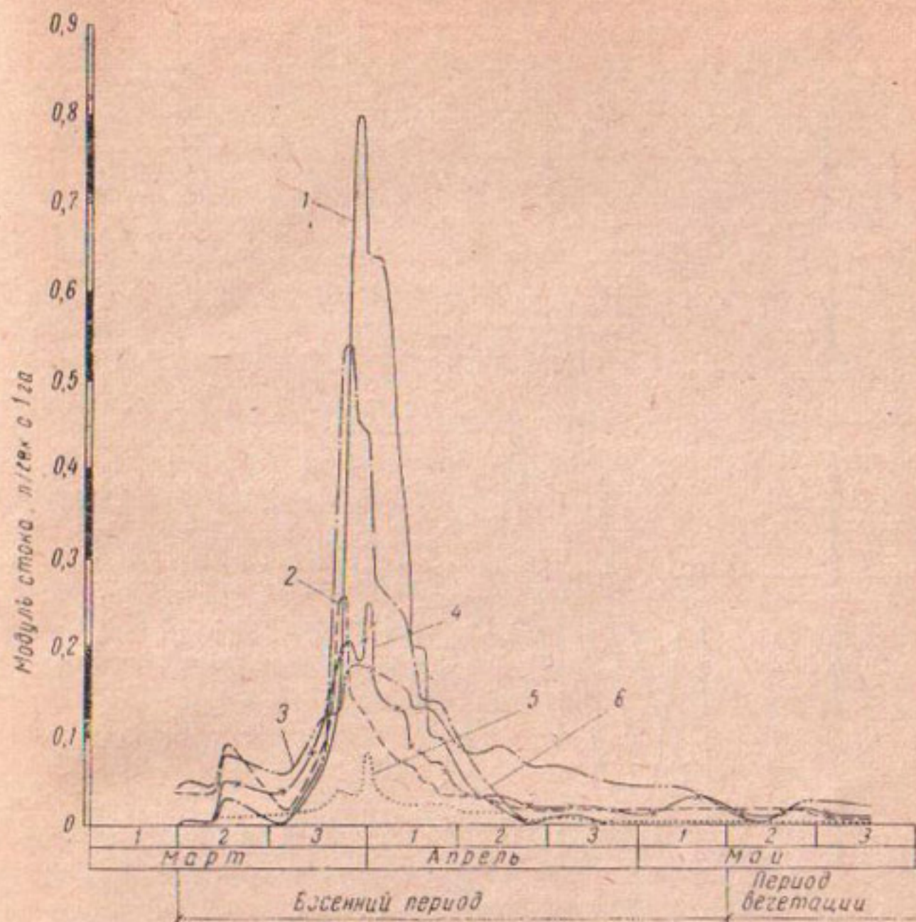
Рис. 26. Работа пластмассовых дренажей различной конструкции:
