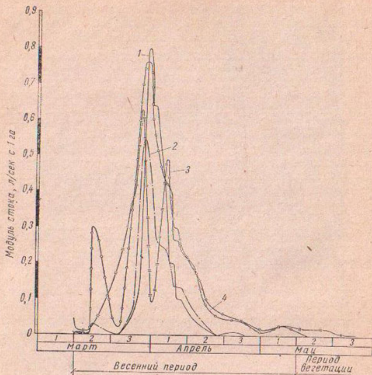
Рис. 27. Работа дрен из различных материалов:
