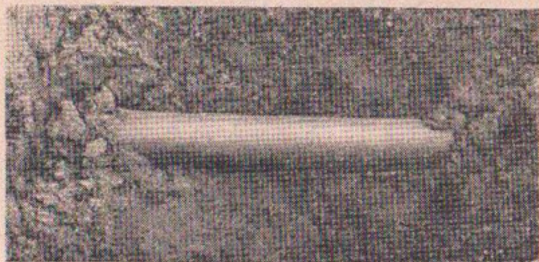
Рис. 25. Бестраншейная дрена с упругоподжатым швом внахлестку, заложенная дреноукладчиком ДПБН-1,8.
