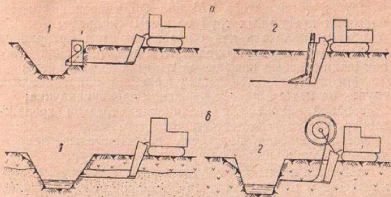
Рис. 16. Способы строительства бестраншейного дренажа из пластмасс:
