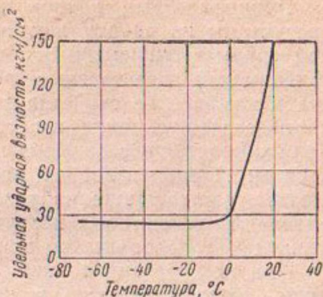
Рис. 3. Зависимость удельной ударной вязкости винипласта от температуры.
