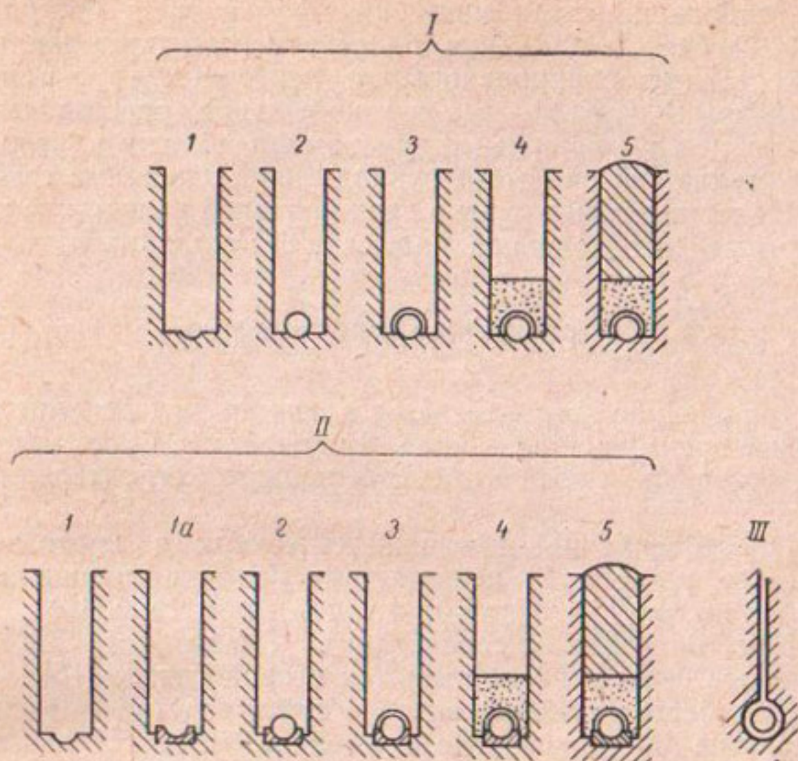
Рис. 15. Технологическая последовательность рабочих процессов при закладке дрен:
