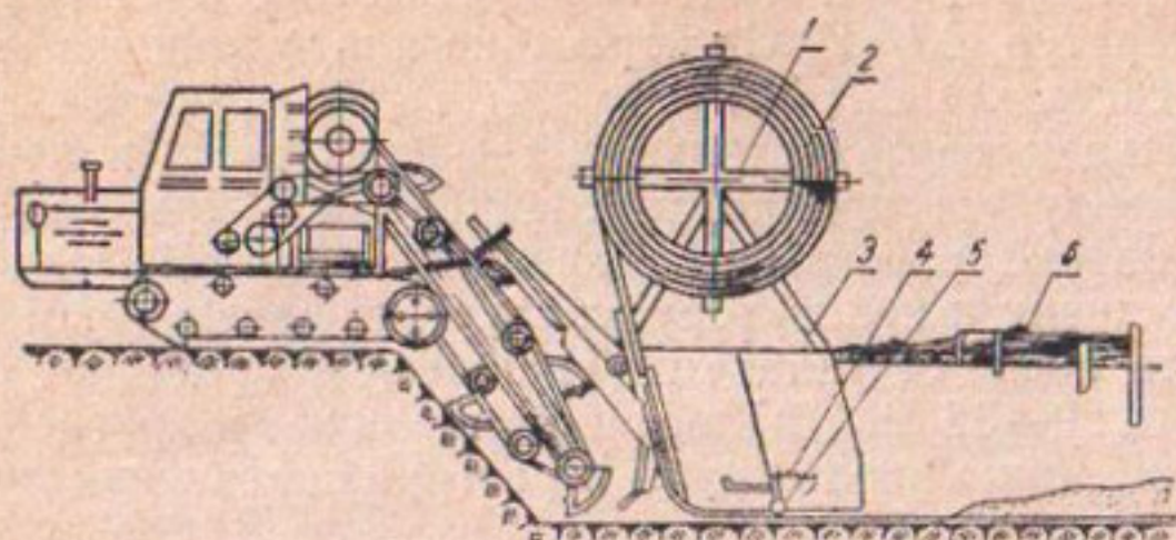
Рис. 14. Схема установки дополнительного оборудования на экскаватор ЭТН-171 при строительстве пластмассового дренажа из готовых труб:
