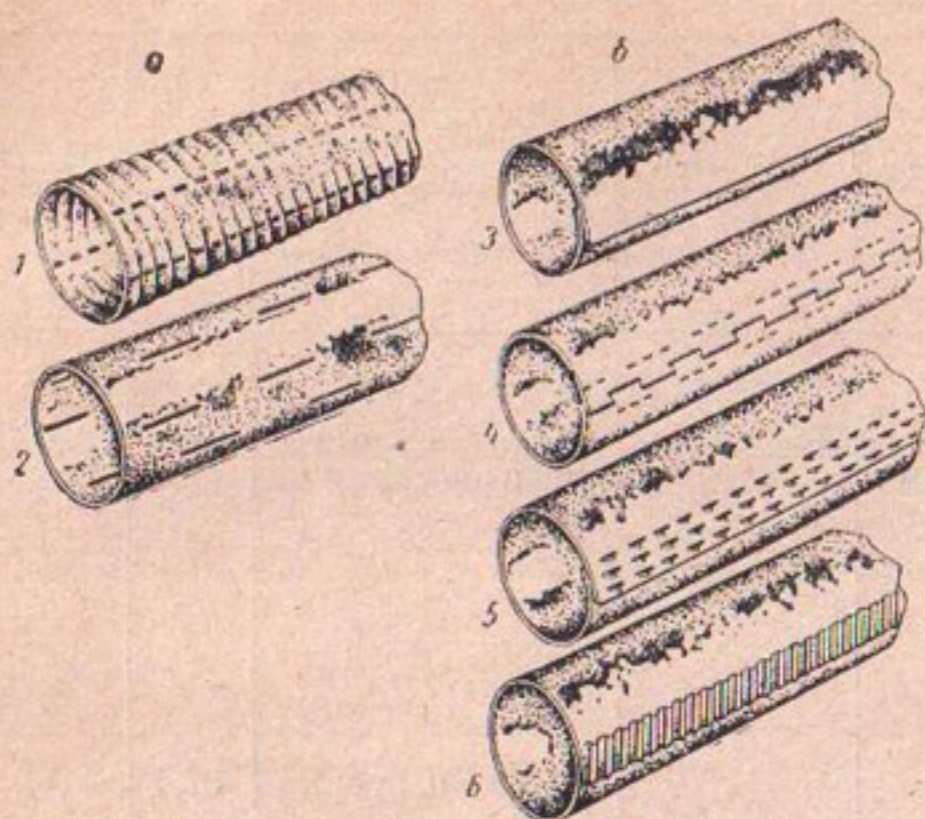
Рис. 6. Основные виды пластмассовых дренажных труб:
