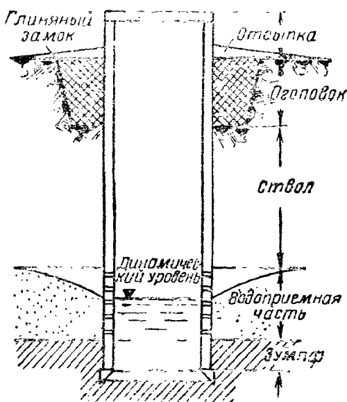
Рис. 44. Схема шахтного колодца
