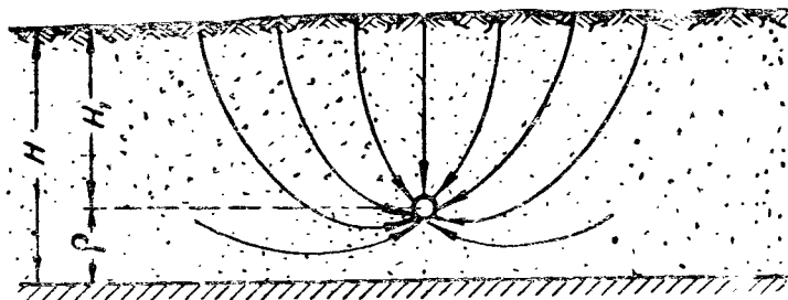
Рис. 85. Схема притока воды в водосборную галерею (по Жуковскому)
