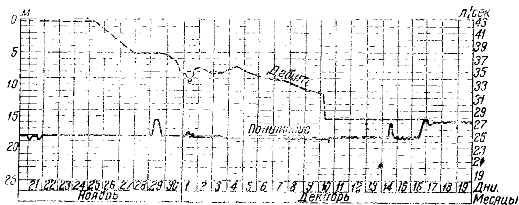
Рис. 4. График колебания уровня воды и дебита скважины при откачке
