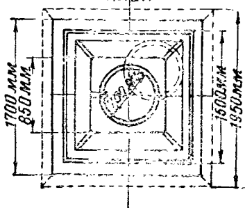
Рис. 53. Донный ящик
