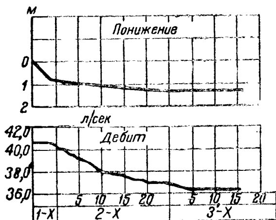
Рис. 1. График колебания уровня воды и дебита скважины при откачке
