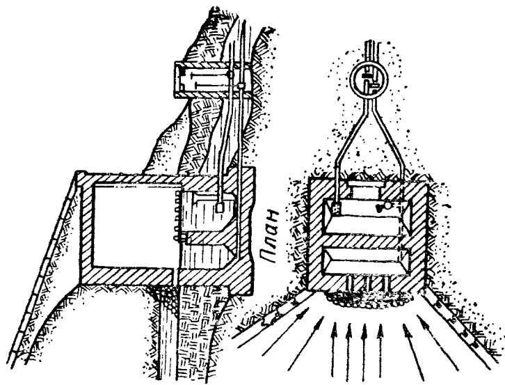
Рис. 92. Каптаж нисходящего источника с применением шпунтовых открьлков
