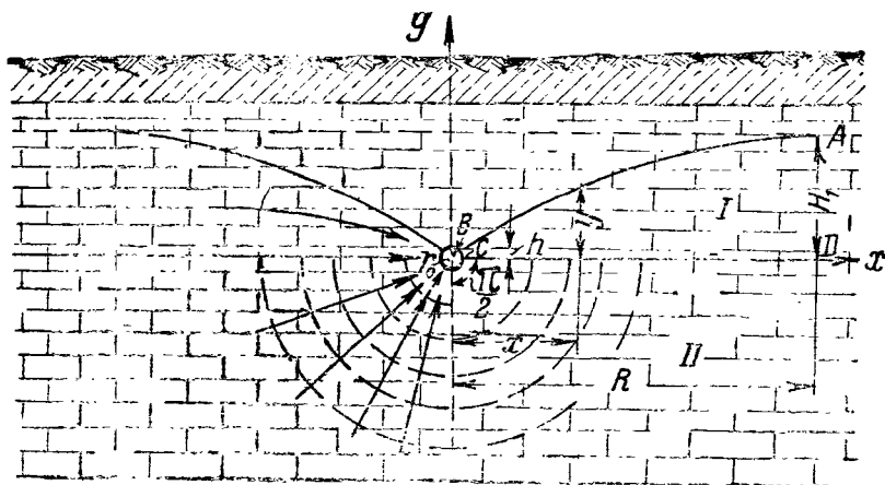
Рис. 80. Схема притока воды к дренаж в трещиноватых породах при глубоком залегании водоупора
