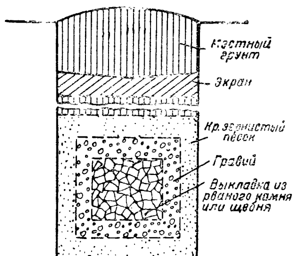
Рис. 69. Каменно-щебеночный водозабор
