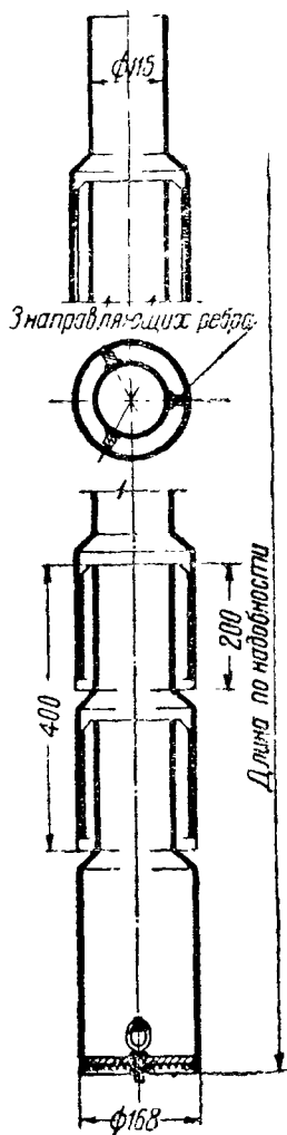
Рис. 31. Колоколь- ный фильтр Симонэ
