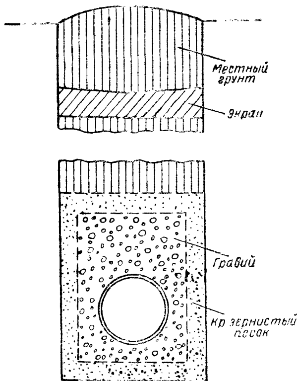
Рис. 70. Трубчатый водозабор
