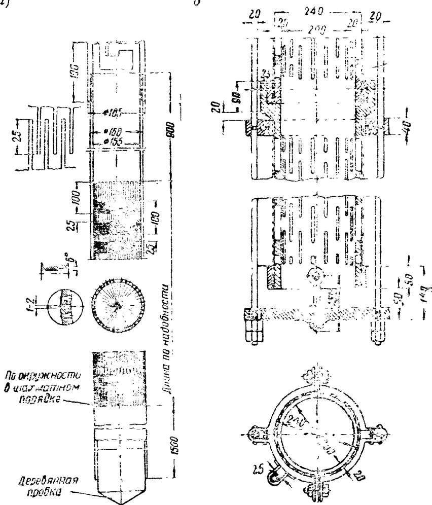
Рис. 25. Дырчатые фильтры с щел видимыми отверстиями:
