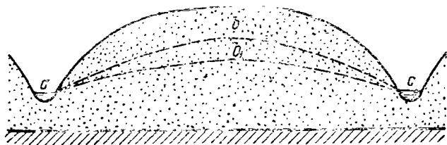
Рис. 6. Схема положения поверхности грунтовых вод для определения статических запасов
