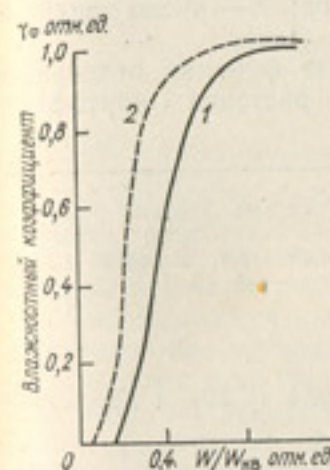
Рис. 7.3. Влажностные кривые фотосинтеза картофеля для супесчаных (1) и суглинистых (2) почв.
