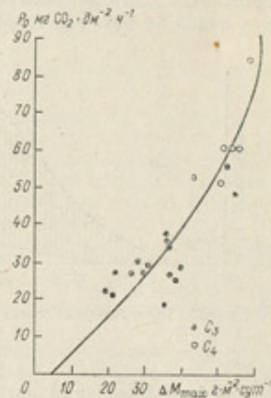
Рис. 5.2. Связь между максимальной интенсивностью фотосинтеза P_0 листьев и максимальной скоростью роста \Delta M_{\max} . По данным [278].
