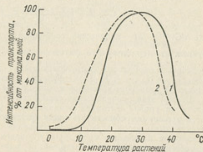
Рис. 4.3. Обобщенные кривые зависимости флоэчного транспорта от температуры у растений с высокой (1) и низкой (2) чувствительностью к охлаждению. По данным [75].
