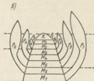
Рис. 4.2. Схема закладки листовых примордиев (а — по данным [42]) и выделение последовательных примордиев междоузлий (б — по данным [293]).
