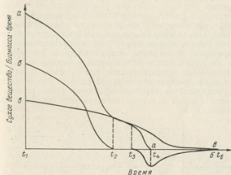
Рис. 4.4. Изменение соотношения между интенсивностью фотосинтеза, дыхания и прироста при прогрессирующей засухе.
