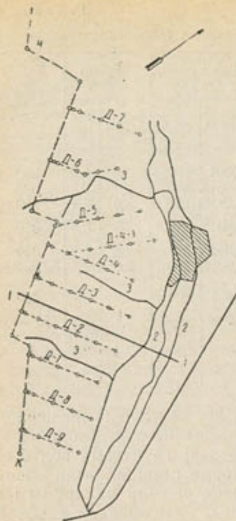
Рис. 23. Схема расположения ирригационной и дренажной сети на полях Марьинской опытной станции:
