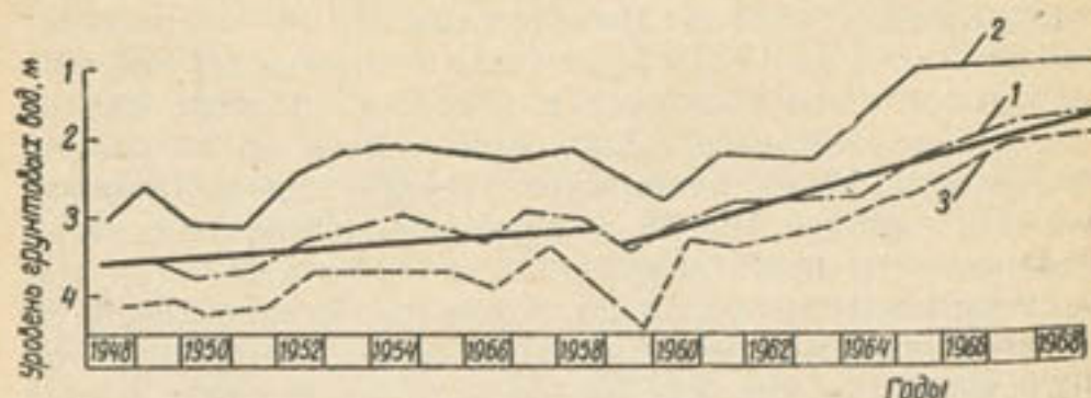
Рис. 21. Многолетняя динамика уровня грунтовых вод: 1 — среднегодовая; 2 — весна (май); 3 — осень (октябрь).
