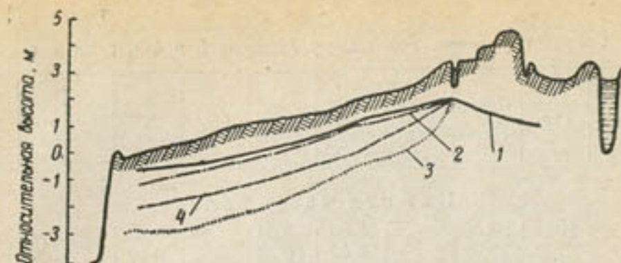
Рис. 24. Изменение уровня грунтовых вод под влиянием дренажа. Профиль по створу I—I:
