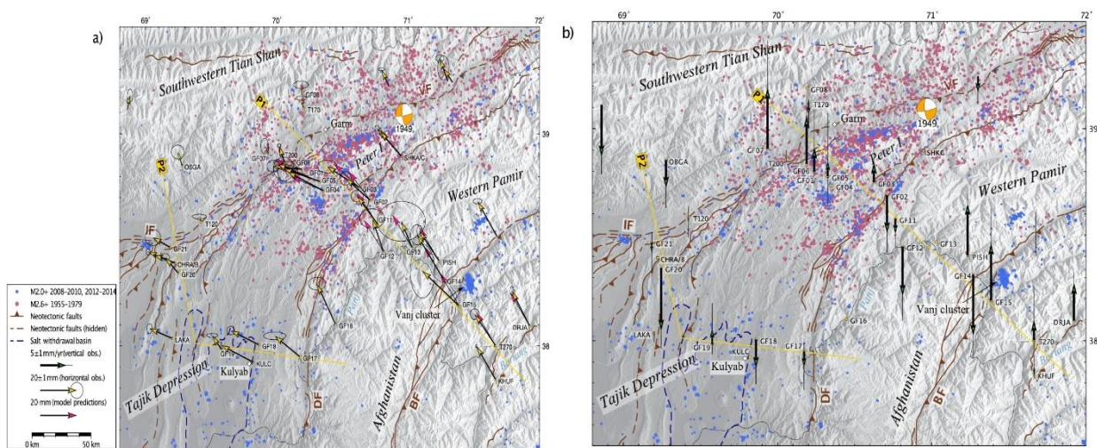
Рис.2. Горизонтальная и (б) вертикальная скорости GNSS, измеренные в период с 2013 по 2015 год с 20 неопределённостями в Евразийской системе отсч`та (Аль-Тамими и др., 2017). Розовые стрелки (а) — смоделированные показатели. Обратите внимание на разные шкалы ставок в (а) и (б). Жёлтыми линиями отмечены профили P1 и P2, коровая сейсмичность Гамбургер и др. (1992) красным цветом, а Куфнер и др. (2018) синим цветом [4].
